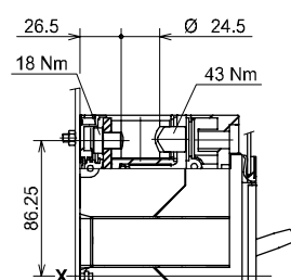
Front for copper/aluminum cables - FC CuAl 300 mm 2
