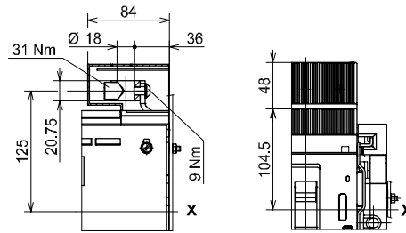
Front for copper/aluminum cables - FC CuAl
