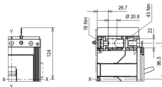
Front for copper/aluminum cables - FC CuAl 2x240 mm 2
