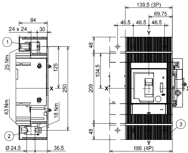
Front for copper cables - FC Cu or for copper/aluminum cables - FC CuAl 400 A
