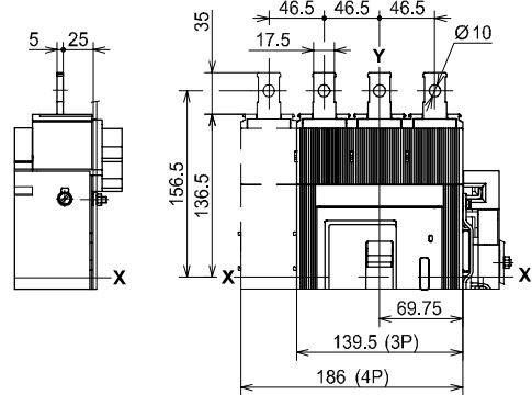
Front for copper cables - FC Cu or for copper/aluminum cables - FC CuAl 400 A
