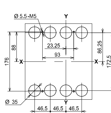
4 POLES
