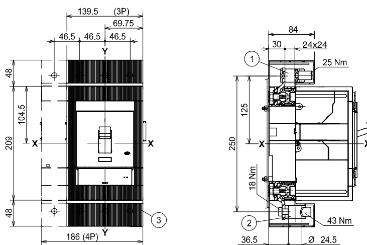
Front for copper cables - FC Cu or for copper/aluminum cables - FC CuAl
