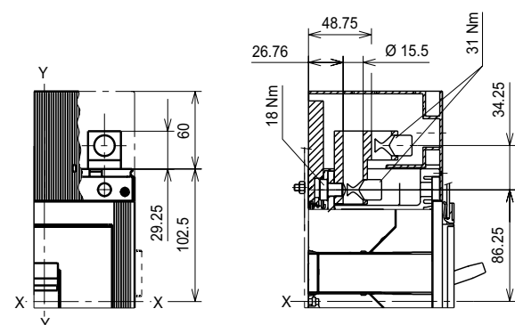
Front for copper/aluminum cables - FC CuAl 300 mm 2
