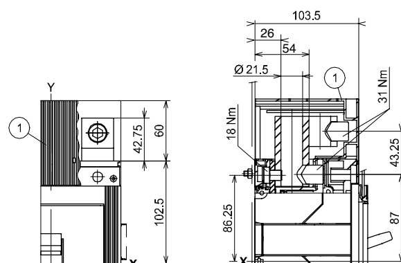
Front for copper/aluminum cables - FC CuAl 2x240 mm 2
