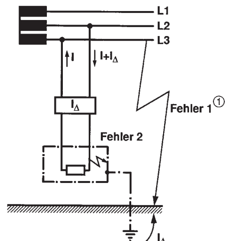
IT-System Der Fehlerstrom-Schuttschalter löst aus, wenn ein doppelter Fehler vorhanden ist z.B. wie dargestellt Fehler 1 und Fehler 2 ① führt nur zur Anzeige durch den Isolationwächter
