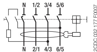
F 204 A Neutraleiter-Anschluss links
