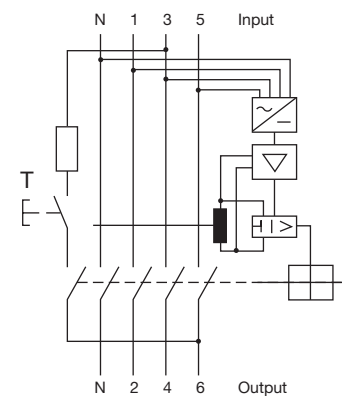
F 204 A (125 A) F 204 B, F 204 B+ (100A, 125A) Neutraleiter-Anschluss links
