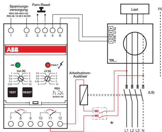
Anschluss eines RD3 mit Arbeitsstrom-Auslöser
