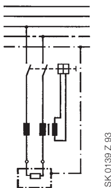
Fehlerstrom-Schutzschalter (FI) bis 125 A VDE 0664-10, DIN EN 61008-1/IEC 61008-1
