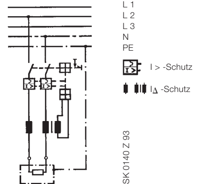
Fehlerstrom-Schutzschalter mit Überstromauslöser (FI/LS) VDE 0664-20, DIN EN 61009-1/IEC 61009-1
