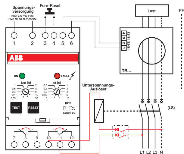
Anschluss eines RD3 mit Unterspannungs-Auslöser
