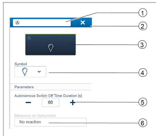
Fig. 64: Actuator settings
