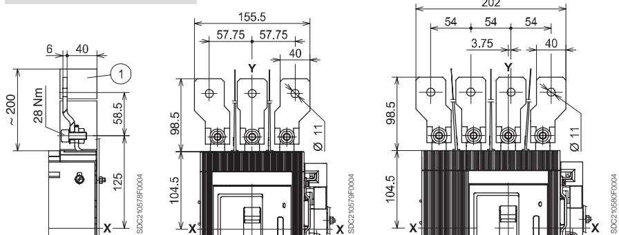
加长扩展前接线端子 - ES 630 A
