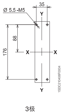
支撑钢板钻孔图
