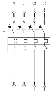
带热磁脱扣器的3/4极断路器
