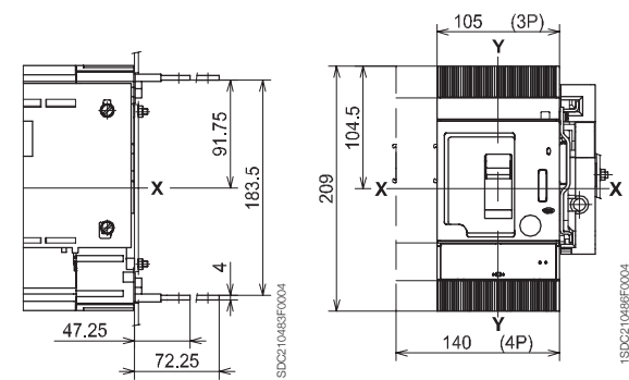
后水平接线端子 - HR
