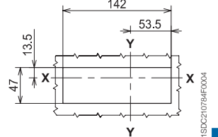
4 极 (不带法兰和断路器扩展)
