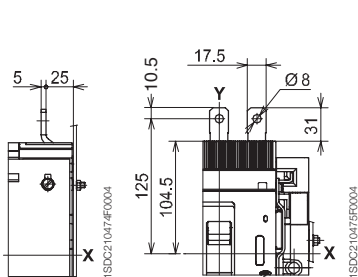
加长前接线端子 - EF
