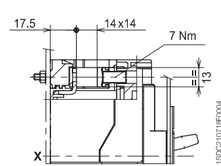
铜电缆前接线端子 - FC Cu
