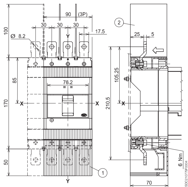
加长前接线端子 - EF
