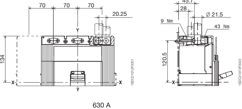
铜 / 铝电缆前接线端子 - FC CuAl 2x240 mm 2
