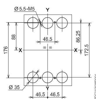
3极
