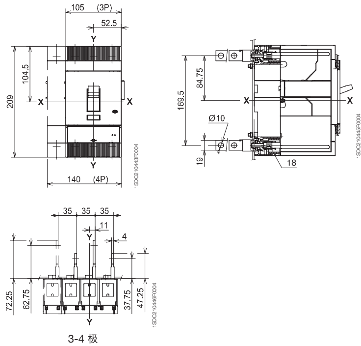
后垂直接线端子 - VR
