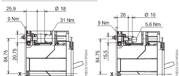
铜 / 铝电缆前接线端子 - FC CuAl
