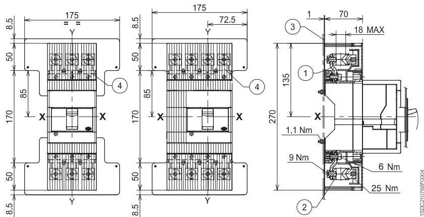
铜 / 铝电缆前接线端子 - FC CuAl 185mm 2
