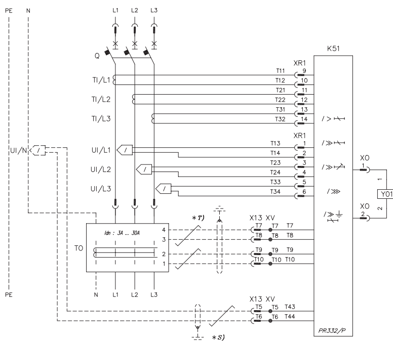
帶PR332/P电子脱扣器和剩余电流保护的3极断路器 ( U \leq 690V )
