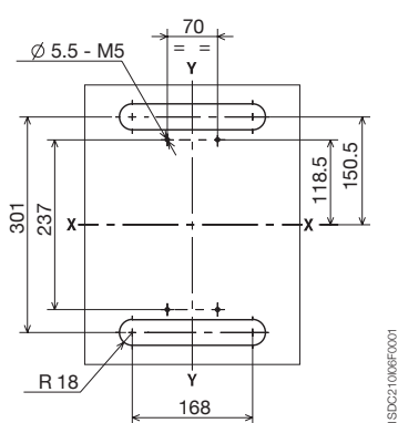
630 A (3极)
