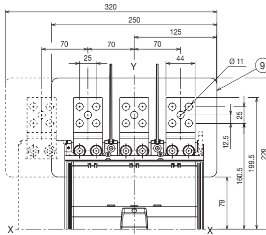
加长前接线 - EF
