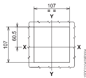
不带法兰
