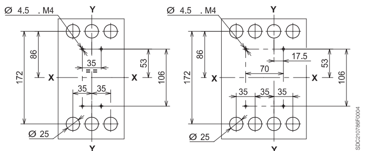
3 极
