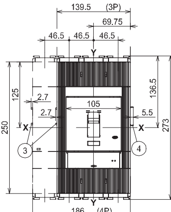
630 A
