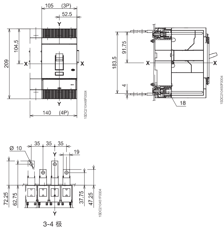
后水平接线端子 - HR
