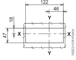
4 极 (不带法兰和断路器扩展)
