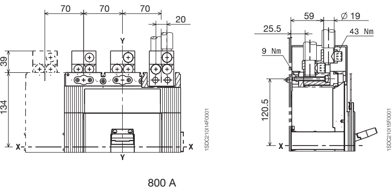
铜 / 铝电缆前接线端子 - FC CuAl 3x185 mm 2
