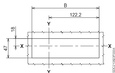
小室门钻孔图
