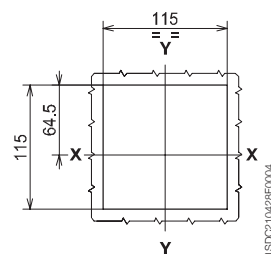
带法兰
