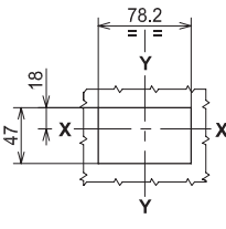
3-4 极 (不带法兰和断路器与小室门平齐)
