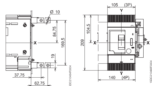
后垂直线端子 - VR
