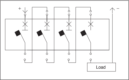
图D：四极串联为单极
