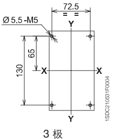
前接线端子 - F 400 A
