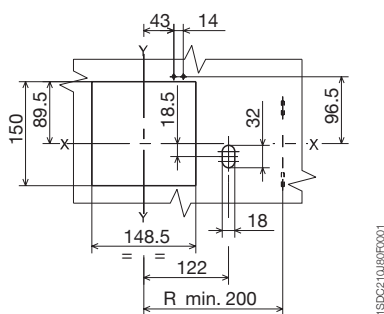
小室门钻孔图
