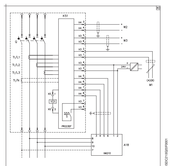
带VM210电压测量装置的PR223EF电子脱扣器
