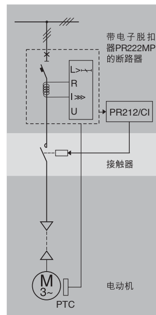
综合保护
