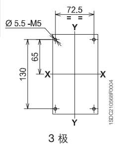
3 极
