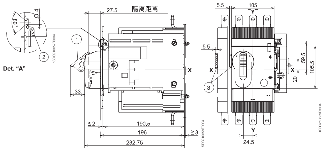
断路器旋转手柄操作机构
