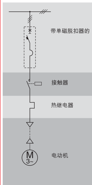
短路保护
