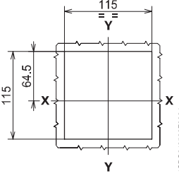
带法兰
