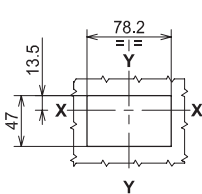
3-4 极 (不带法兰和断路器与小室门平齐)
