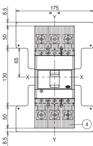
铜 / 铝电缆前接线端子 - FC CUAL 185mm 2
