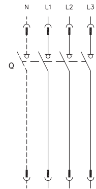
3/4极隔离开关
