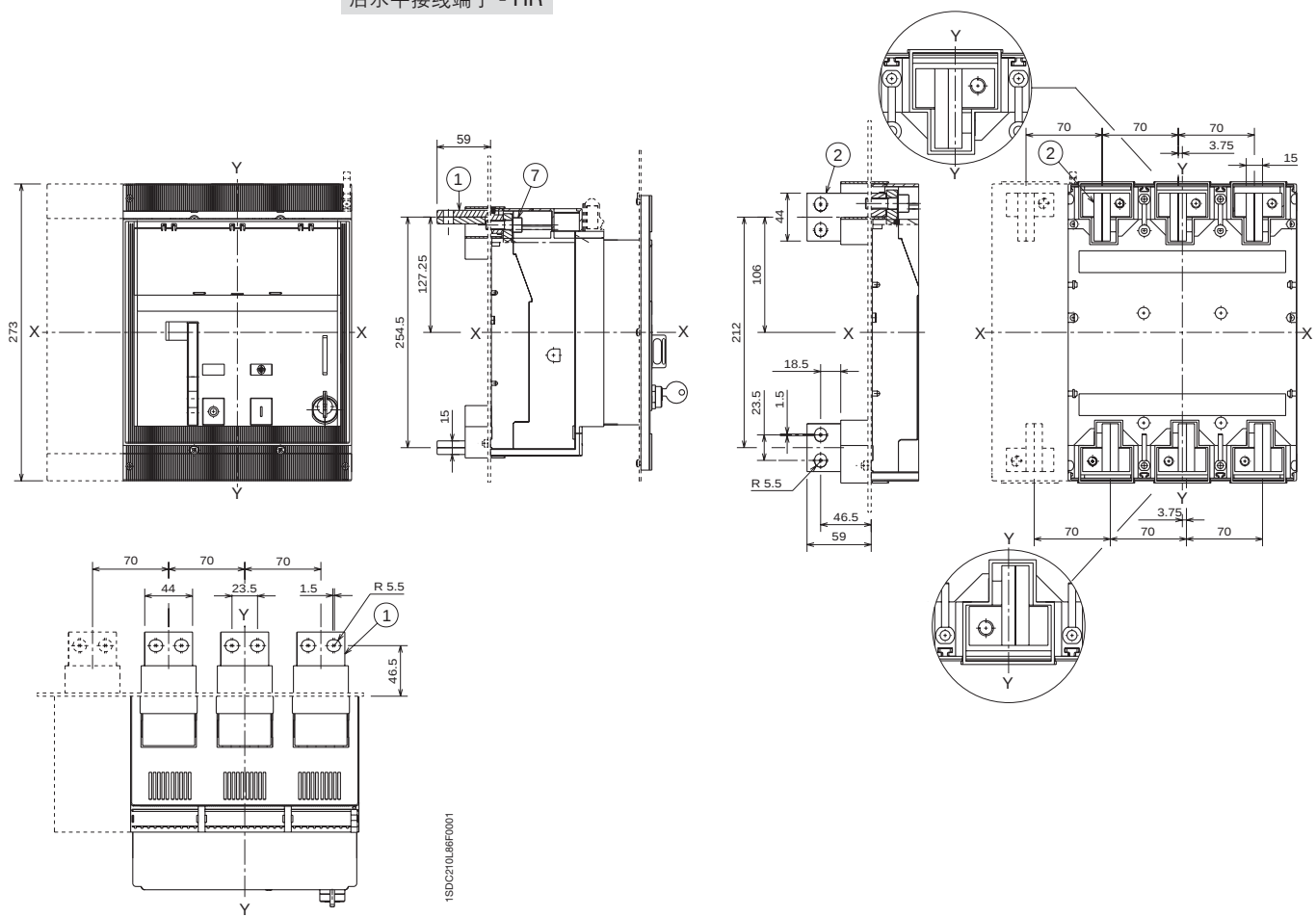
后水平接线端子 - HR
