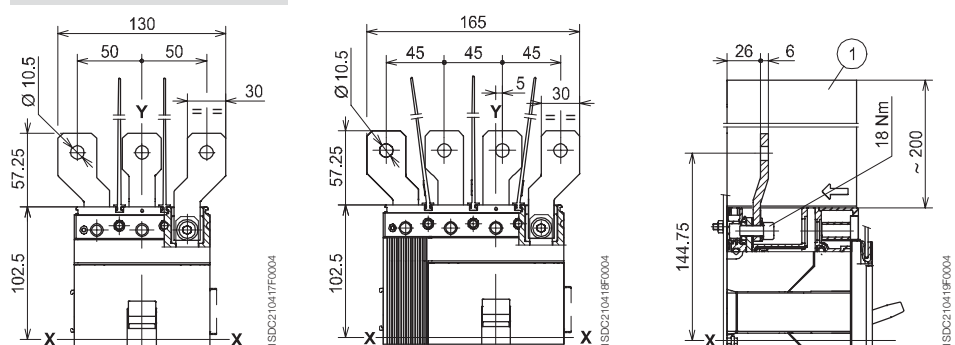
加长扩展型前接线端子 - ES
