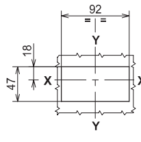
3 极 (不带法兰和断路器扩展)
