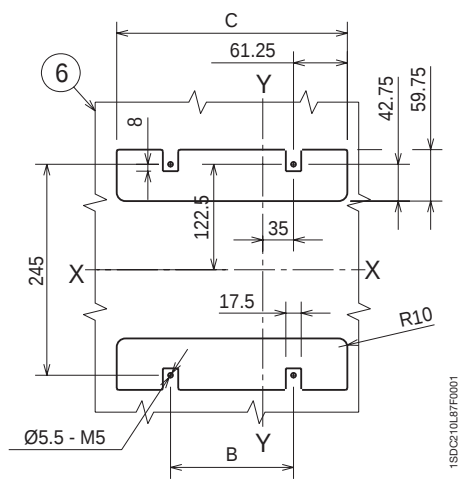
支撑钢板钻孔图
