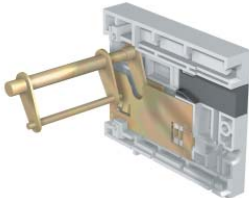
插入式固定部件改成 抽出式固定部分的转换套件
