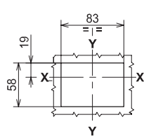
3-4 极 (带法兰和断路器与小室门平齐)
