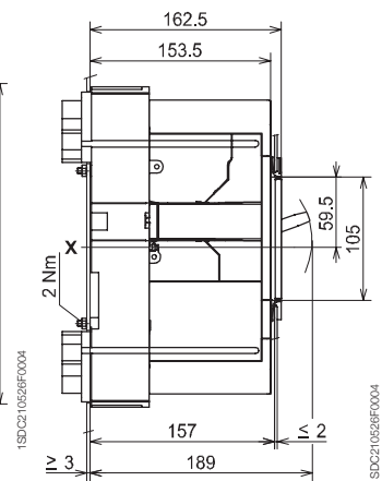
630 A
