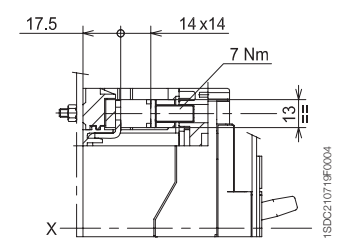
铜 / 铝电缆前接线端子 - FC CuAl 95mm 2
