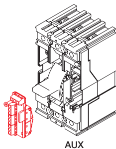
AUX
