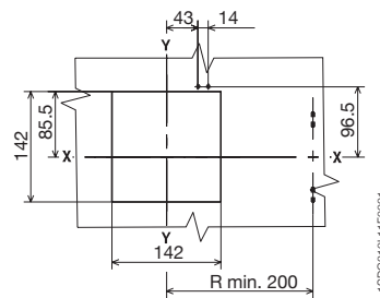
不带法兰
