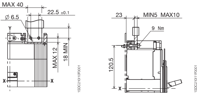
前接线端子 - F
