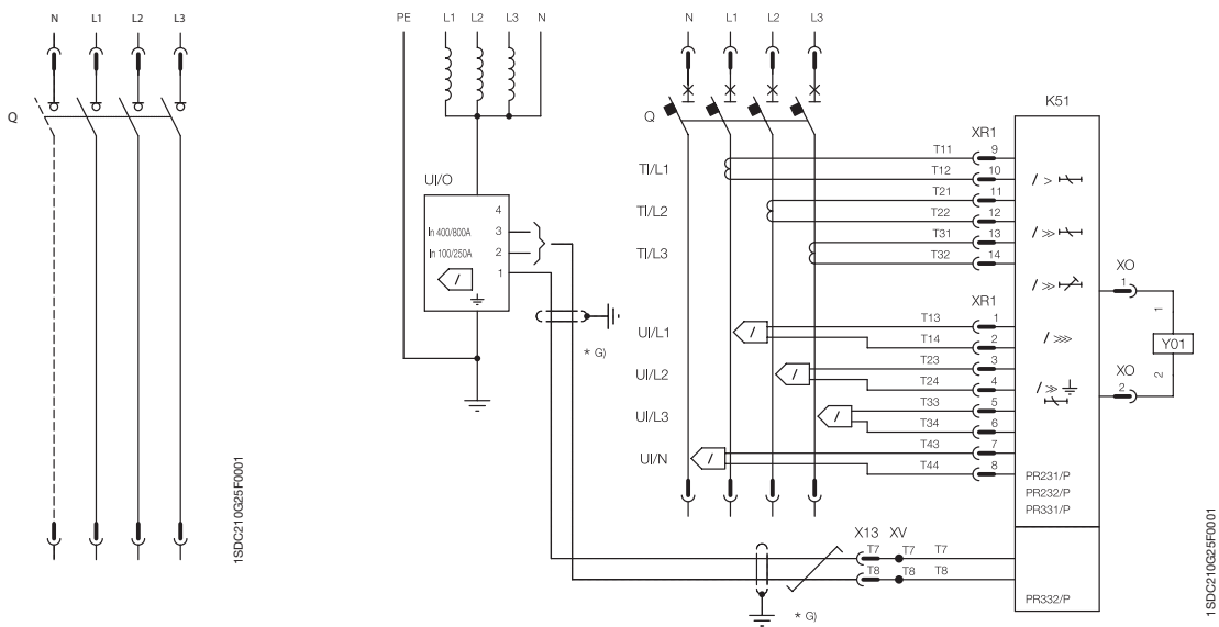
3/4隔离开关
