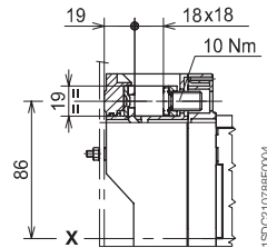
铜 / 铝电缆前接线端子 - FC CuAl 240mm 2
