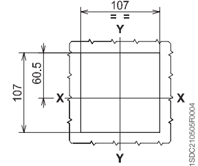
3-4 极 (不带法兰)
