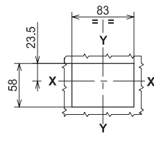
3-4 极 (带法兰和断路器与小室门平齐)
