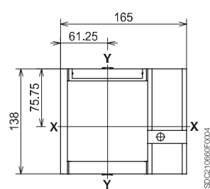
小室门法兰
