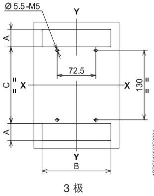
后接线端子 - F 400 A - 630 A
