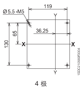
4 极
