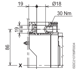
铜 / 铝电缆前接线端子 - FC CuAl 185mm 2
