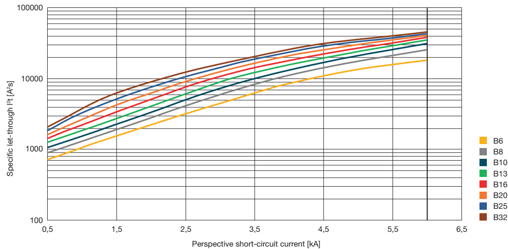
DS203NC, характеристика В 400 В удельная пропускаемая энергия
