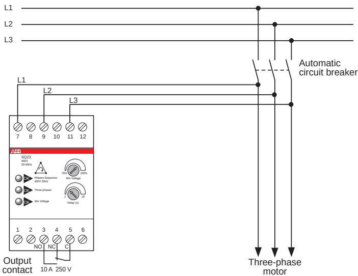
SQZ3 Реле последовательности фаз
