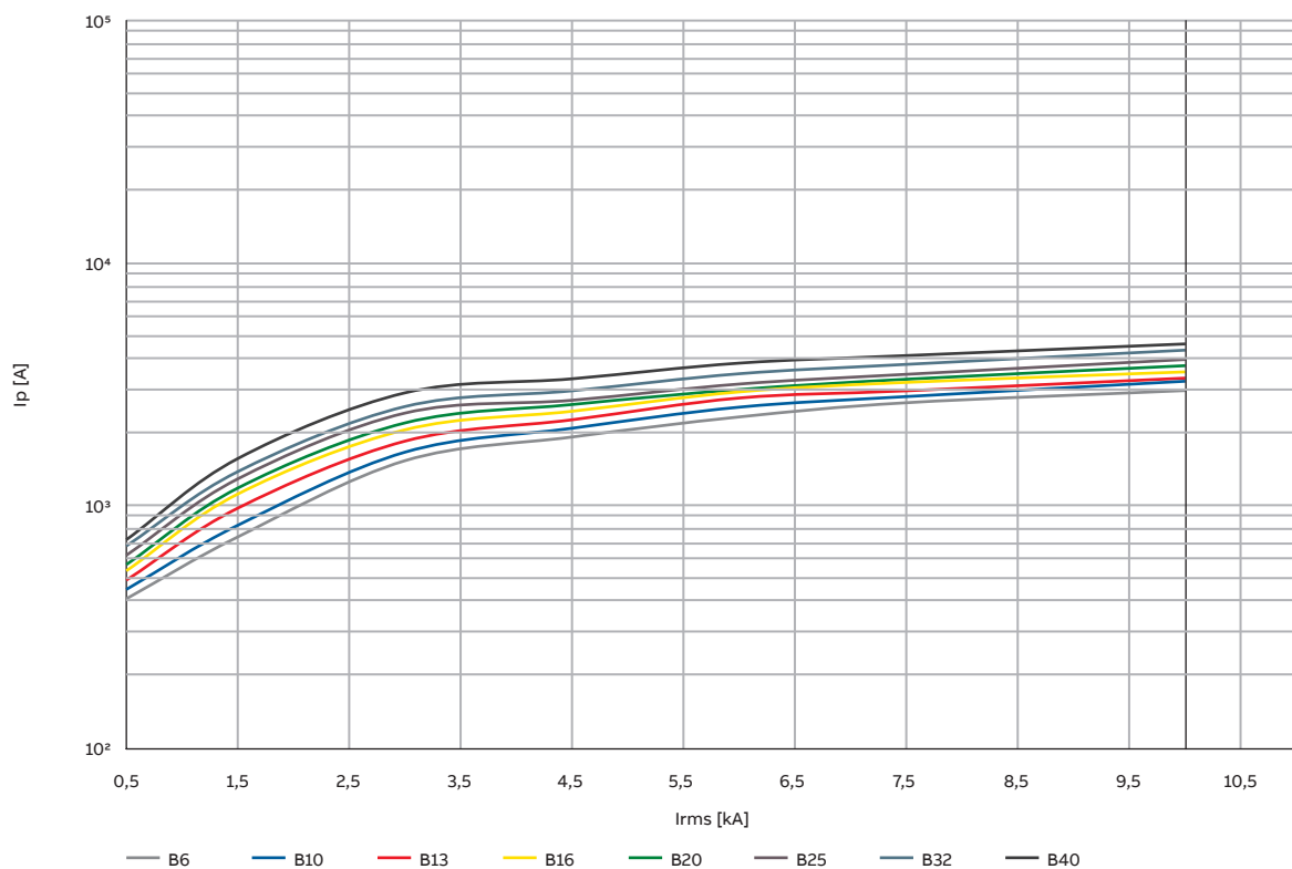
I_{peak} для DS201M - Характеристика В
