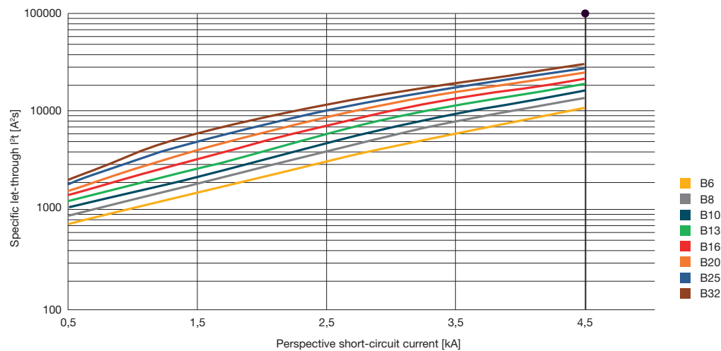
DS203NC L, характеристика В 400 В удельная пропускаемая энергия
