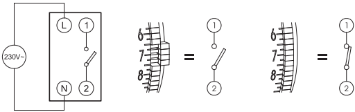
Схема подключения
