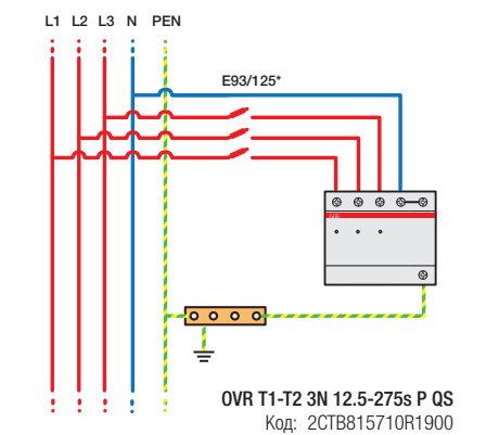
Конфигурация 3 I_p \leq 7\text{ kA}
