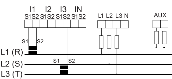
3-фазная 3-проводная с двумя ТТ
