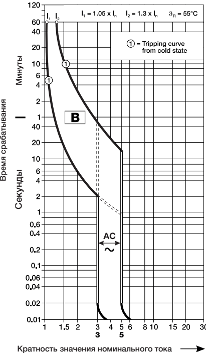
Характеристика В IEC-EN60947-2
