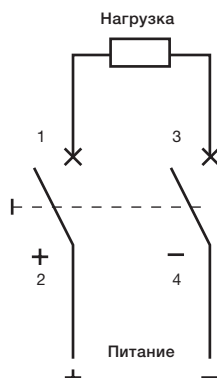
Схема подключения, 2-полюсные (макс. 440В пост.т.) S402M-UCZ
