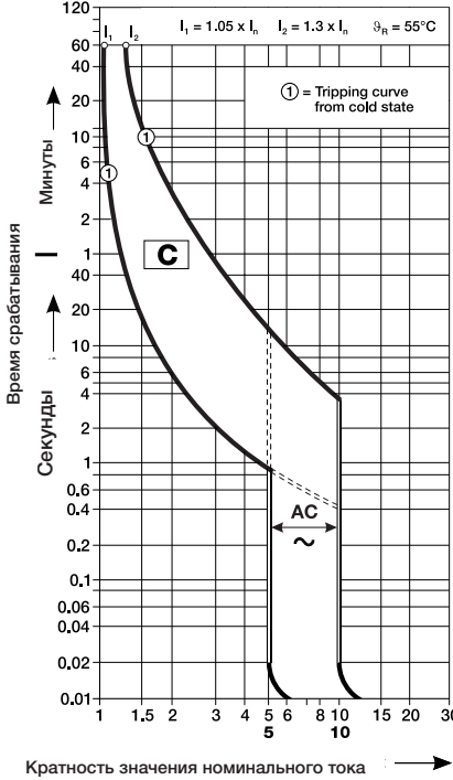
Характеристика С IEC-EN60947-2
