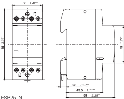
ESB25..N Габаритные размеры, мм, дюйм
