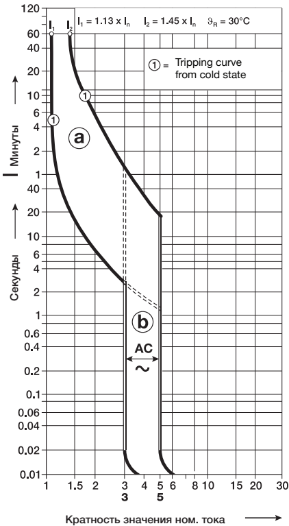
Характеристика В IEC/EN 61009-1
