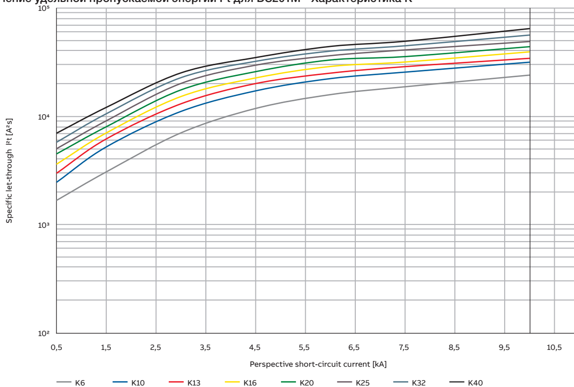
Значение удельной пропускаемой энергии I^2t для DS201M - Характеристика K
