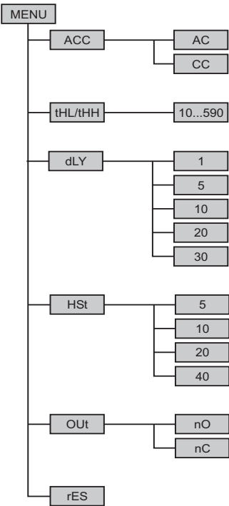
Вид меню вольтметров
