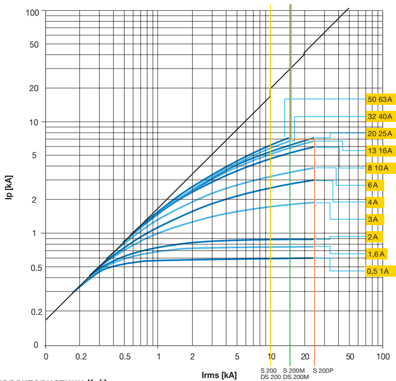
S 200-S 200 M-S 200 P, характеристики К-D
