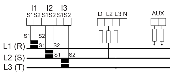
3-фазная 3-проводная с тремя ТТ
