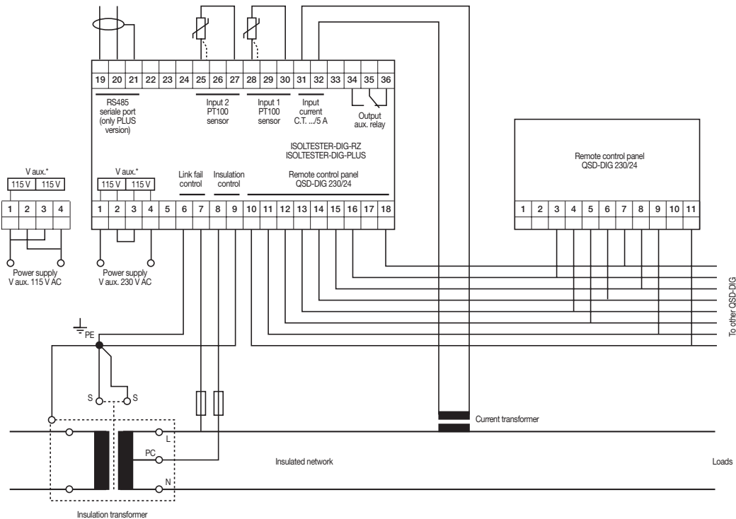
Схема подключения ISOLTESTER-DIG, QSD-DIG и SELVTESTER-24 для трансформатора с центральной точкой (PC)
