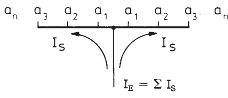
Подача питания в центре шины
