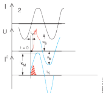
Автоматический выключатель с ограничением тока
