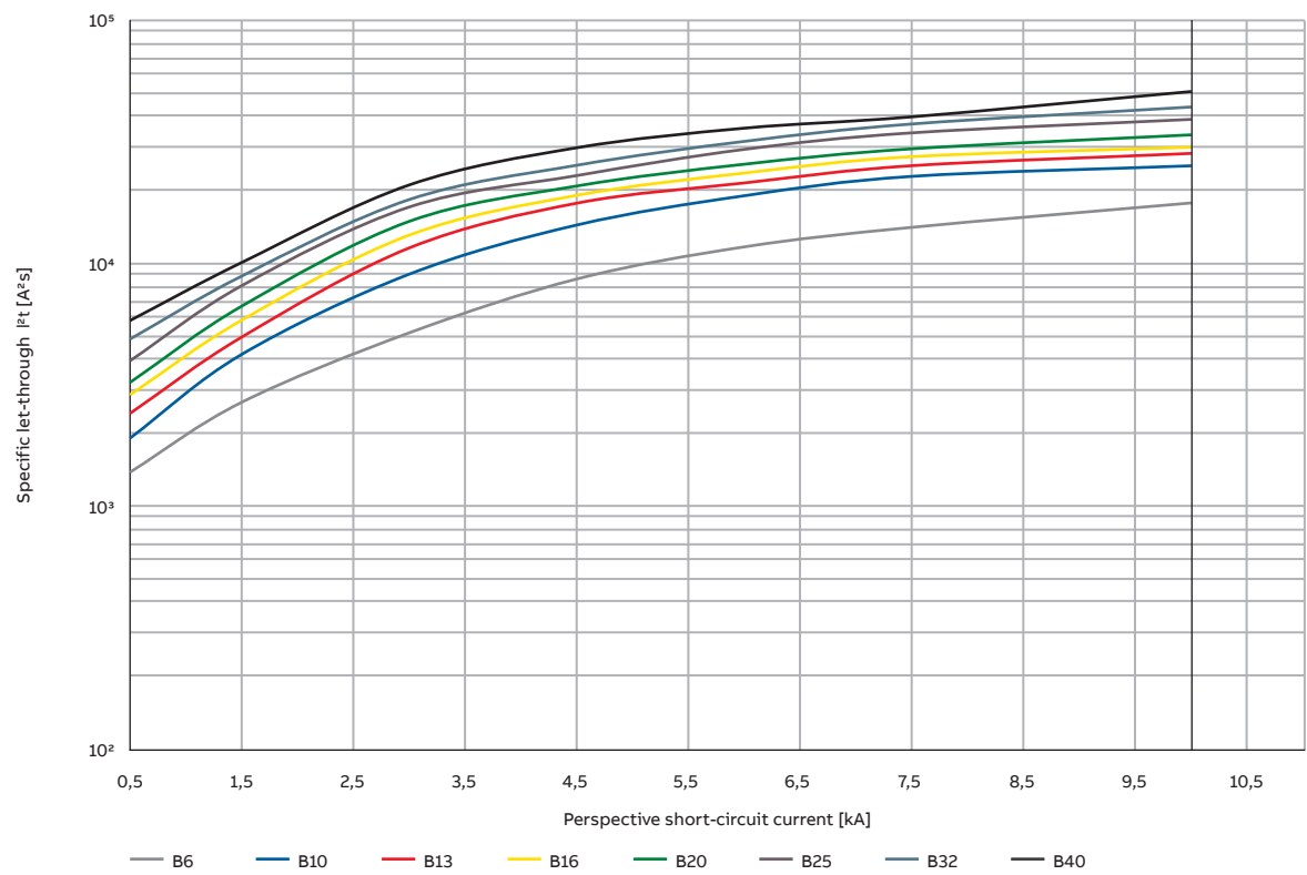
Значение удельной пропускаемой энергии I^2t для DS201M - Характеристика В
