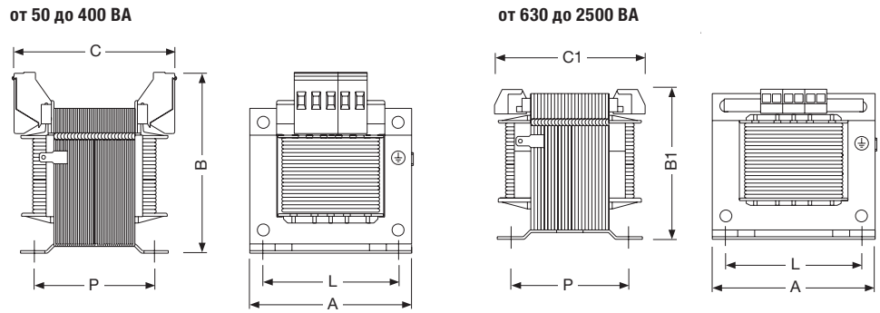
ТМ-С трансформаторы для цепей управления
