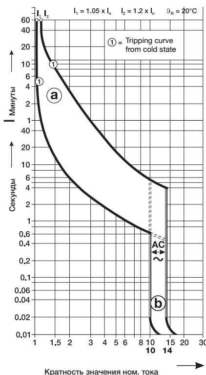
Характеристика К IEC-EN60947-2
