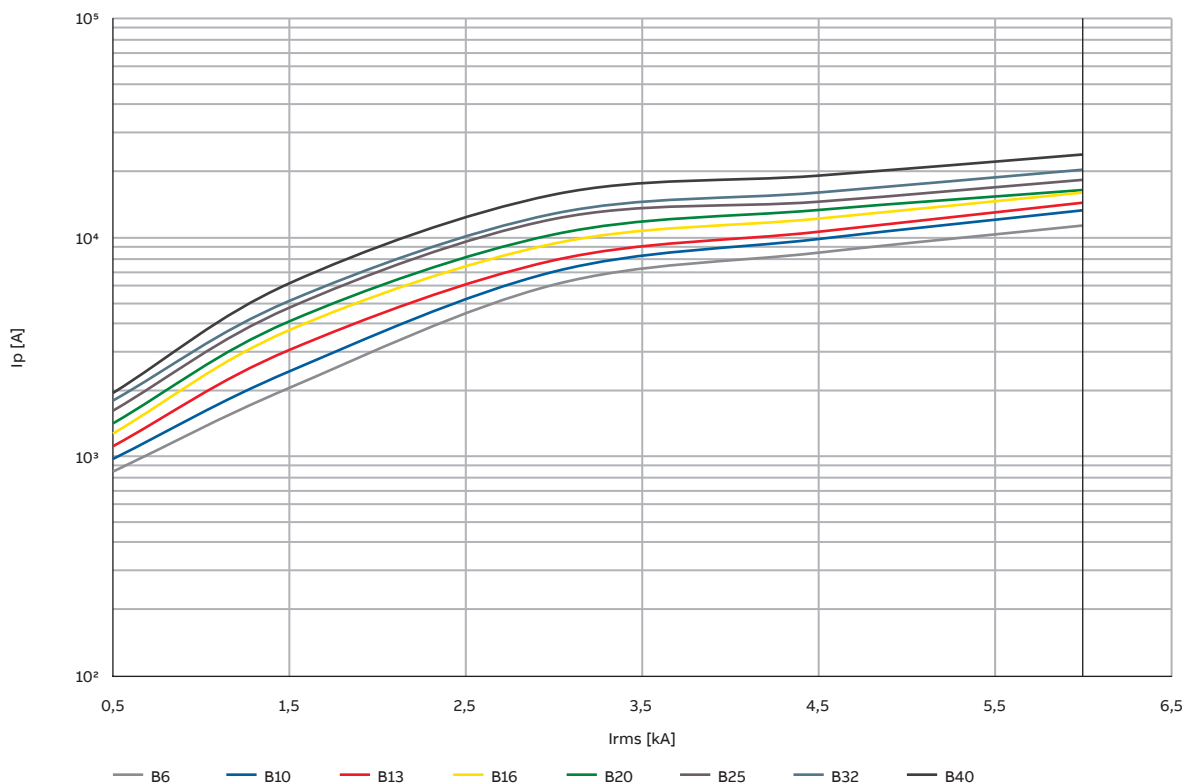
I_{peak} для DS201 - характеристика B
