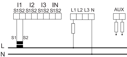
1-фазная 2-проводная с одним ТТ
