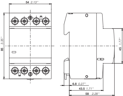
ESB40..N Габаритные размеры, мм, дюйм
