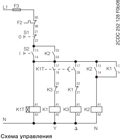
Схема управления
