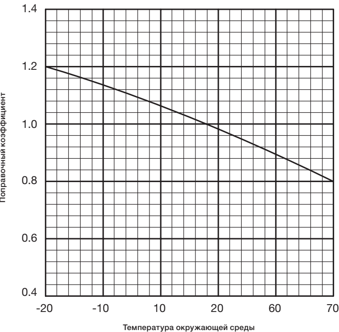
Дерейтинг в зависимости от температуры окружающей среды
