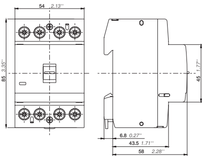
EN40..N Габаритные размеры, мм, дюйм
