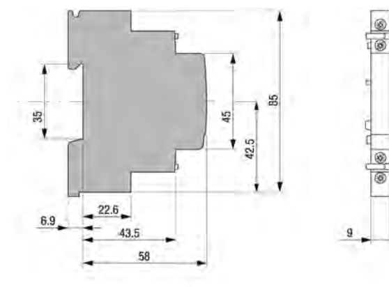
E299-11 вспомогательный контакт
