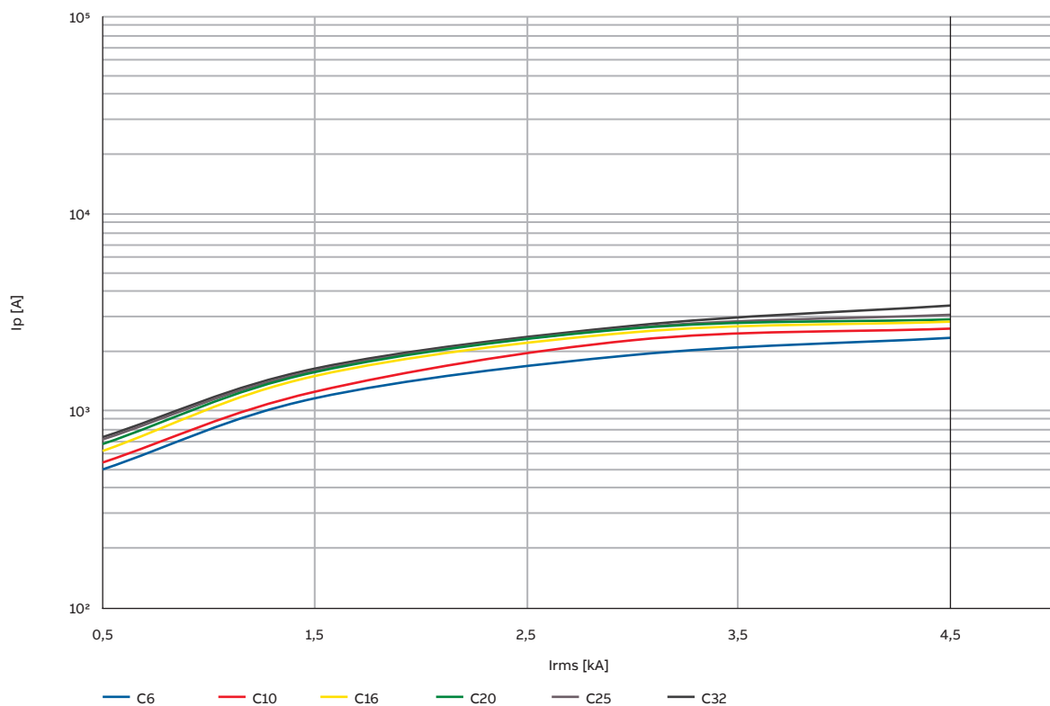
I_{peak} для DS201L - характеристика C
