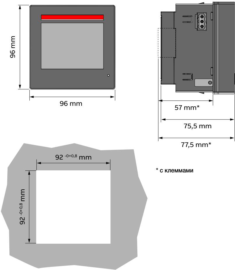
M4M - анализаторы сети
