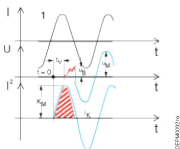
Автоматический выключатель без ограничения тока
