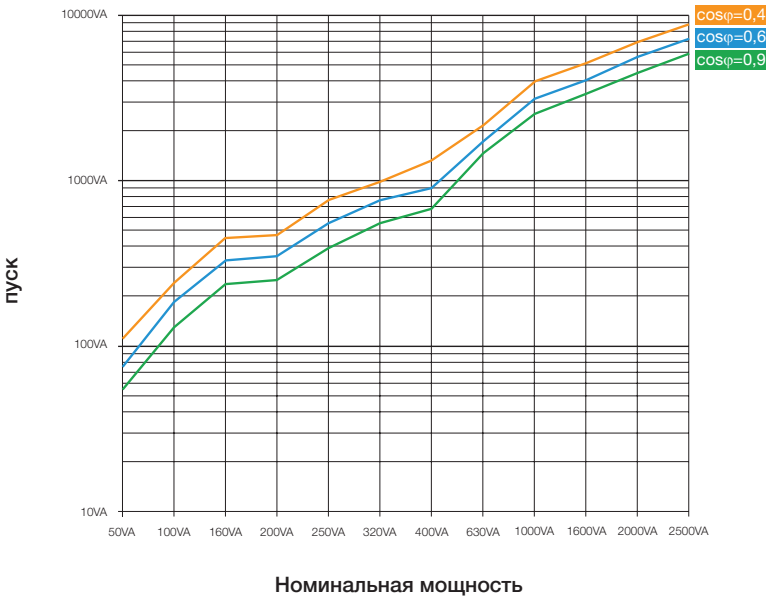
Кривая пусковой мощности
