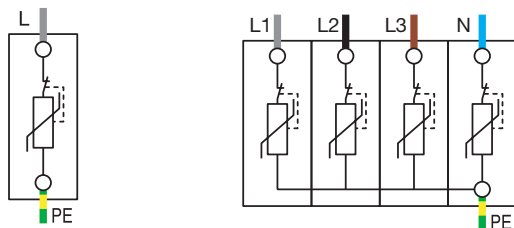
OVR T2 40-275 P QS OVR T2-T3 20-275 P QS
