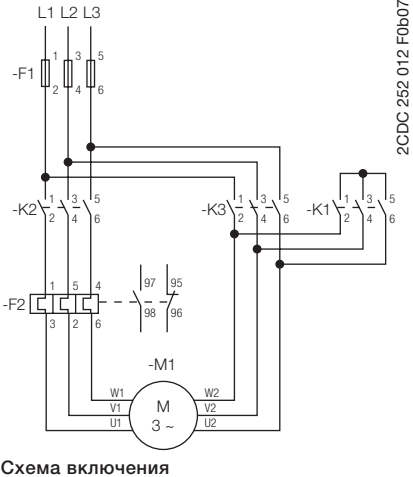
Схема включения
