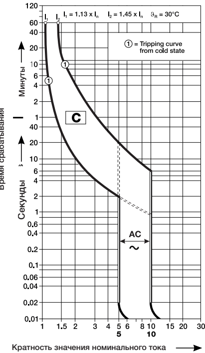
Характеристика С IEC-EN60898-1
