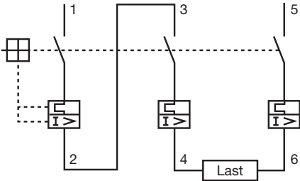
Схема подключения пускателя электродвигателя
