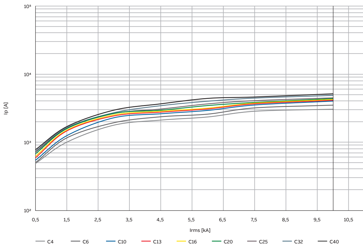
I_{peak} для DS201M -Характеристика С
