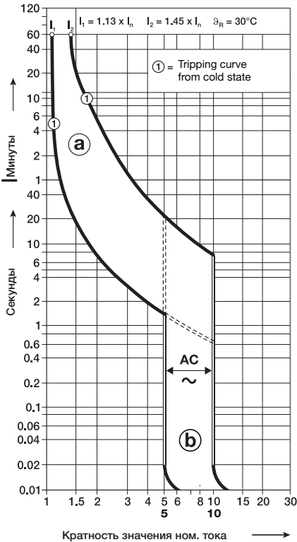
Характеристика С IEC/EN 61009-1
