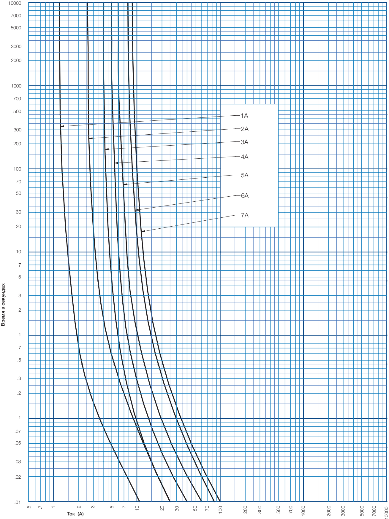
Время-токовые характеристики
