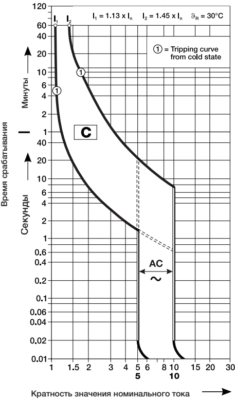
Характеристика С
