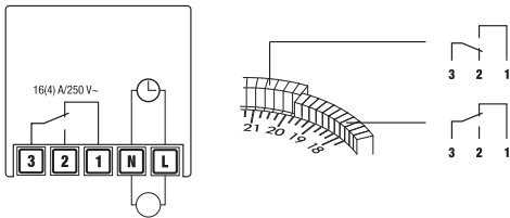
Схема подключения
