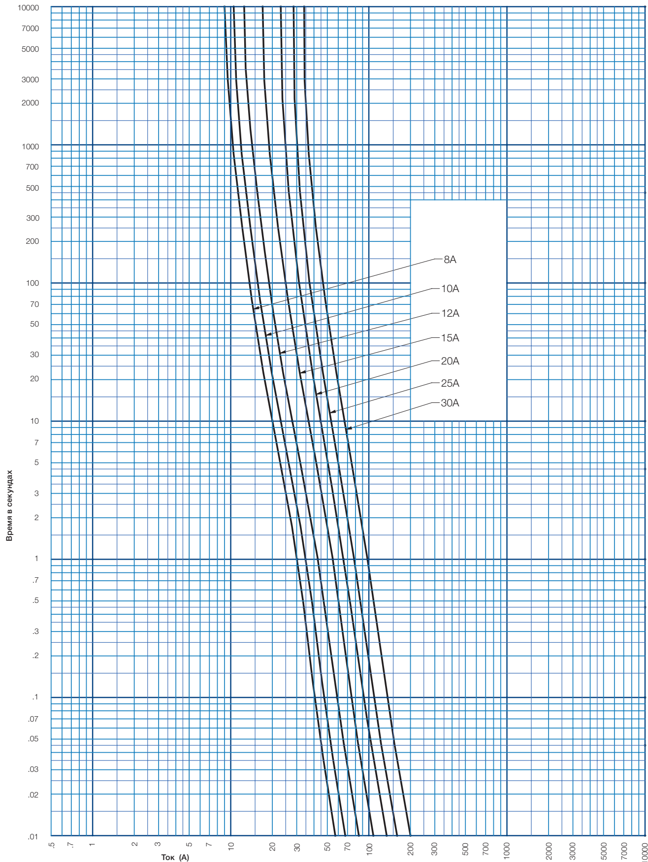
Время-токовые характеристики
