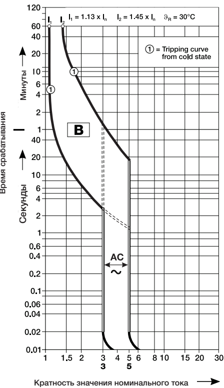
Характеристика В
