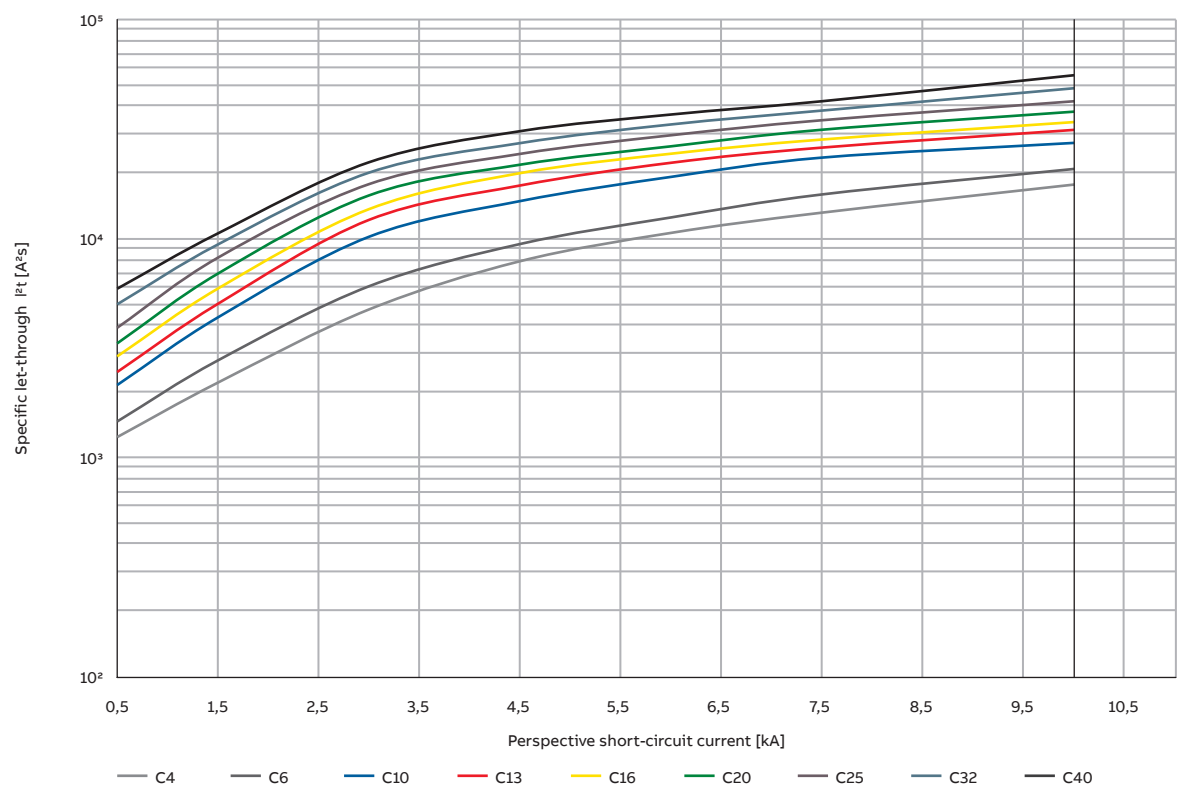
Значение удельной пропускаемой энергии I^2t для DS201M - Характеристика С
