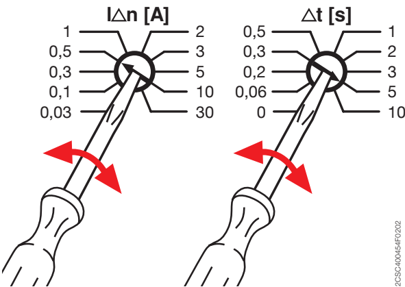
Регулировка отключающего дифференциального тока ( I_{\Delta n} [A]) и времени задержки срабатывания ( \Delta t [c]).
