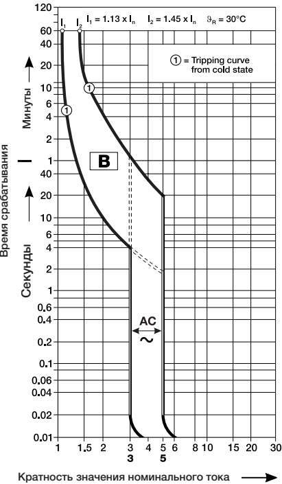
Характеристика В IEC-EN60898-1
