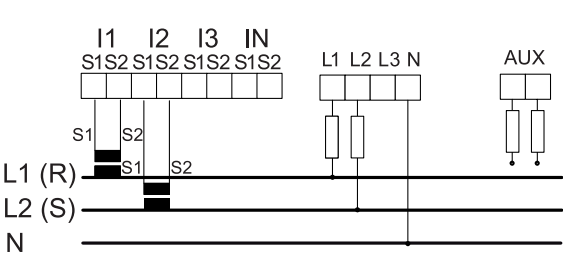
2-фазная 3-проводная с двумя ТТ
