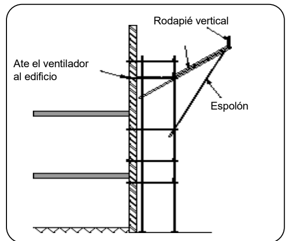
Fig. 3 – Suministro del ventilador de protección
