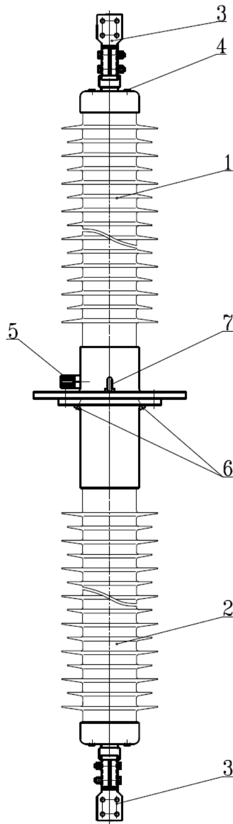
Рис. 1 Конструкция ввода
