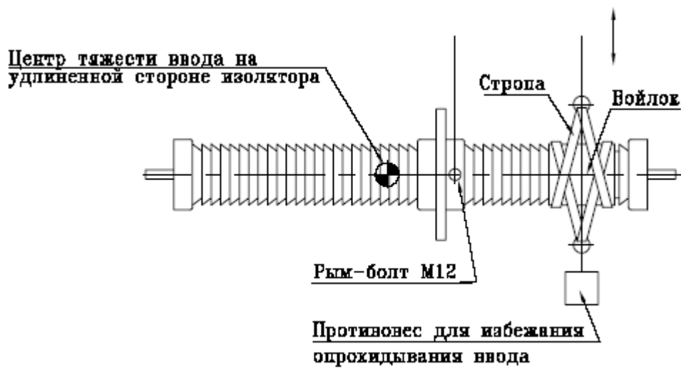
Рис.3 Монтаж ввода
