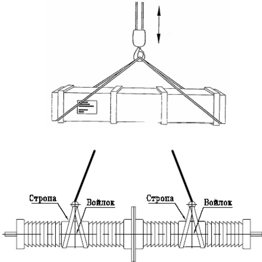
Рис.2 Выемка ввода из упаковочного ящика
