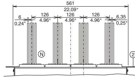
E3 4 poles 2500 A
