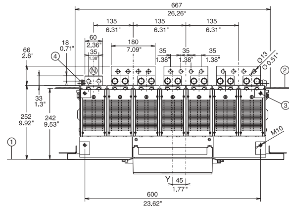
E4 4 poles
