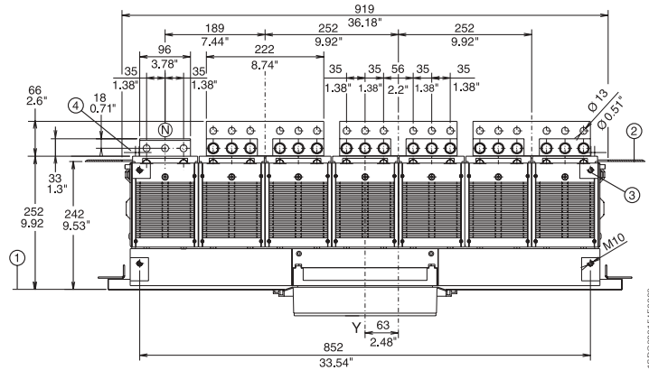
E6 4 poles
