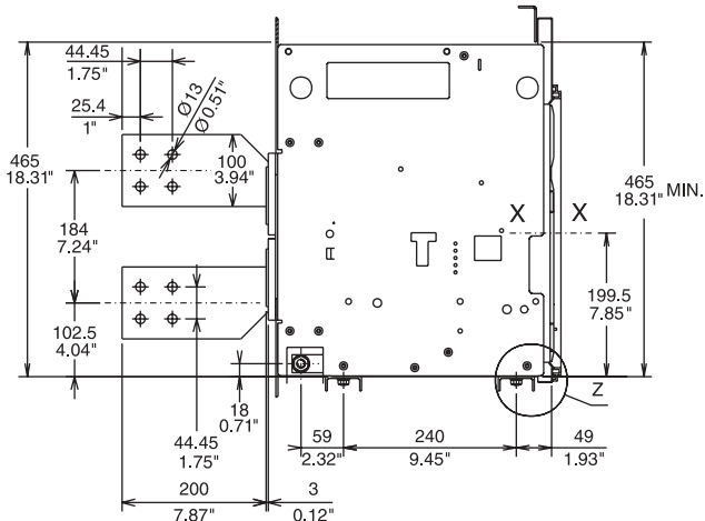
E3 2500 A/3200 A
