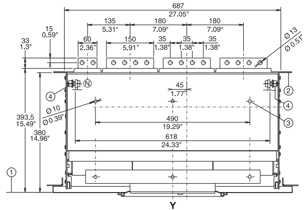
E4 4 poles
