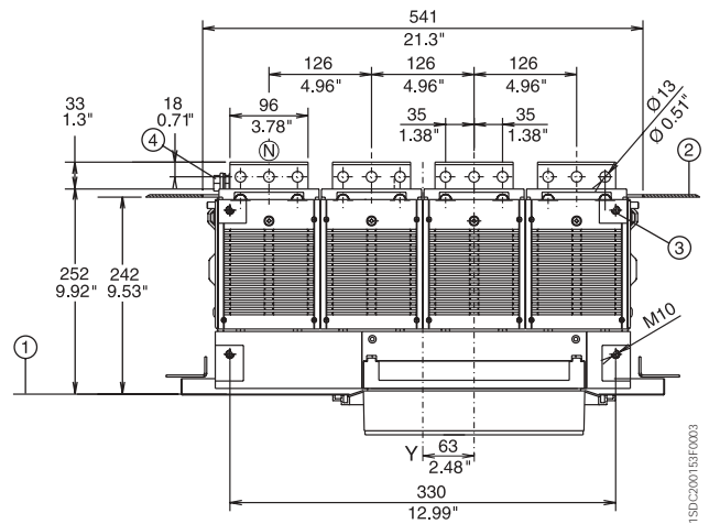
E3 4 poles
