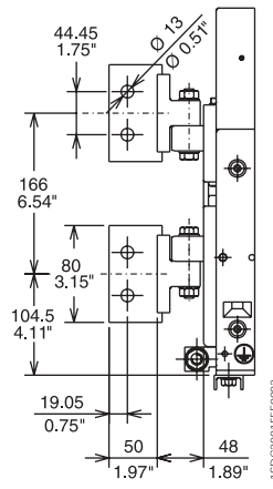
E3 1200÷2000 A
