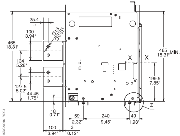
E3 1200÷2000 A
