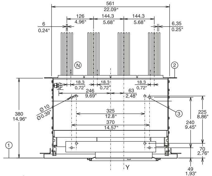
E3 4 poles 3200 A
