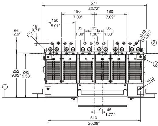
E4 3 poles
