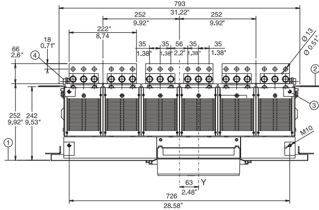
E6 3 poles
