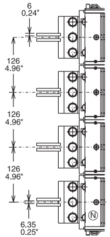
E3 1200÷2000 A
