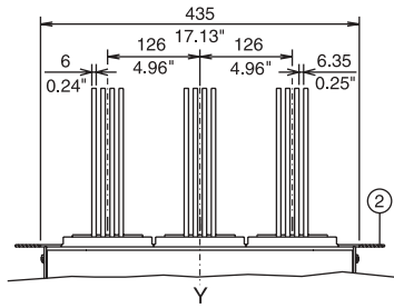
E3 3 poles 3200 A
