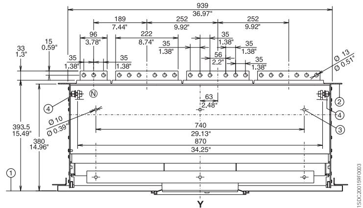
E6 4 poles
