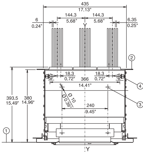
E3 3 poles 3200 A
