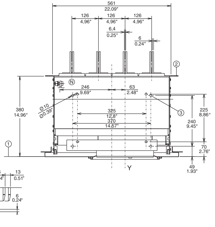
E3 4 poles 1200÷2000 A
