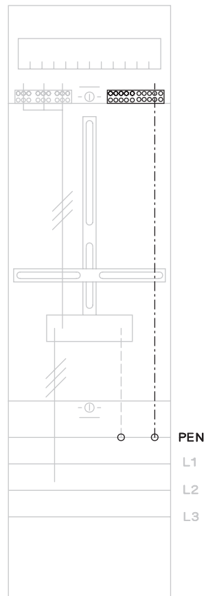
TN-C-System
