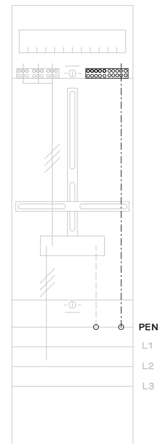
TN-C-System
