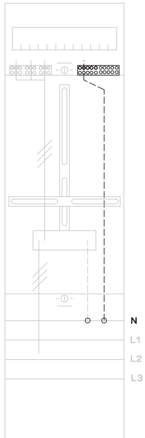
TT-System
