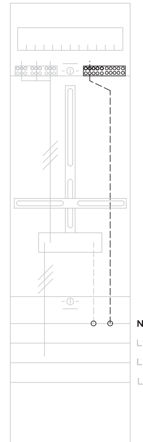
TT-System
