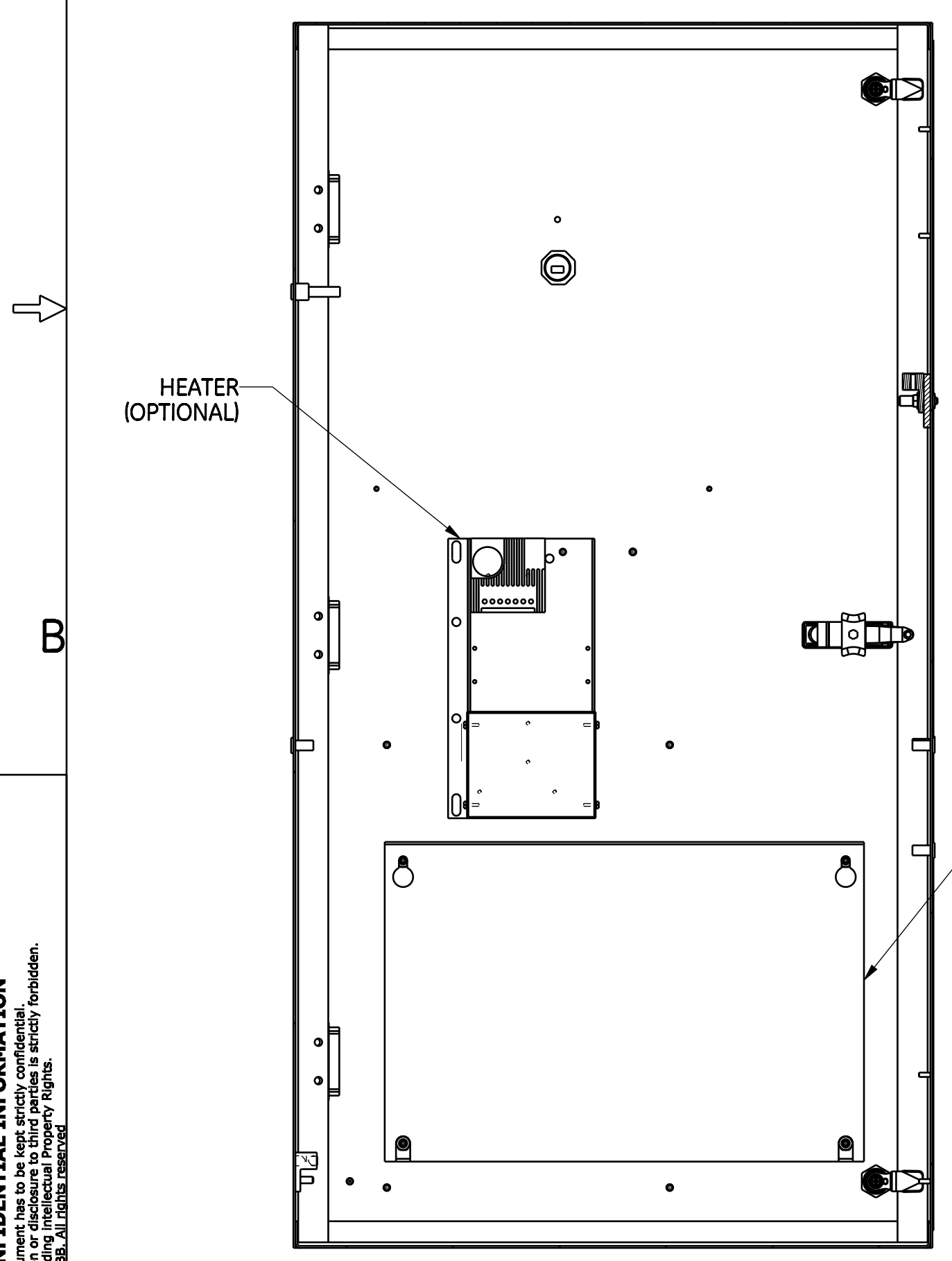
SECTION D-D DOOR INSIDE VIEW
