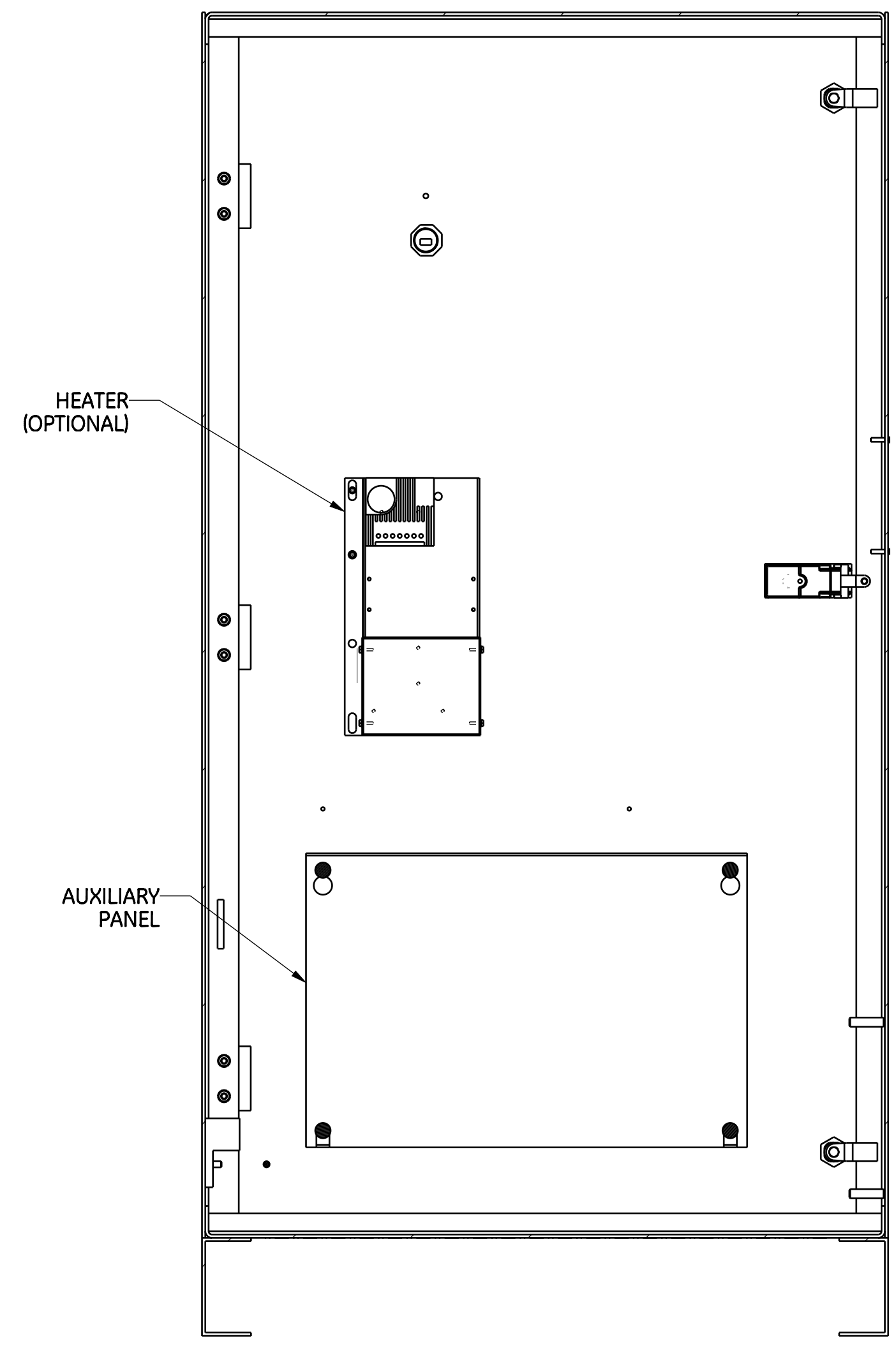
SECTION D-D DOOR INSIDE VIEW
