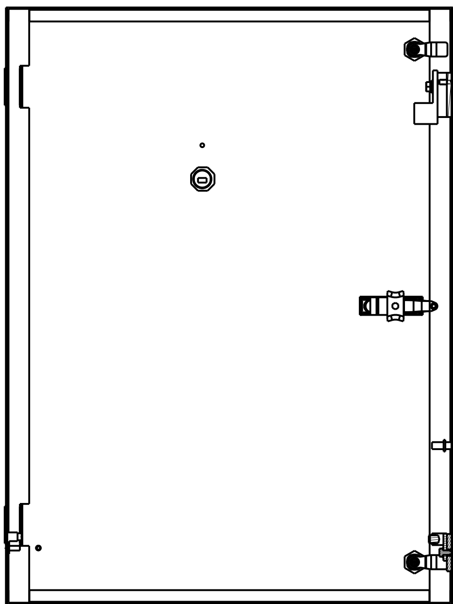
SECTION D-D DOOR INSIDE VIEW
