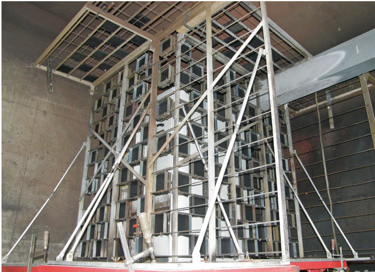
— Configuration pour un essai de résistance aux arcs internes
