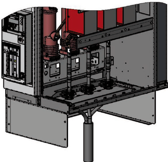
Conessioni cavi a tre poli
