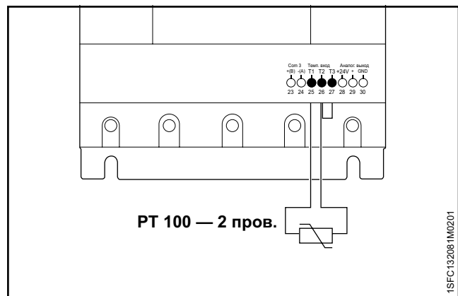
Рис. 5.22 PT100 — 2 пров.
