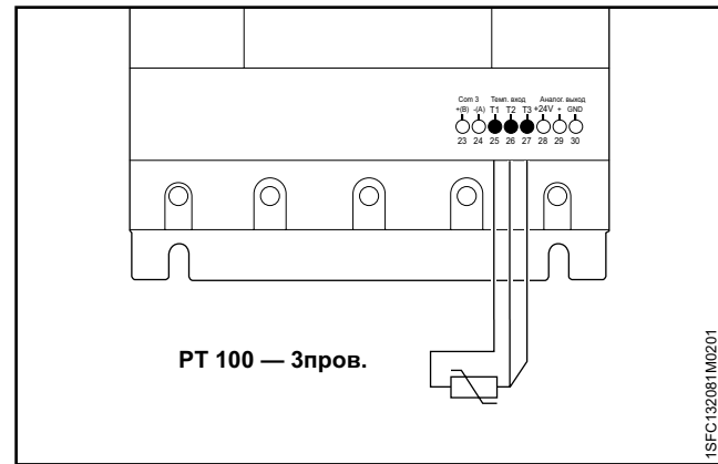
Рис. 5.21 PT100 — 3 пров.
