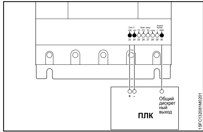
Рис. 5.20 Modbus RTU
