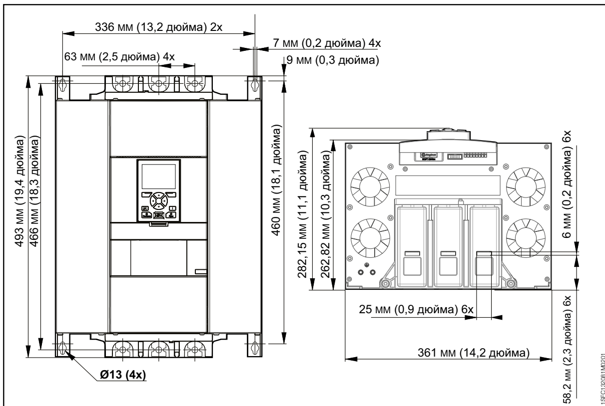
Рис. 3.6 Габариты PSTX470...570
