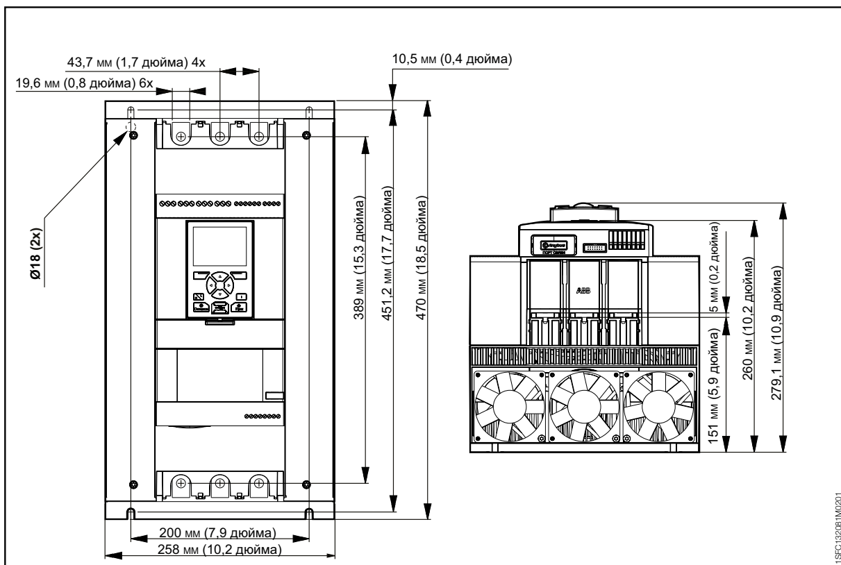
Рис. 3.5 Габариты PSTX210...370
