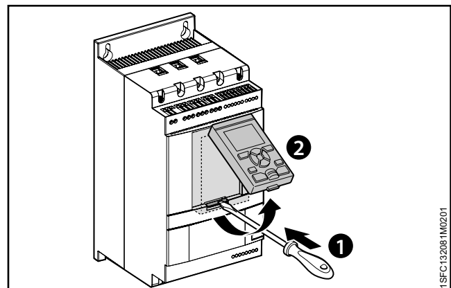
Рис. 4.8 Отсоединение клавиатуры
