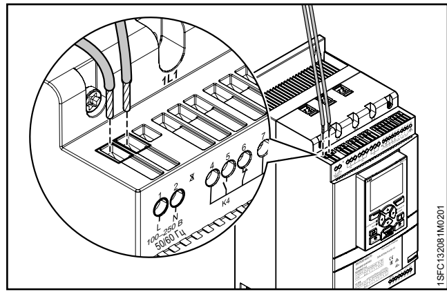
Рис. 5.4 Напряжение питания и цепь управления
