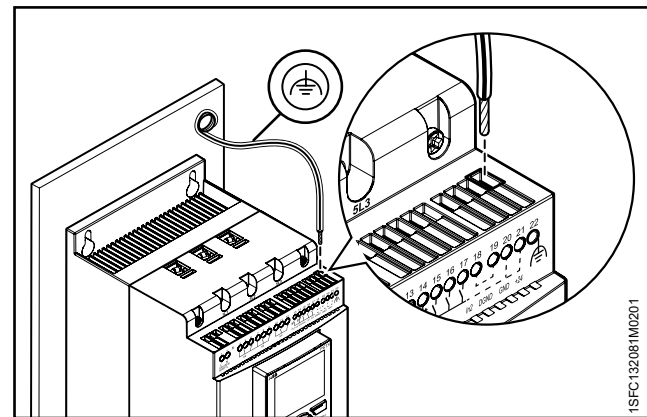
Рис. 5.5 Рабочее заземление, клемма 22
