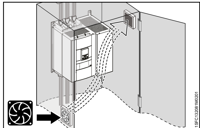
Рис. 4.6 Воздушный поток
