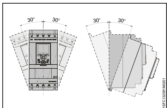
Рис. 4.7 Максимальный угол установки
