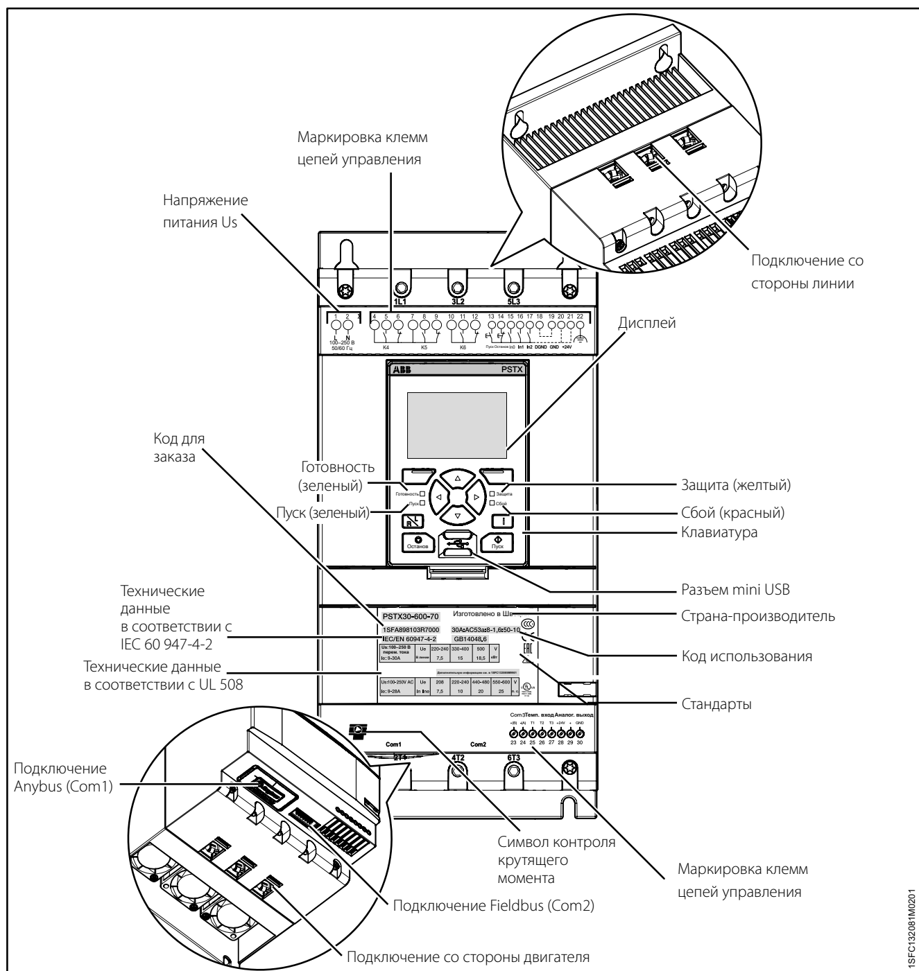
Рис. 3.1 Обзор устройства плавного пуска
