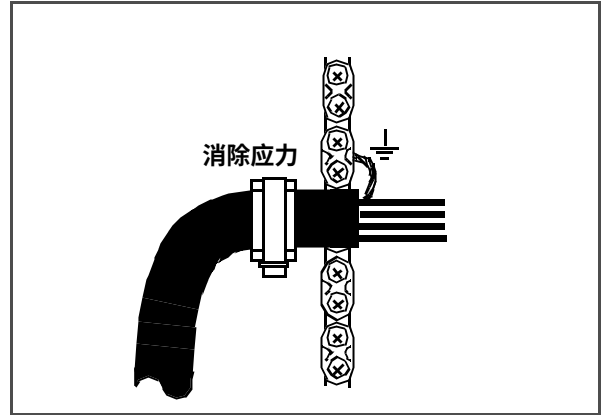
单屏蔽电缆
