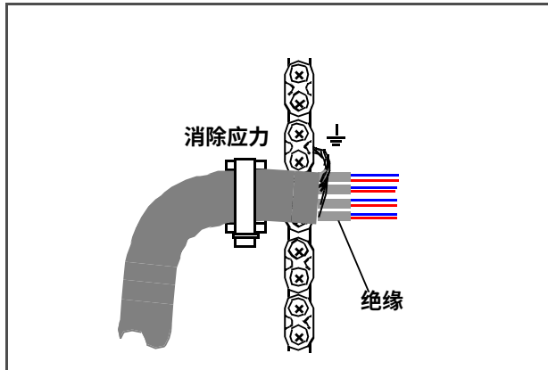
双屏蔽电缆
