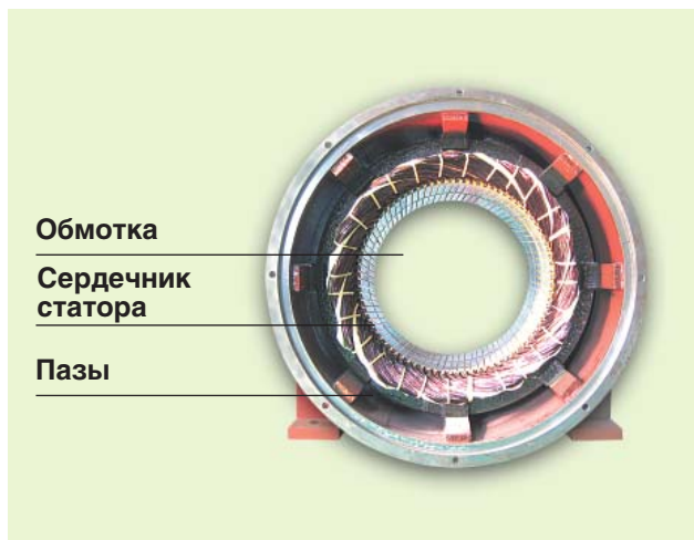
Рисунок 1. Статор трехфазного асинхронного двигателя
