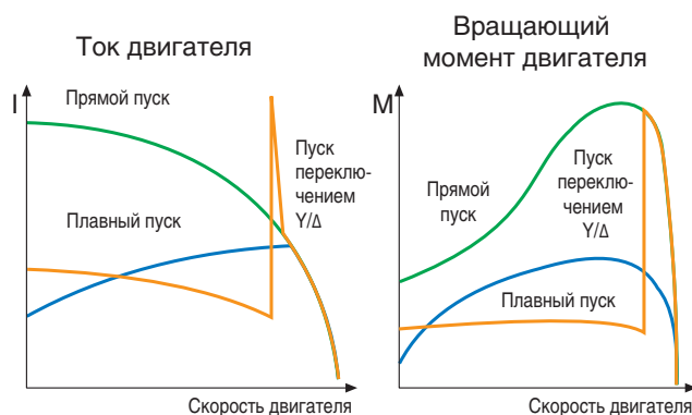
Рисунок 10. Кривые тока и вращающего момента двигателя для различных методов пуска
