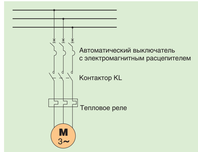
Рисунок 5. Принципиальная схема прямого пуска
