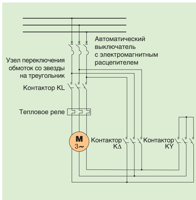
Рисунок 6. Принципиальная схема пуска двигателя переключением по схеме звезда/треугольник
