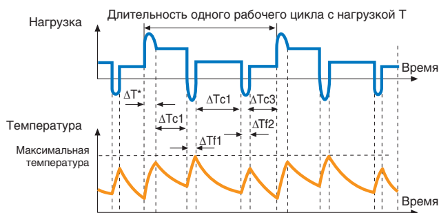
Периодический непрерывный режим с взаимозависимыми изменениями нагрузки и частоты вращения: типовой режим работы S8
