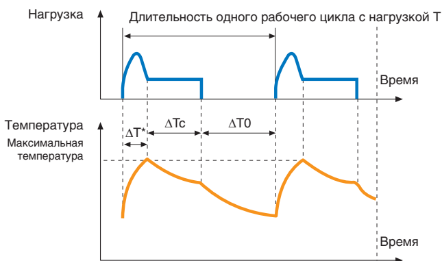
Периодический повторно-кратковременный режим с длинными пусками: Типовой режим работы S4
