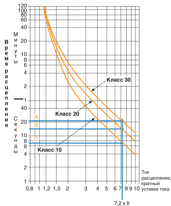
Рисунок 4. Время-токовые характеристики тепловых реле с различными классами расцепления
