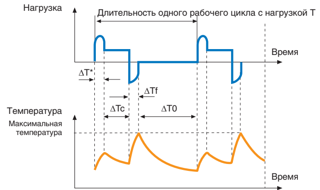
Периодический повторно-кратковременный режим с динамическим торможением: Типовой режим работы S5
