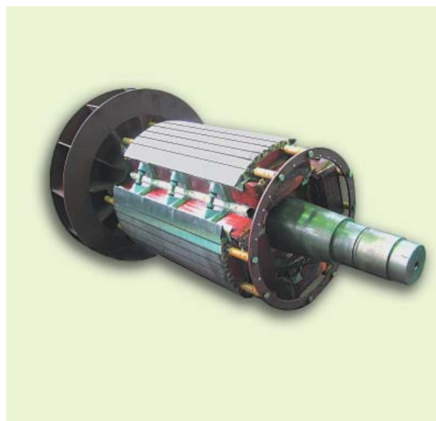
Рисунок 2. Ротор трехфазного асинхронного двигателя
