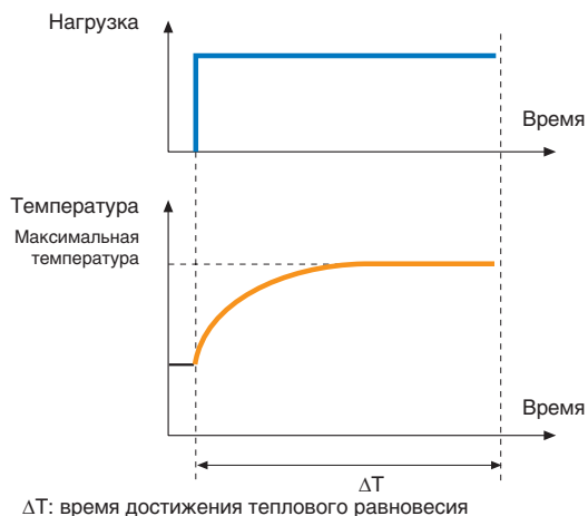
Продолжительный режим работы. Типовой режим работы S1
