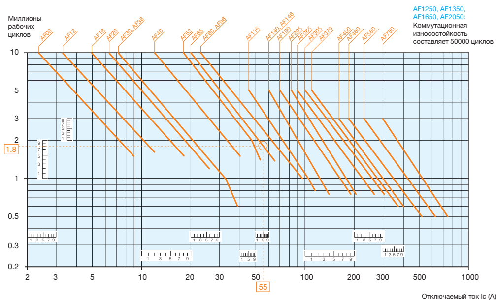
Рисунок 14. График коммутационной износостойкости контакторов для категории применения АС-3, напряжения менее 440 В и температуры окружающей среды менее 55 °С
