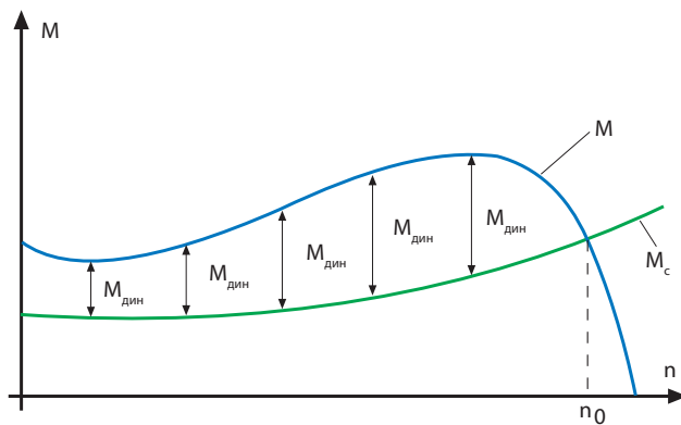
Рисунок В1. Типичные кривые вращающего момента
