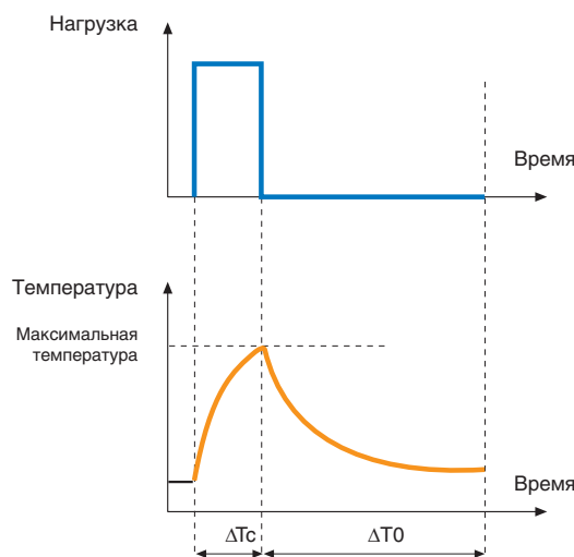
Кратковременный режим. Типовой режим работы S2
