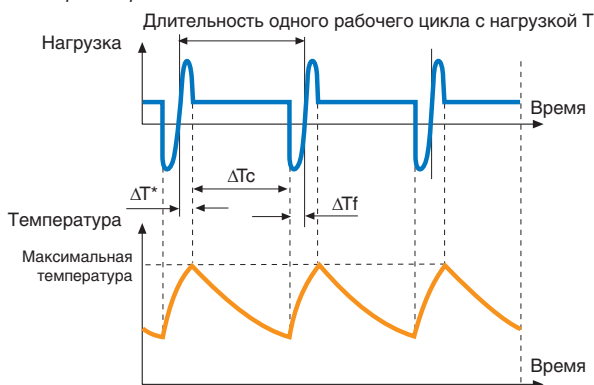
Периодический непрерывный режим с динамическим торможением: типовой режим работы S7
