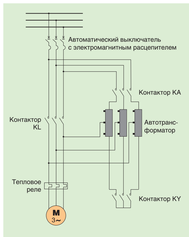
Рисунок 7. Принципиальная схема автотрансформаторного пуска
