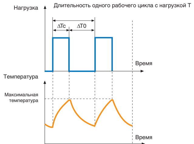
Периодический непрерывный режим с кратковременной нагрузкой: типовой режим работы S6
