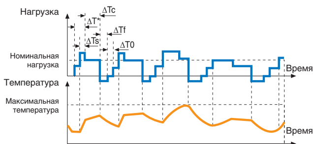
Режим работы с непериодическими изменениями нагрузки и частоты вращения: типовой режим работы S9
