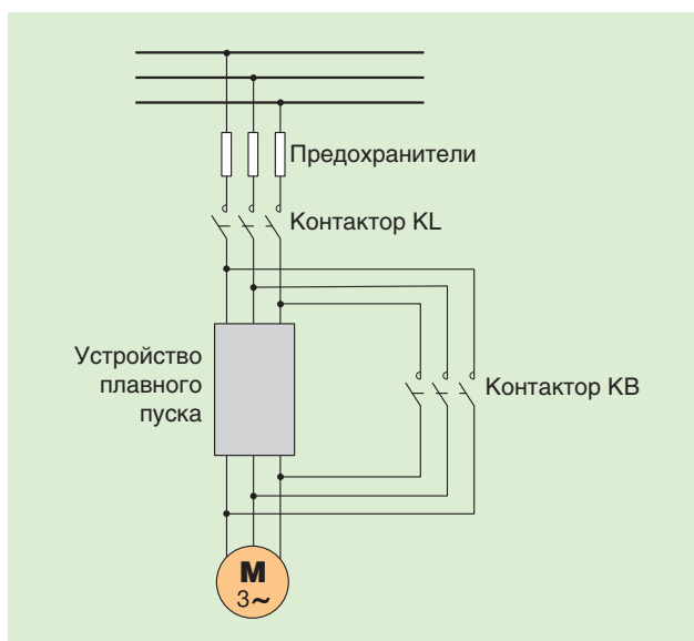
Рисунок 9. Принципиальная схема плавного пуска
