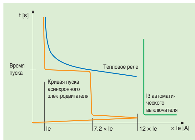
Рисунок 11. Время-токовые характеристики для пуска двигателя, параметры теплового реле и электромагнитного расцепителя
