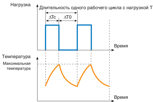
Периодический повторно-кратковременный режим: Типовой режим работы S3
