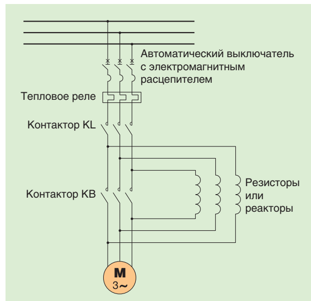
Рисунок 8. Принципиальная схема реостатного пуска
