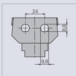
2x BNC-/ TNC разъемы паяного соединения для Busch-Jaeger № арт. 1855 EB
