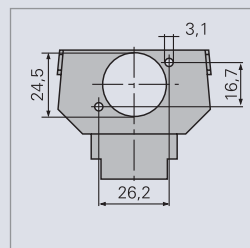
XLR разъем Neutrik, тип FP Busch-Jaeger № арт. 1853 EB
