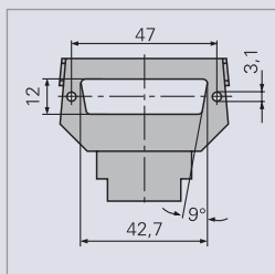
Разъем D-Sub 25 полюсов Busch-Jaeger № арт. 1852 EB Принадлежности: Разъем D-Sub 25 полюсов № арт. 0202
