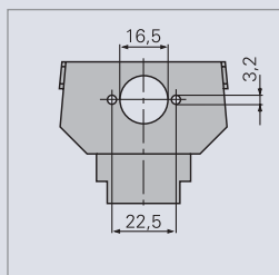
Диодный разъем для вин- тового крепления Busch-Jaeger № арт. 1860 EB
