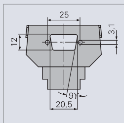
Разъем D-Sub 9 полюсов Busch-Jaeger № арт. 1850 EB Принадлежности: Разъем D-Sub 9 полюсов № арт. 0200
