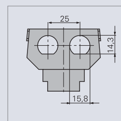
2x Разъем UHF Busch-Jaeger № арт. 1859 EB
