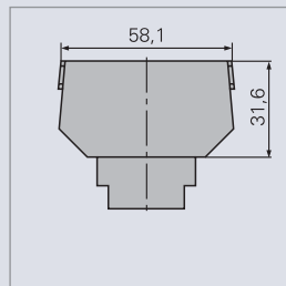
Заглушка. Busch-Jaeger № арт. 1869 EB
