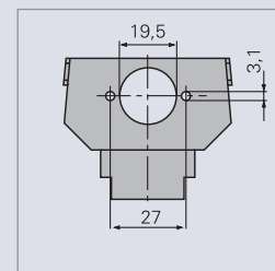
XLR разъем Neutrik, тип MP Busch-Jaeger № арт. 1854 EB
