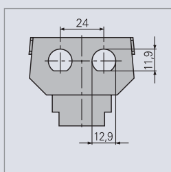
2x BNC-/ TNC кабельных разъемов Busch-Jaeger № арт. 1857 EB
