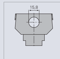
Разъем Twinax Busch-Jaeger № арт. 1864 EB
