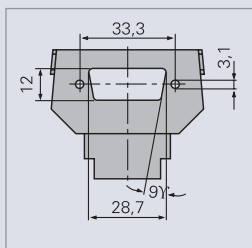
Разъем D-Sub 15 полюсов Busch-Jaeger № арт. 1851 EB Принадлежности: Разъем D-Sub 15 полюсов № арт. 0201
