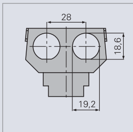
2x Twinax разъема Busch-Jaeger № арт. 1865 EB
