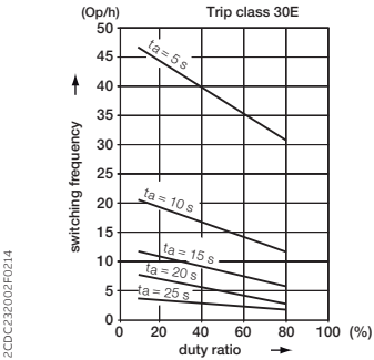
Trip class 30E
