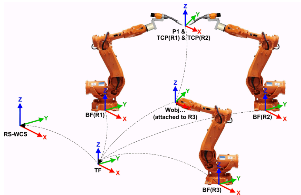
en1000001306_Coordinated_MultiMove_OneRobot
