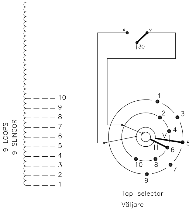
Diverter switch Lastkopplare
