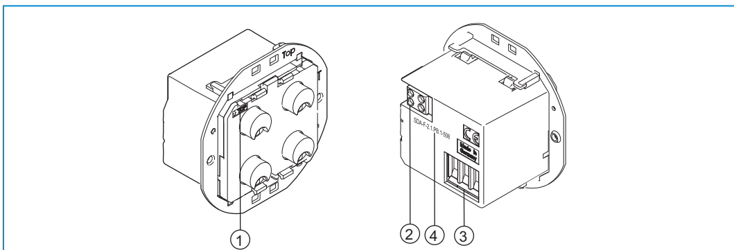
Abb. 3: Geräteübersicht Sensor/Dimmaktor 2/1-fach
