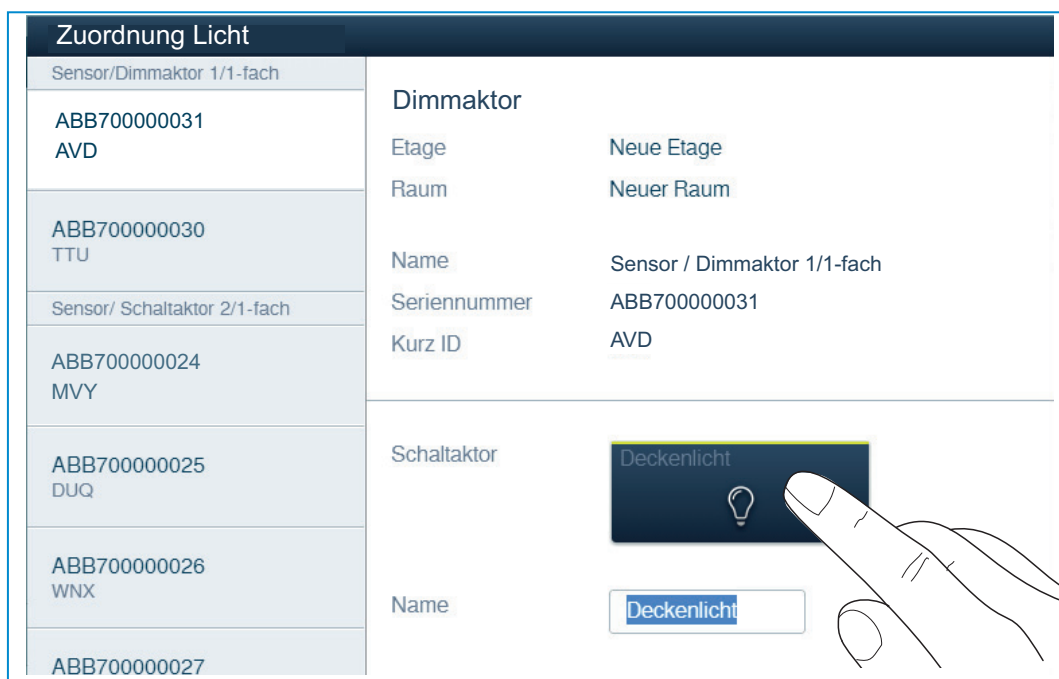
Abb. 11: Identifikation durch Schalten
