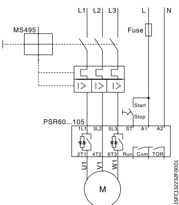
PSR60 ... PSR105 Avec MMS
