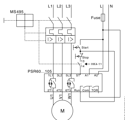
Avec MMS et contact auxiliaire
