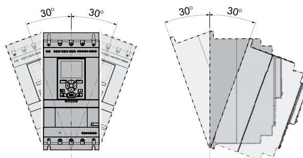
Angle de montage maximal
