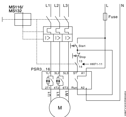
Avec MMS et contact auxiliaire
