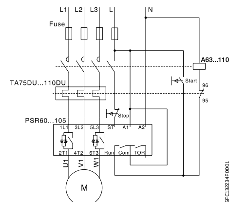
Avec fusibles, contacteur et O.L.
