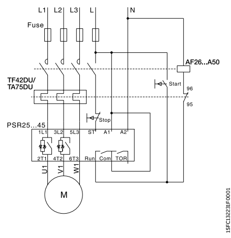
Avec fusibles, contacteur et O.L.
