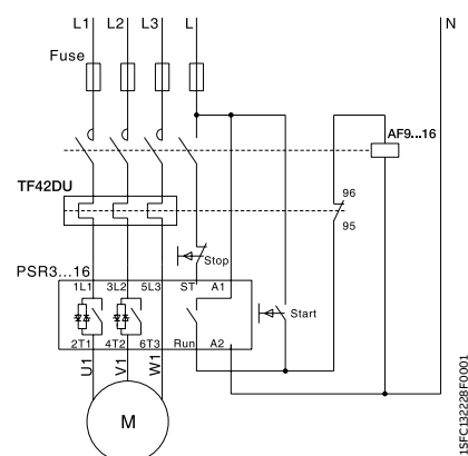
Avec fusibles, contacteur et O.L.
