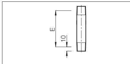
E2S or E3S nipple 2 x 1/2 in. NPT
