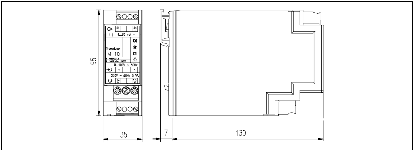
Bild 1 Maßbild (Maße in mm) Z-18547
