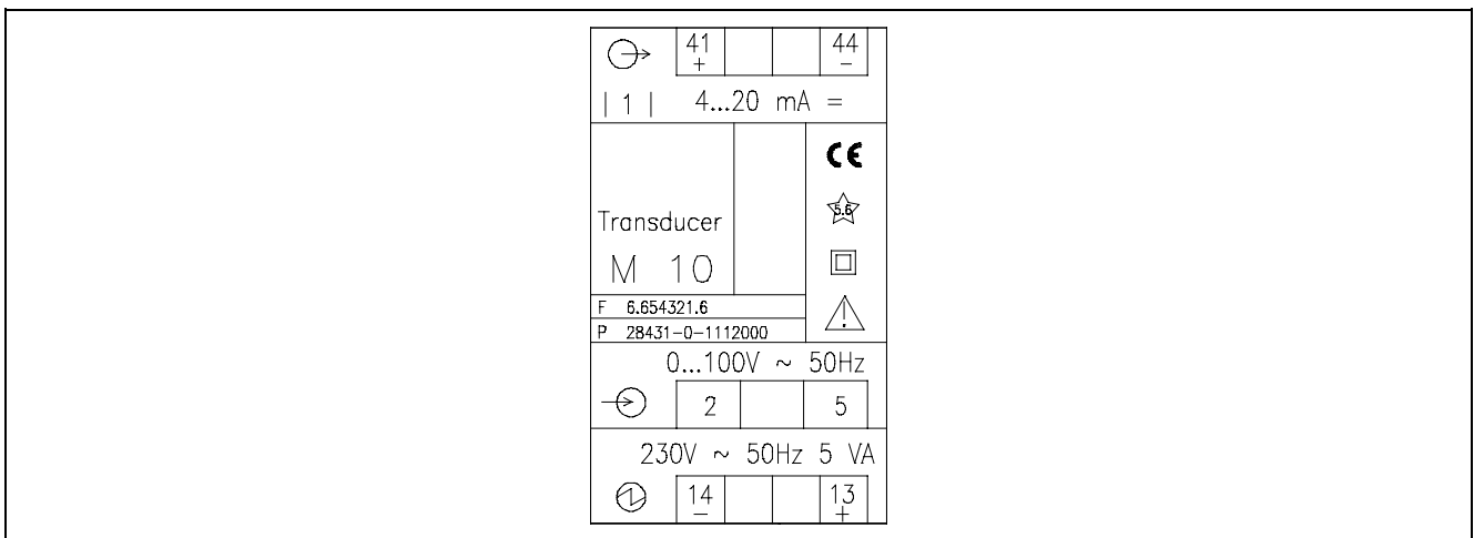
Bild 2 CE ★ □ ⚠ 2, 5 1, 3 13, 14 41, 44 F P Z-18547 Anschließen CE-Zeichen Prüfspannung Schutzklasse Gebrauchsanweisung beachten Eingang Spannung Eingang Strom Energieversorgung Ausgang Fertigungsnummer Bestellnummer
