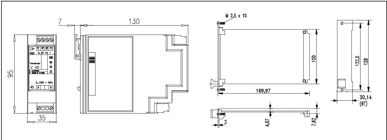
Bild 1 Maßbild (Maße in mm) Z-18537A Z-18537S
