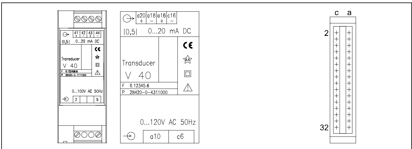
Bild 2 Anschließen CE CE-Zeichen ★ Prüfspannung ☐ Schutzklasse ⚠ Gebrauchsanweisung beachten F Fertigungsnummer P Bestellnummer Z-18002
