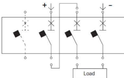
4P 外形
