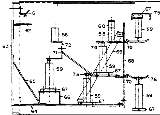
Fig. 14. Fuse rollout unit
