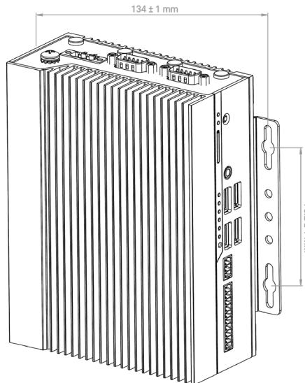
Монтаж на DIN-рейке за боковую поверхность
