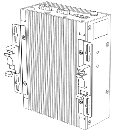
Монтаж на DIN-рейке за заднюю поверхность
