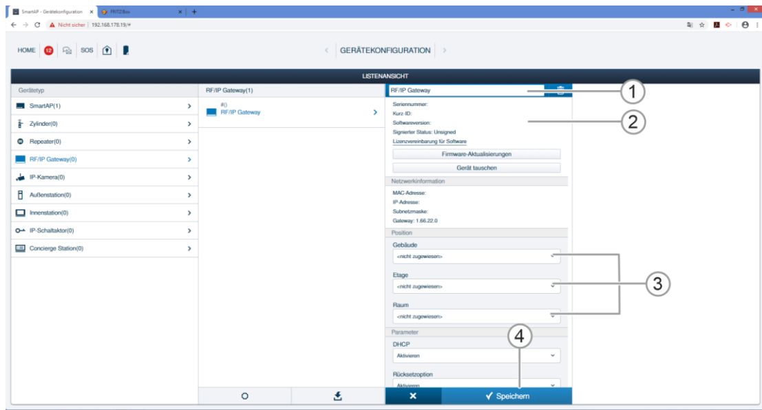
Abb. 91: „RF/IP Gateway“ Eigenschaften
