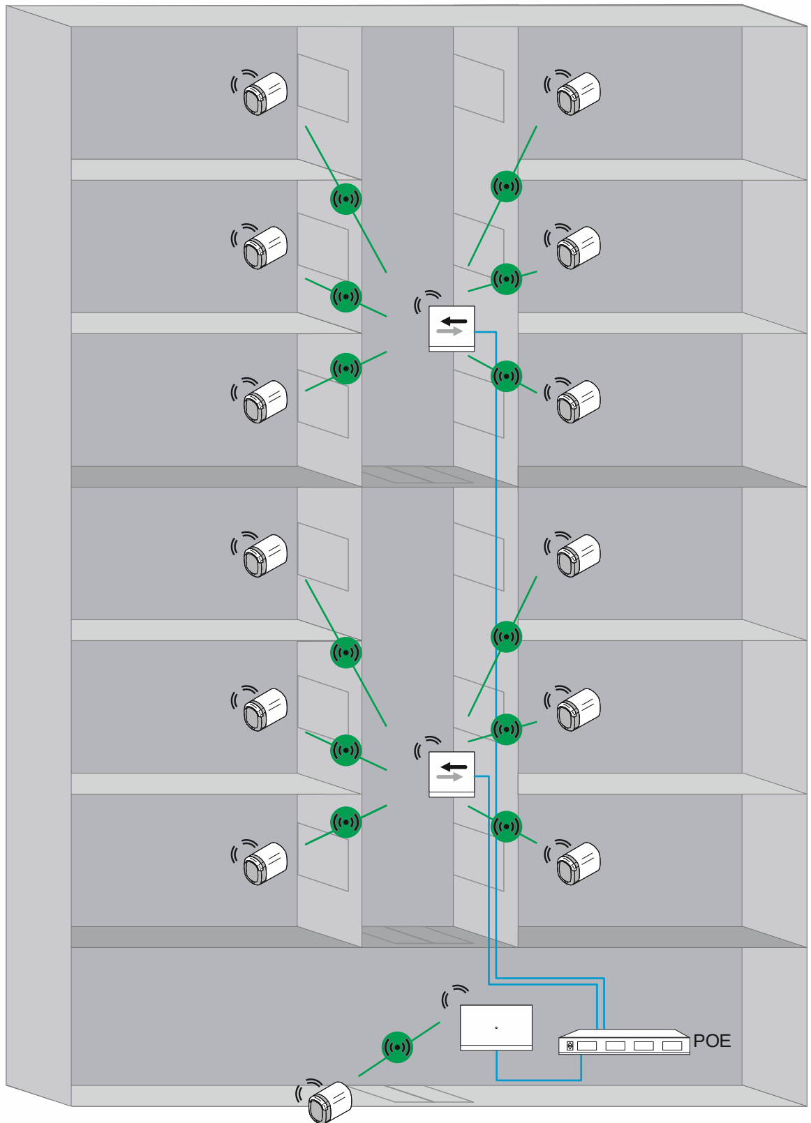
Abb. 59: Übersicht (Draufsicht): Wohngebäude mit mehr als 10 Meter Übertragungsstrecke und Funksignalhemmung durch Feuerschutzwände.
