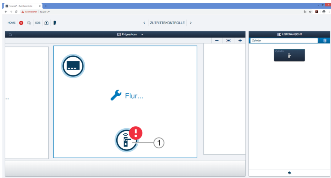
Abb. 159: „Elektronischer Schließzylinder“ entkoppelt
