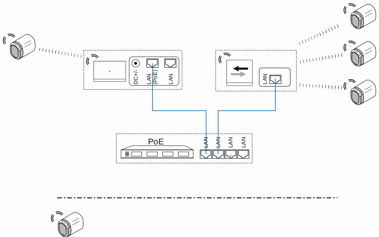
Abb. 57: Anschluss: Mehrfamilienhaus mit Arztpraxis und Archiv
