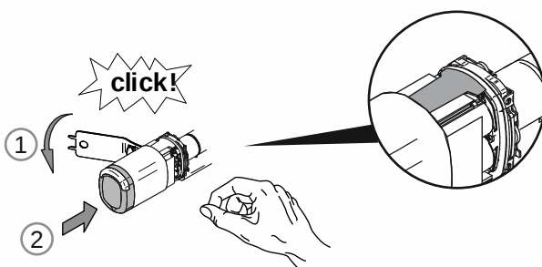
Abb. 37: Knaufgehäuse montieren
