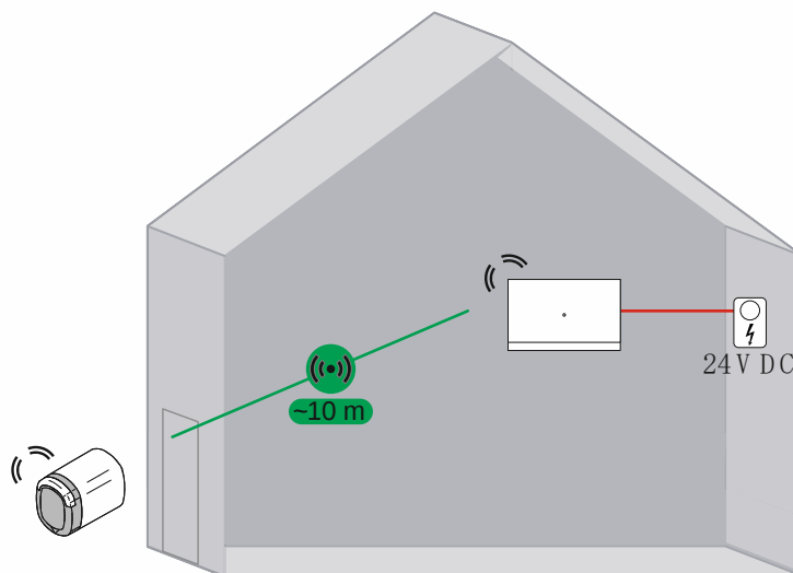
Abb. 47: Übersicht: Einfamilienhaus mit einem „Elektronischer Schließzylinder“
