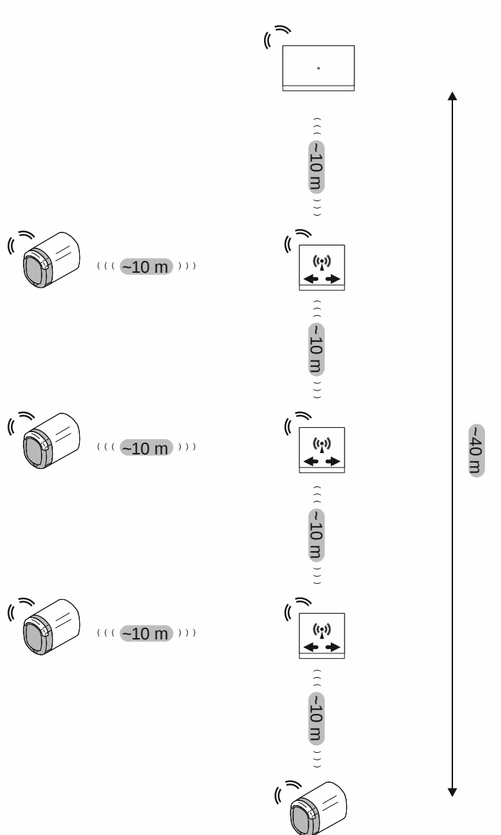
Abb. 44: Funkreichweite zwischen Geräten
