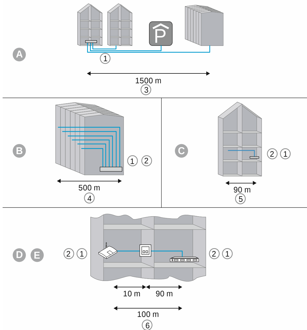
Abb. 2: Strukturierte Verkabelung
