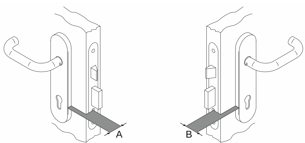
Abb. 9: Schließzylinder ausmessen: Türbreite
