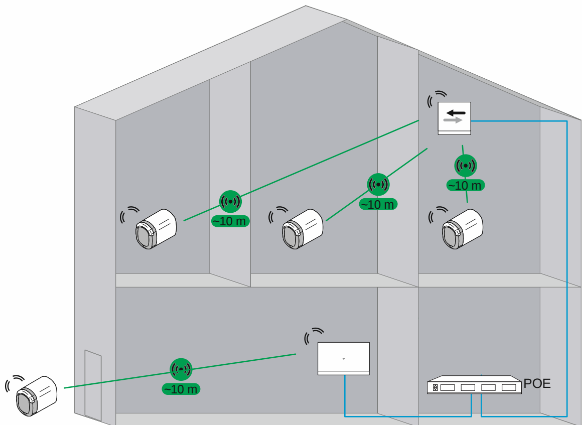
Abb. 53: Übersicht: Mehrfamilienhaus mit 4 „Elektronischer Schließzylinder“
