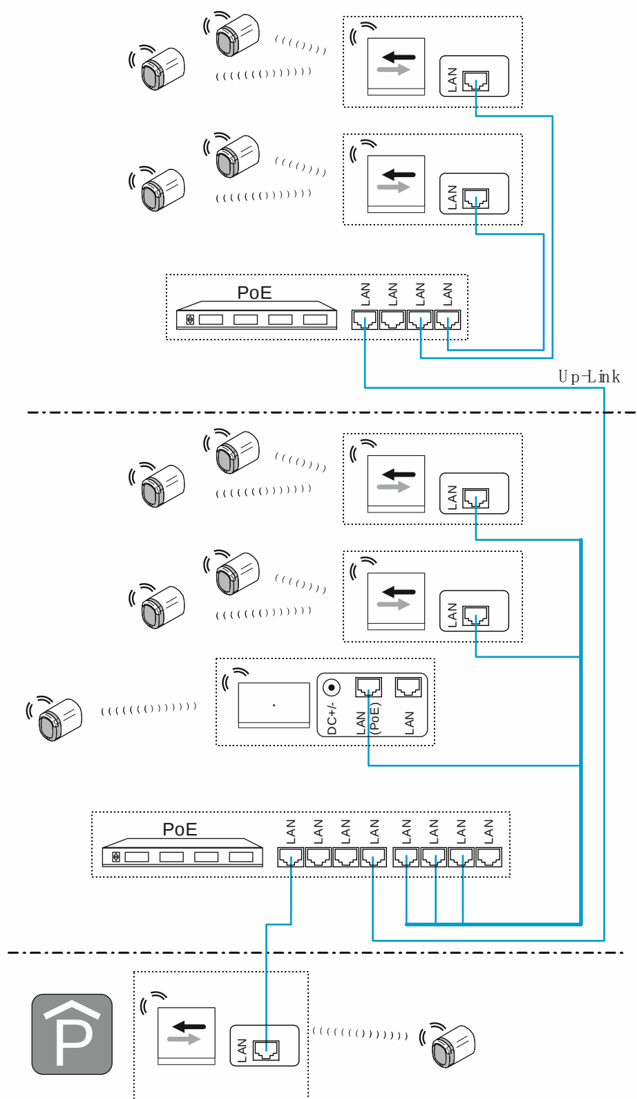
Abb. 66: Anschluss Perimeter mit mehr als 40 Meter Übertragungsstrecke und weniger als 16 „Elektronischer Schließzylinder“
