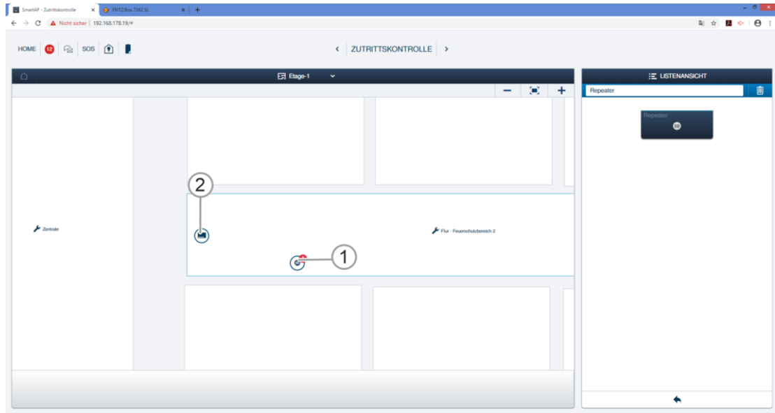
Abb. 119: „RF Repeater“ mit „Smart Access Point Pro“ koppeln
