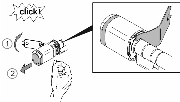
Abb. 34: Knaufgehäuse abziehen
