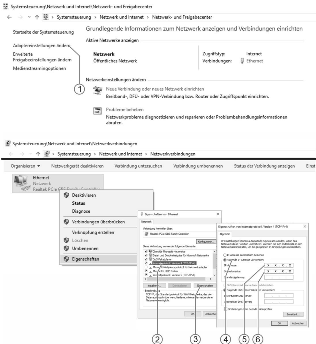
Abb. 33: IP-Adresse im PC einstellen (Beispiel Windows 10)
