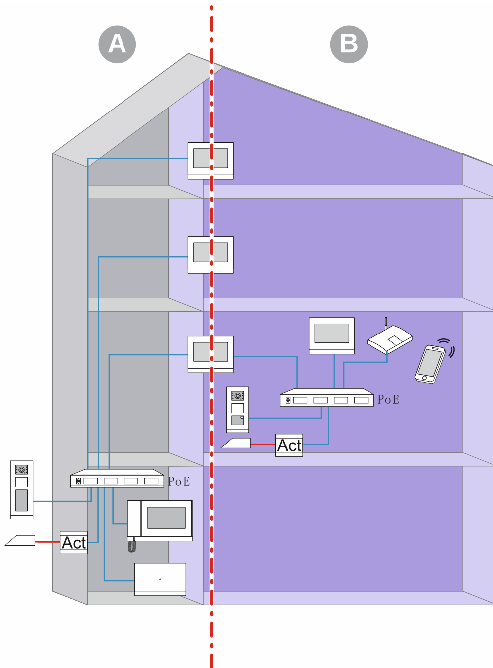
Abb. 15: Vorinformation Auswahl Systemmodi
