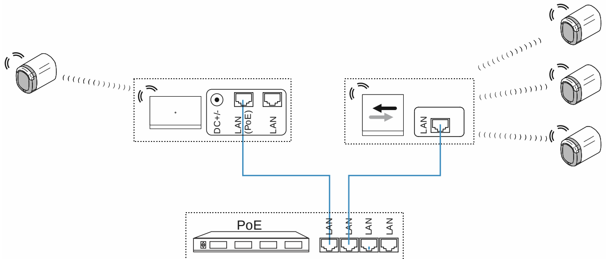
Abb. 54: Anschluss: Mehrfamilienhaus mit 4 „Elektronischer Schließzylinder“
