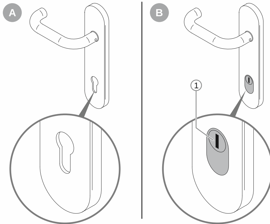
Abb. 7: Montagesituation Sicherheitsbeschläge
