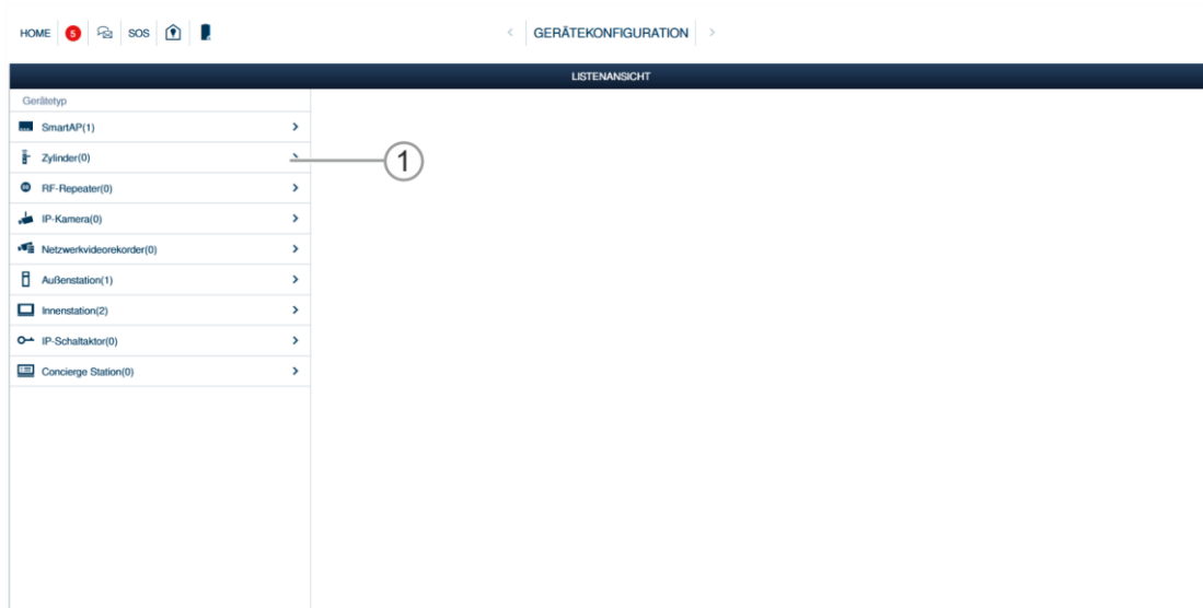
Abb. 83: „Elektronischer Schließzylinder“ hinzufügen
