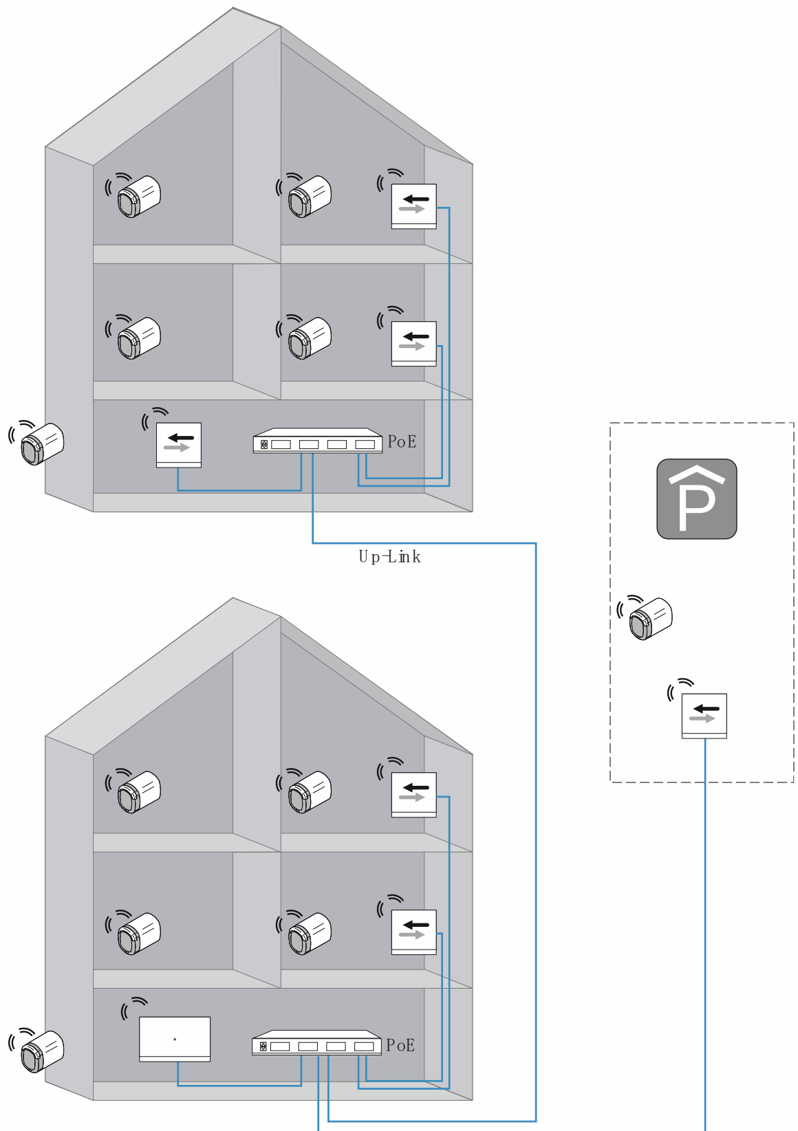
Abb. 65: Übersicht: Perimeter mit mehr als 40 Meter Übertragungsstrecke und weniger als 16 „Elektronischer Schließzylinder“
