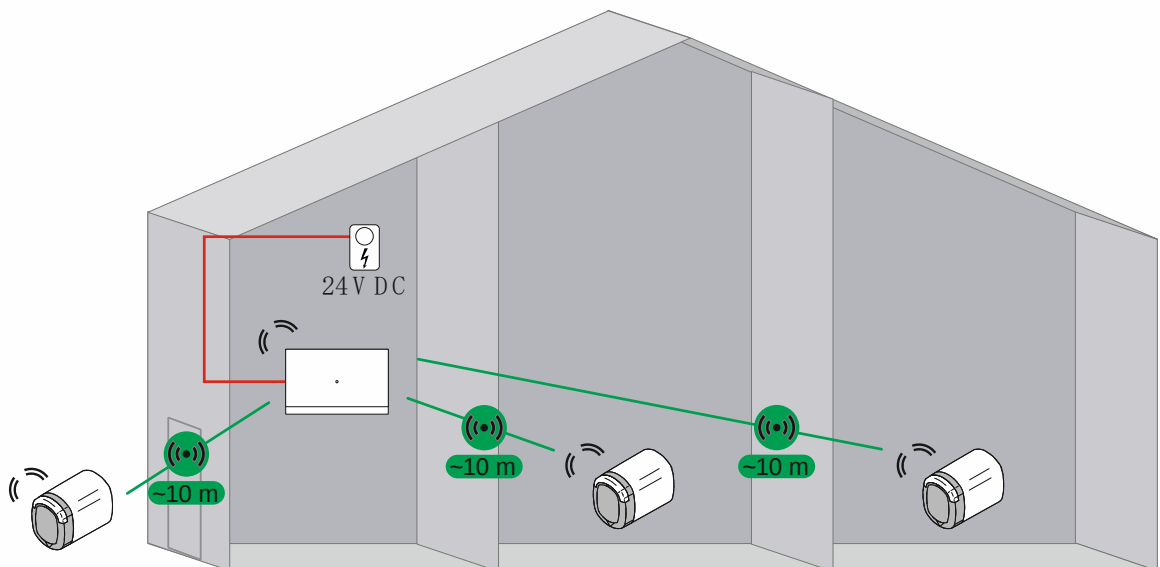
Abb. 50: Übersicht: Mehrfamilienhaus mit 3 „Elektronischer Schließzylinder“
