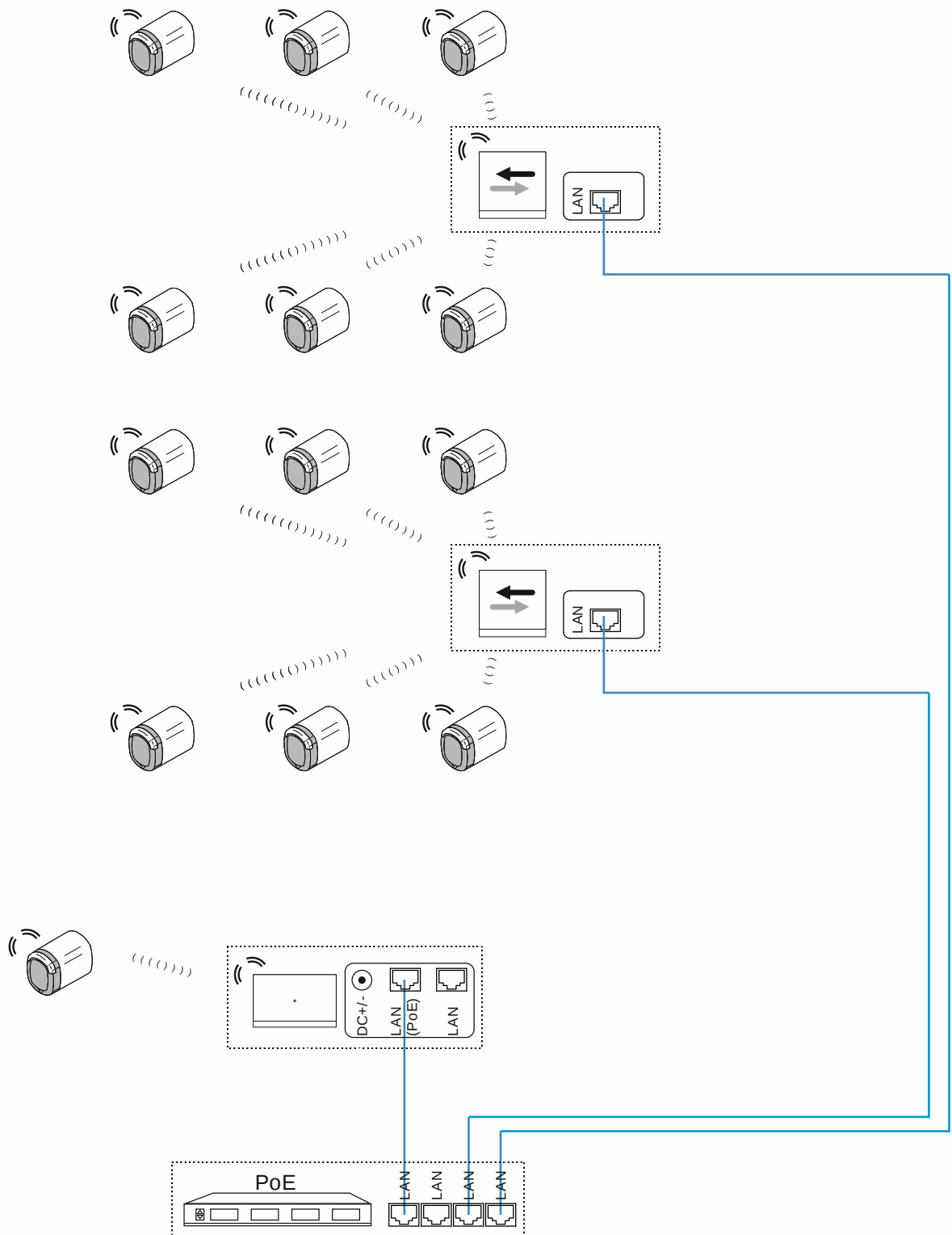
Abb. 60: Anschluss: Wohngebäude mit mehr als 10 Meter Übertragungsstrecke und Funksignalhemmung durch Feuerschutzwände.
