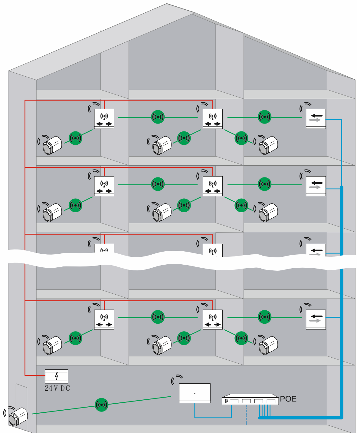
Abb. 62: Übersicht: Mehrgeschossiges Wohngebäude mit mehr als 10 Meter Übertragungsstrecke
