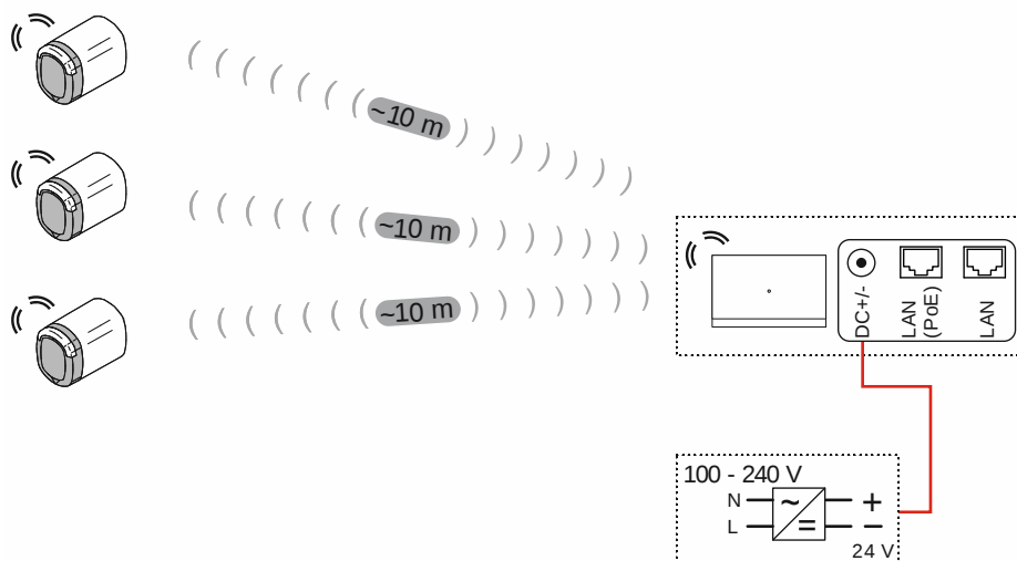
Abb. 51: Anschluss: Mehrfamilienhaus mit 3 „Elektronischer Schließzylinder“
