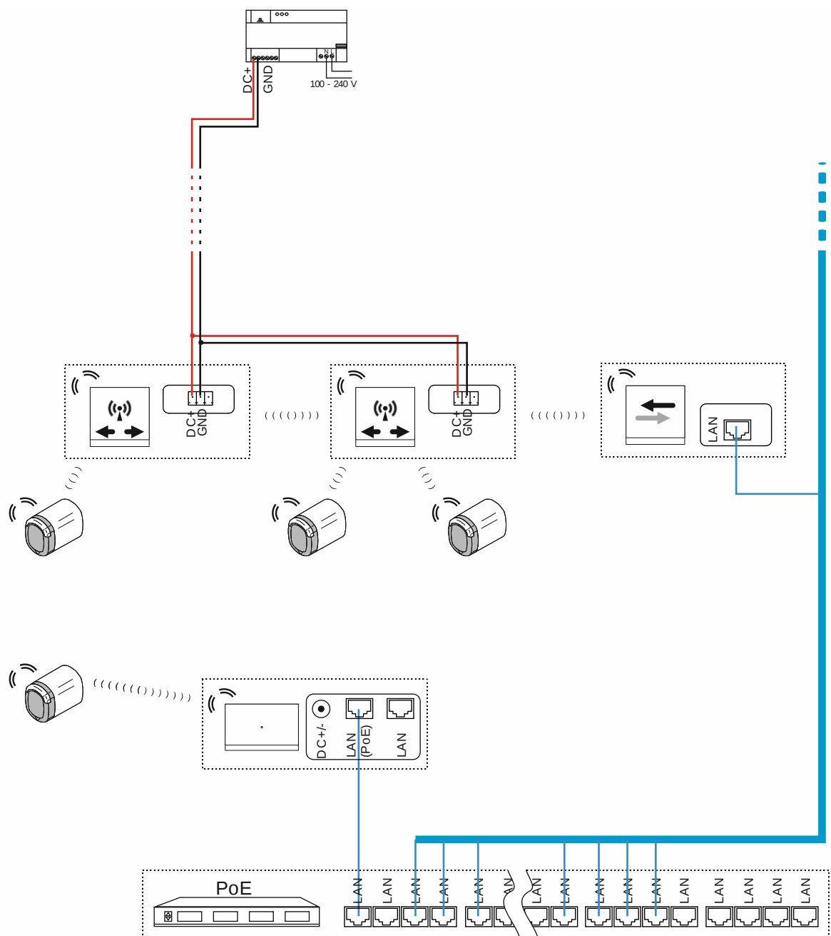
Abb. 63: Anschluss: Mehrgeschossiges Wohngebäude mit mehr als 10 Meter Übertragungsstrecke
