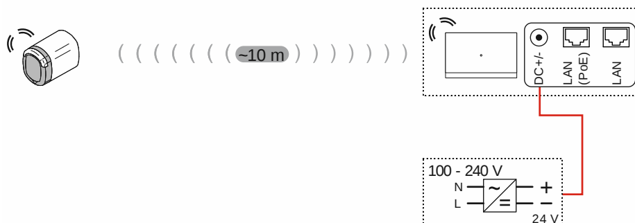
Abb. 48: Anschluss: Einfamilienhaus mit einem „Elektronischer Schließzylinder“
