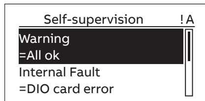
圖 46: LHMI 自監督頁面的內部故障
