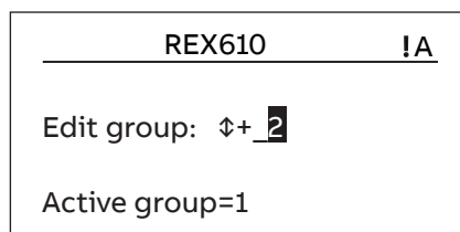
圖 18: 選擇設定群組
