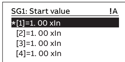
圖 57: 選擇設定群組值
