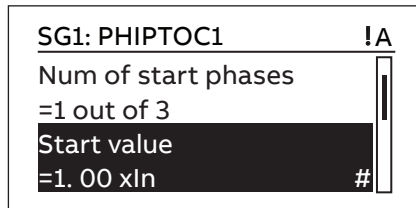
圖 56: 設定群組參數
