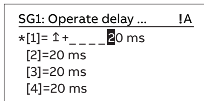
圖 58: 編輯設定群組值
