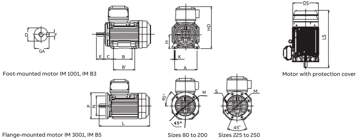
Flange-mounted motor IM 3001, IM B5
