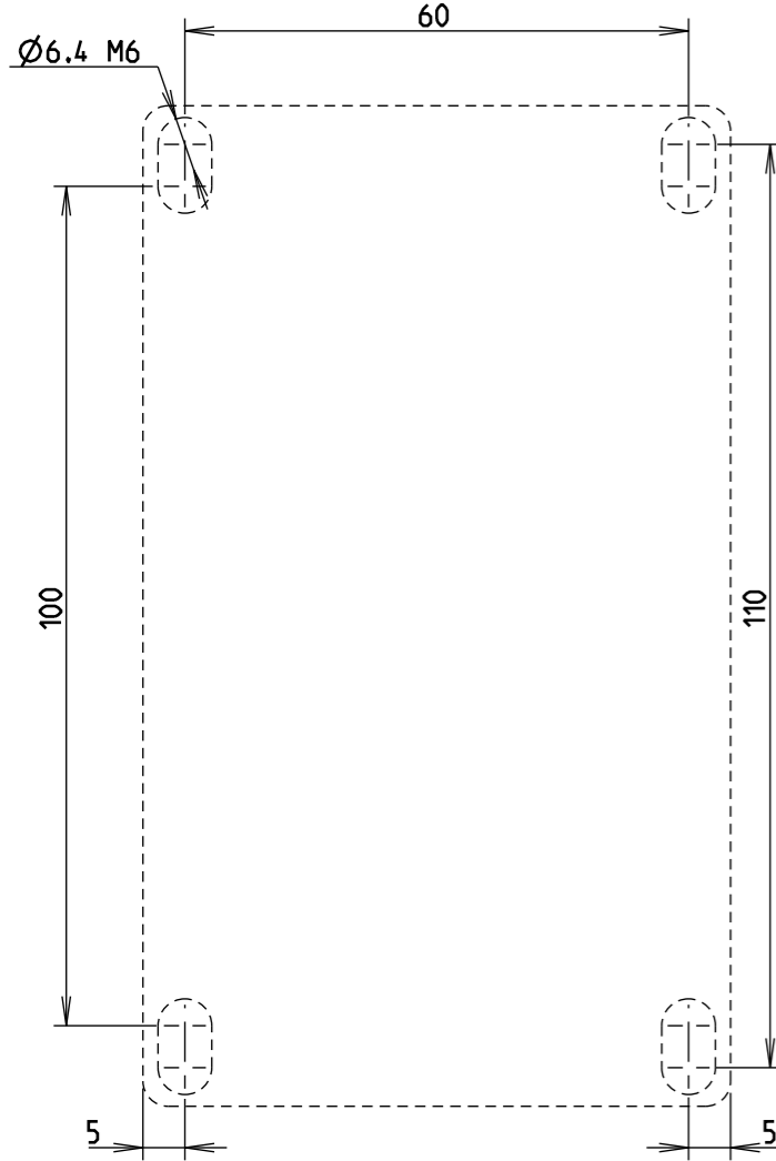
ECHELLE 1:2
