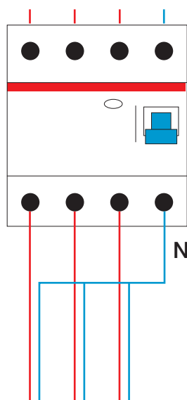
Einphasige Stromkreise
