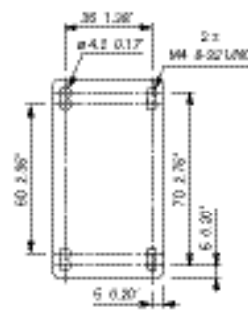
NF22EK, NF31EK, NF40EK
