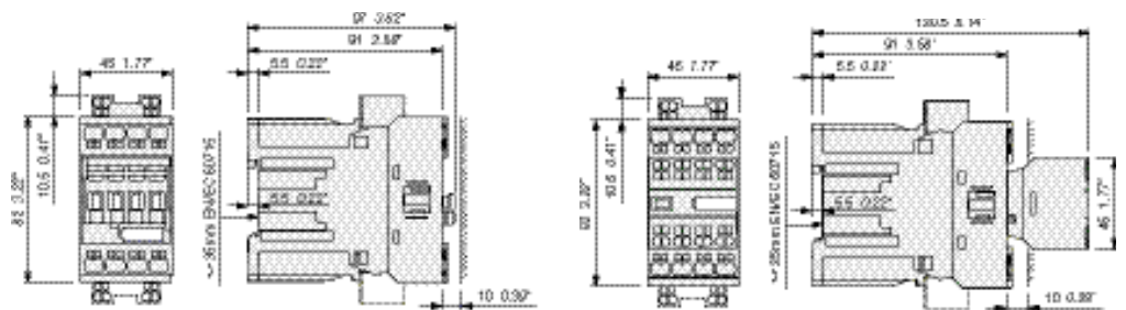
NFZ22EK, NFZ31EK, NFZ40EK
