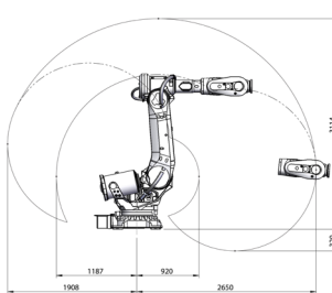
IRB 6700-235/2.65
