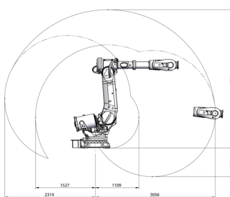
IRB 6700-175/3.05
