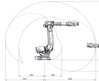
IRB 6700-150/3.20
