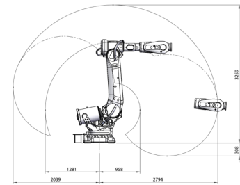
IRB 6700-205/2.80
