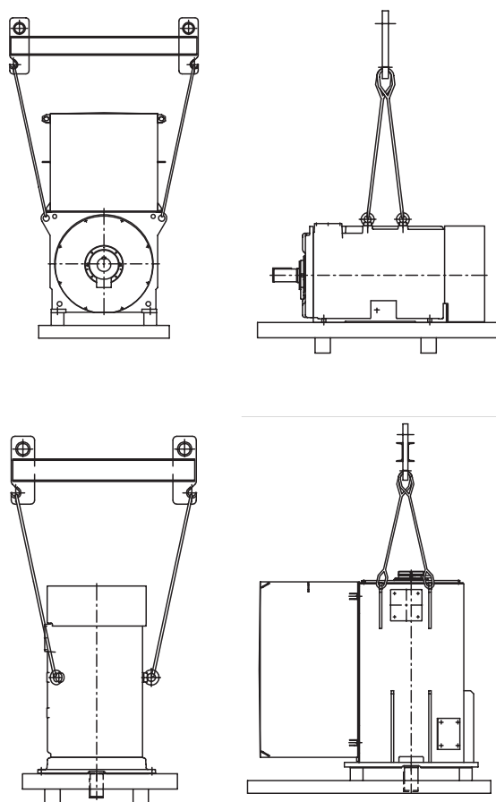
Figure 2-4 Levage de machines horizontales et verticales sur palette
