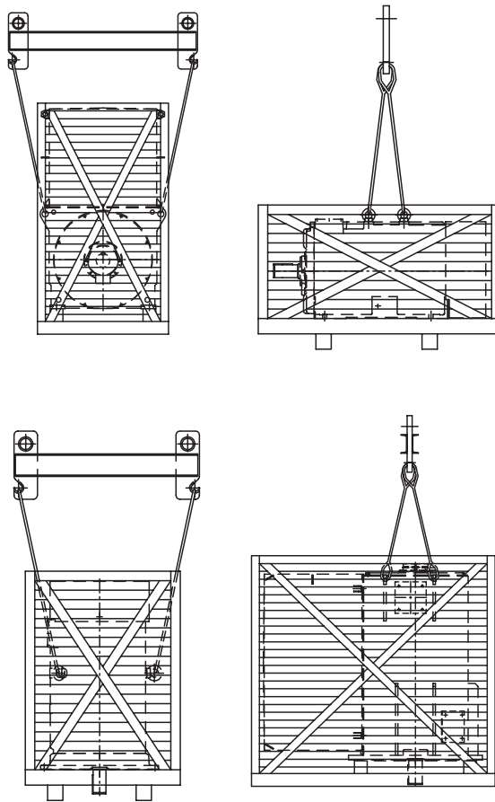
Figure 2-3 Levage de machines horizontales et verticales sous emballage maritime
