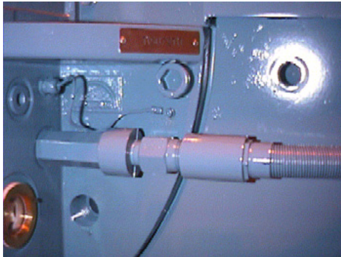
Figure 7-2 Câble de mise à la terre du palier de l'extrémité motrice
