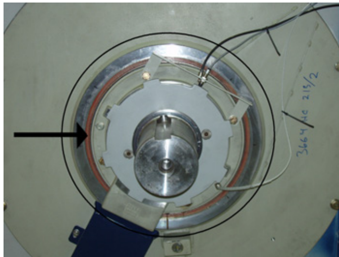
Figure 7-5 Surfaces de flasque et d'isolation du palier
