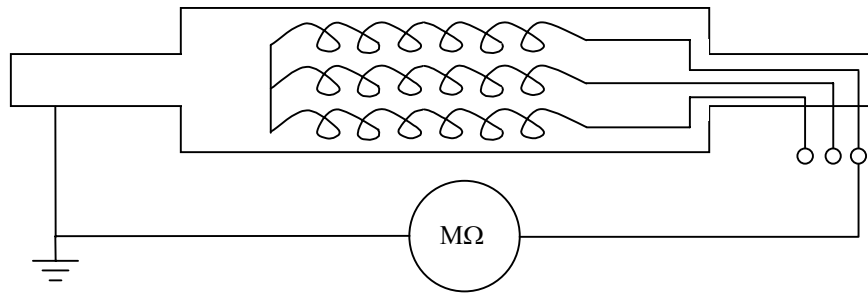
Figure 7-8 Mesure de la résistance d'isolation du bobinage du rotor
