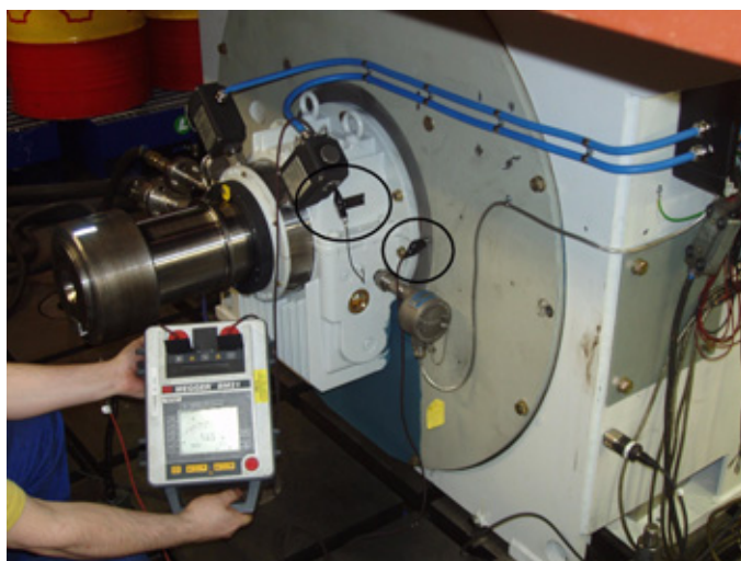
Figure 7-3 Mesure de la résistance d'isolation d'un palier lisse
