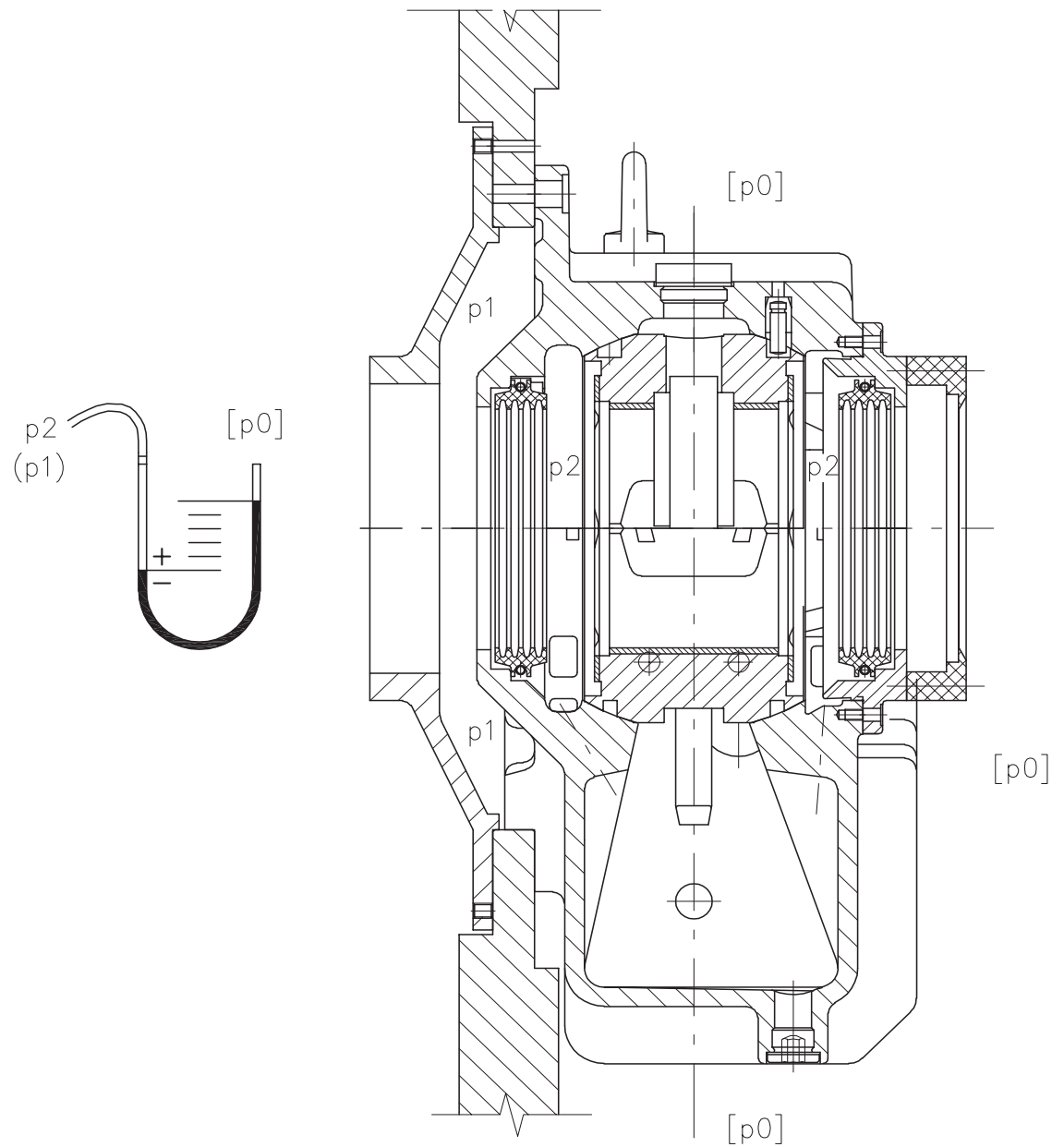
Figure 8-1 Vérification de la pression d'air à l'intérieur ou à l'extérieur d'un palier lisse
