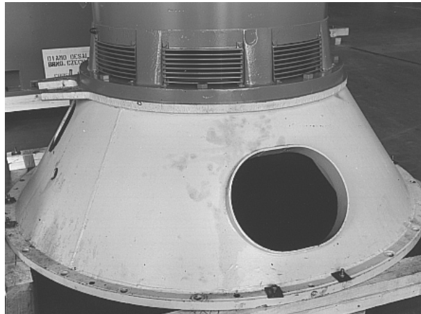
Figure 3-3 Plateau d'accouplement
