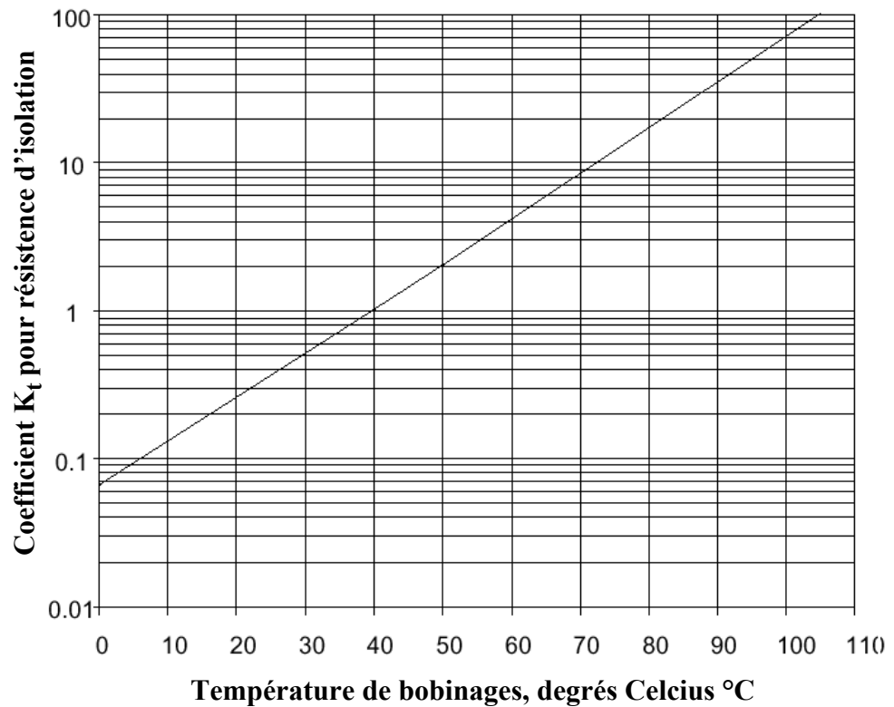
Figure 7-6 Corrélation entre la résistance d'isolation et la température
