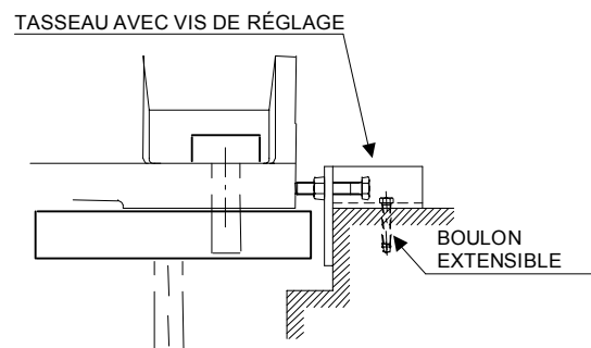
Figure 3-6 Montage d'un tasseau
