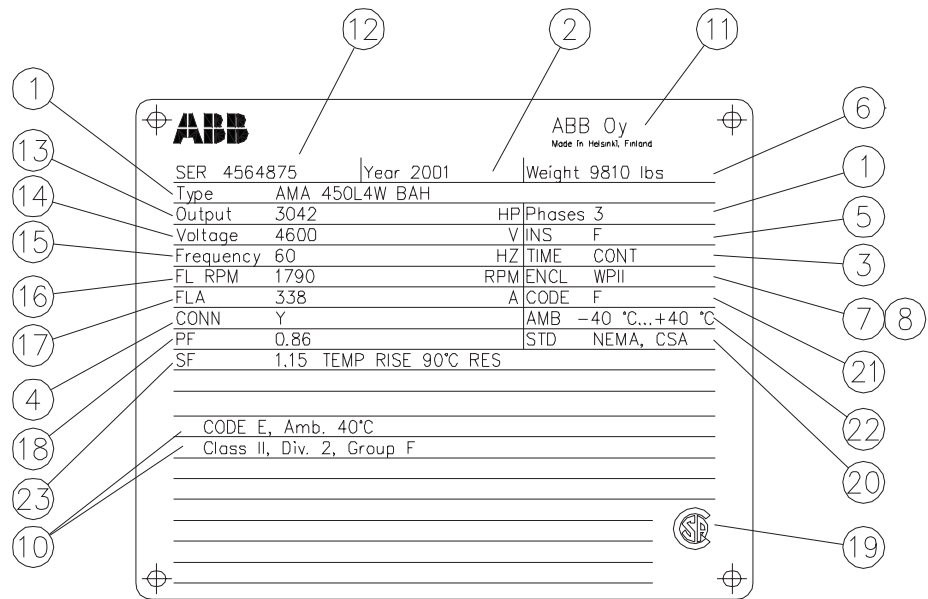
Figure 1-3 Plaque signalétique pour machines en ligne directe construites conformément à la norme NEMA
