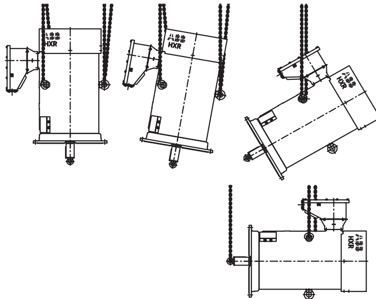
Figure 2-6 Machine équipée d'anneaux de levage tournants : levage et rotation
