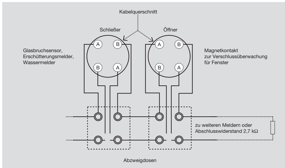
Bild 20: Prinzipieller Anschluss von 4adrigen Sensoren in einer Meldergruppe mit Abschlusswiderstand
