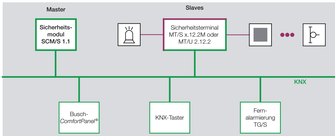
Bild 10: Prinzipieller Aufbau einer Überwachungsanlage mit einem Sicherheitsmodul
