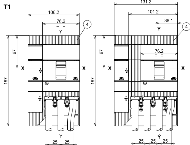
前接线端子 - F
