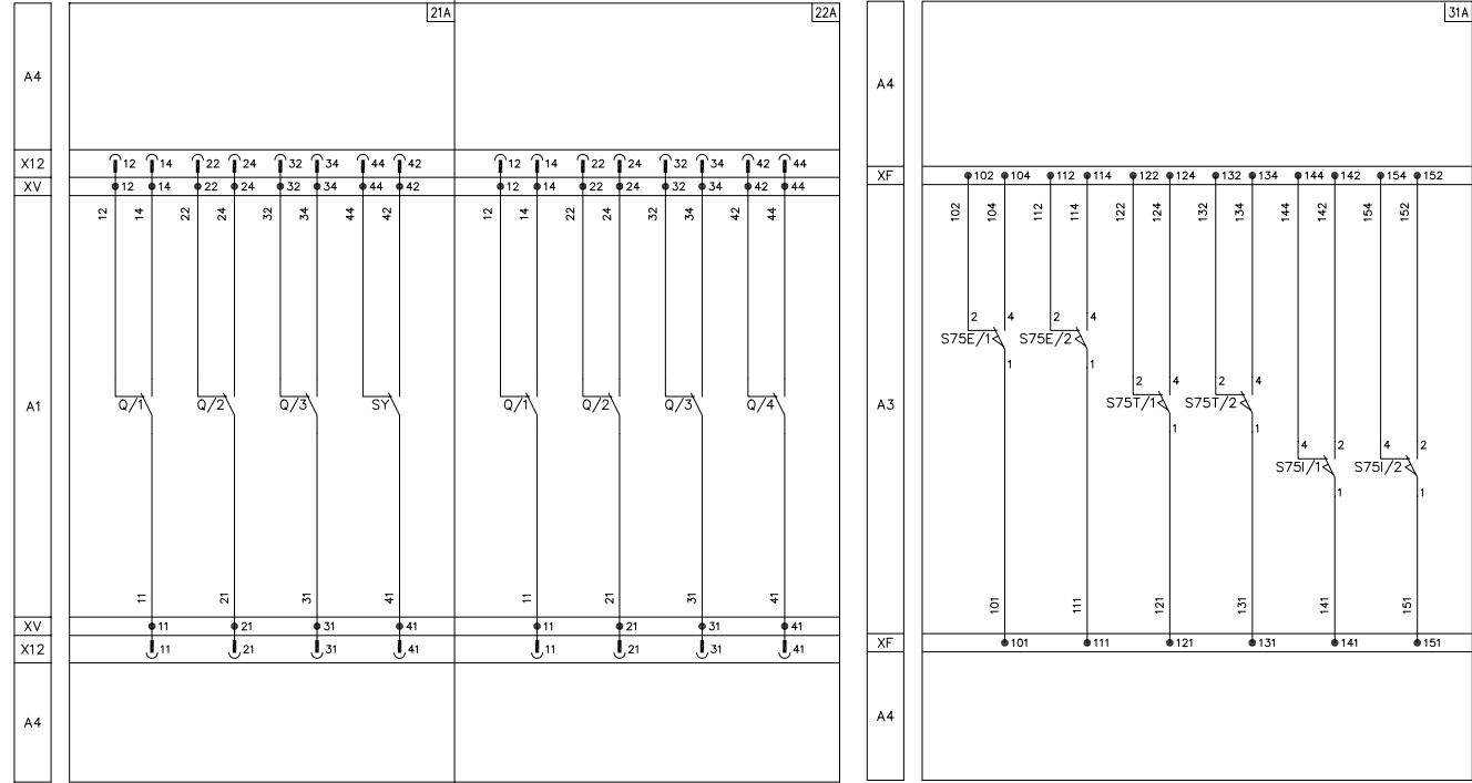
信号触头
