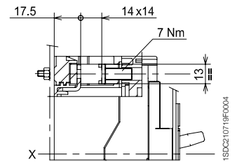
铜 / 铝电缆前接线端子 - FC CuAl 95mm 2
