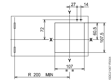
不带法兰
