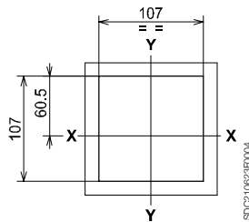
不带法兰
