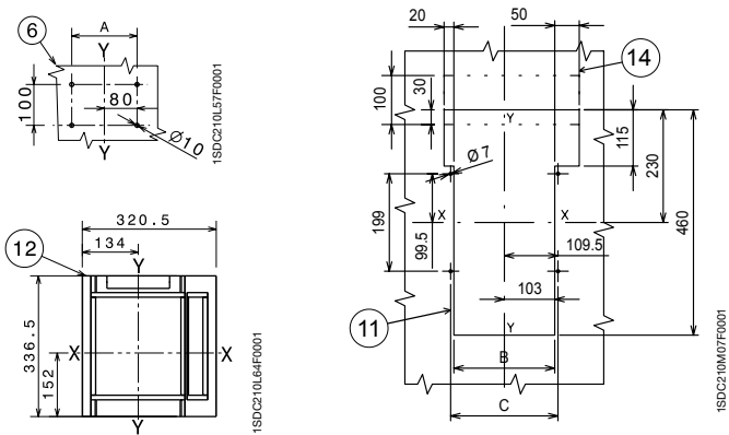
支撑钢板钻孔图
