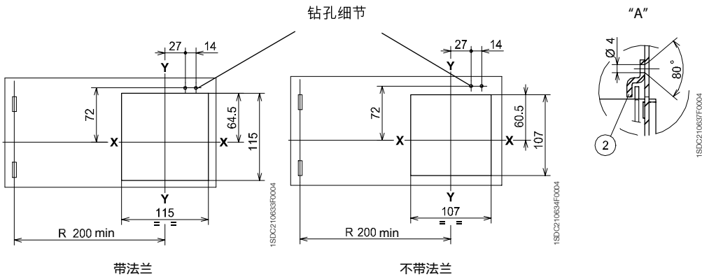
小室门钻孔图
