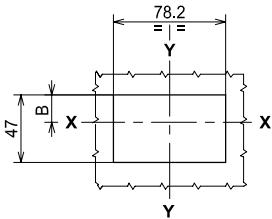
不带法兰 操作机构扩展
