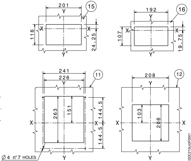
小室门钻孔图
