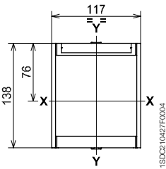
小室门法兰
