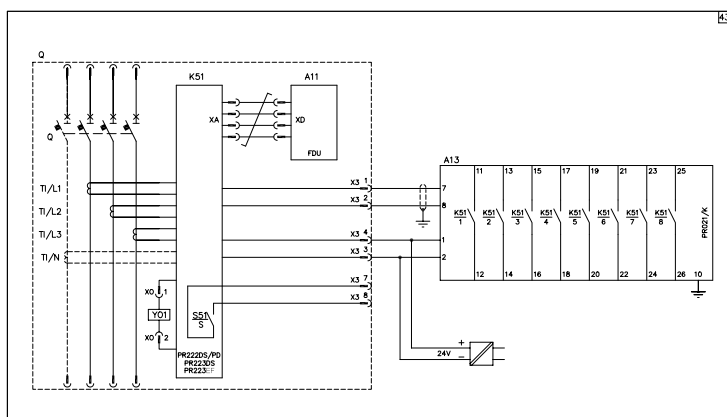
PR222DS/PD、PR223DS或PR223EF电子脱扣器与FPU前面板显示单元及PR021/K信号单元的连接
