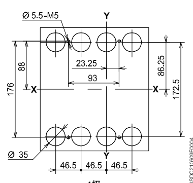
4极
