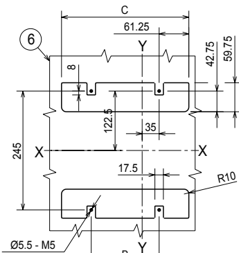
支撑钢板钻孔图
