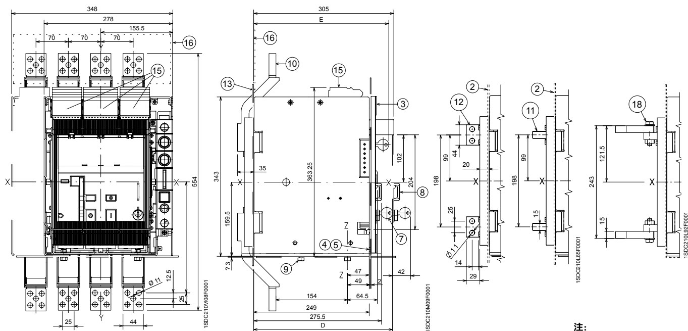
后垂直接线端子 - VR
