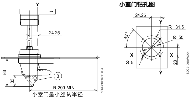
小室门钻孔图
