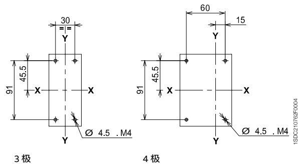
前接线端子 - F
