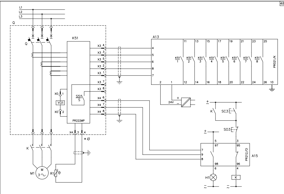
PR222MP电子脱扣器与PR021/K信号单元和PR212/CI 接触器控制单元的连接
