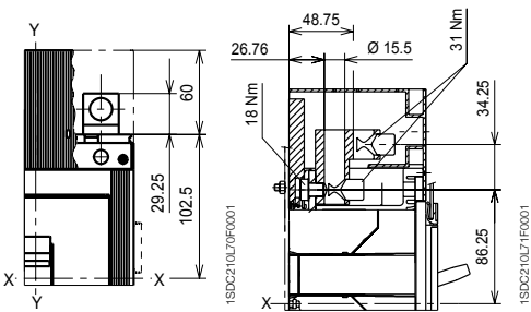
铜 / 铝电缆前接线端子 - FC CuAl 2x120mm 2
