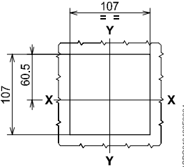
不带法兰
