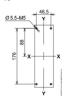
3 极
