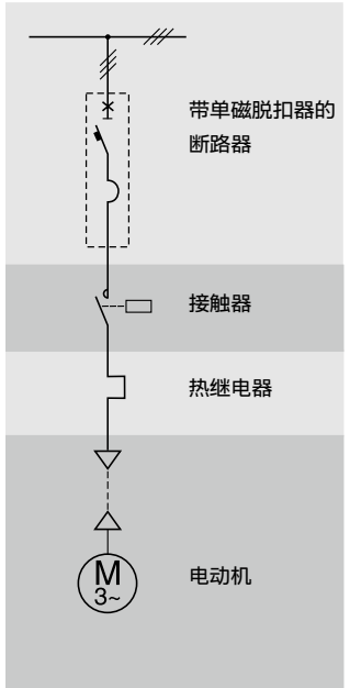
短路保护
