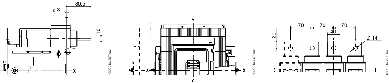
3-4 极
