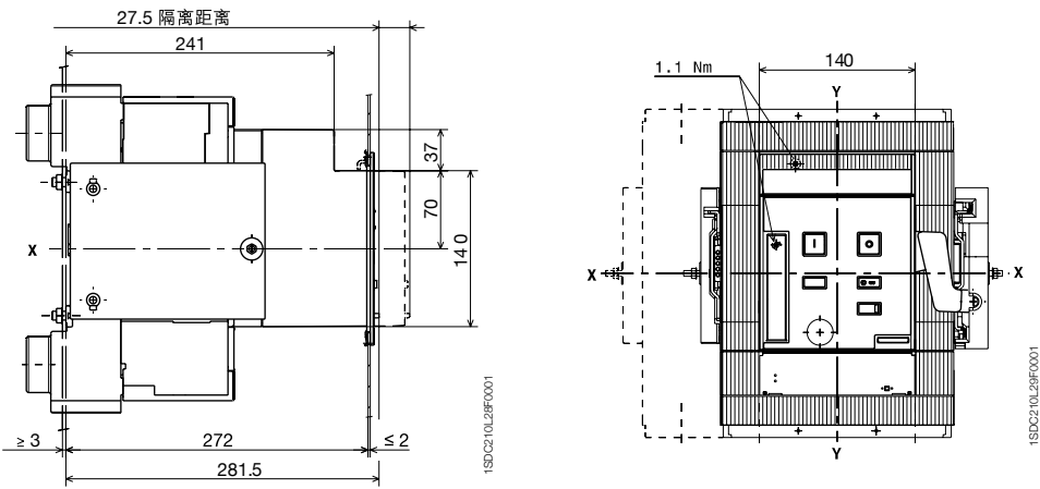
电动操作机构
