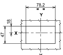
不带法兰和断路器 与小室门平齐（3-4极） 或扩展（3极）
