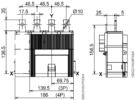
加长前接线端子 - EF 630 A
