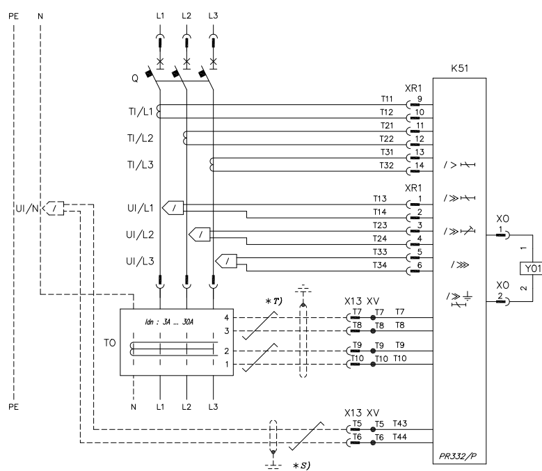
带PR332/P电子脱扣器和剩余电流保护的3极断路器 ( U \leq 690V )
