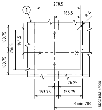
小室门钻孔图
