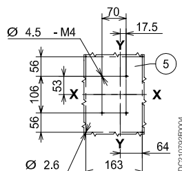
4 极
