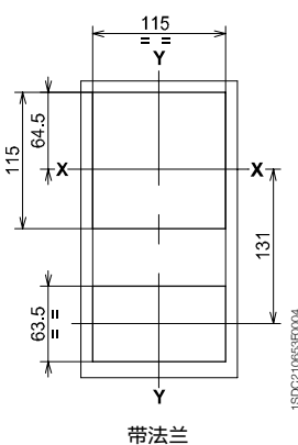
带法兰
