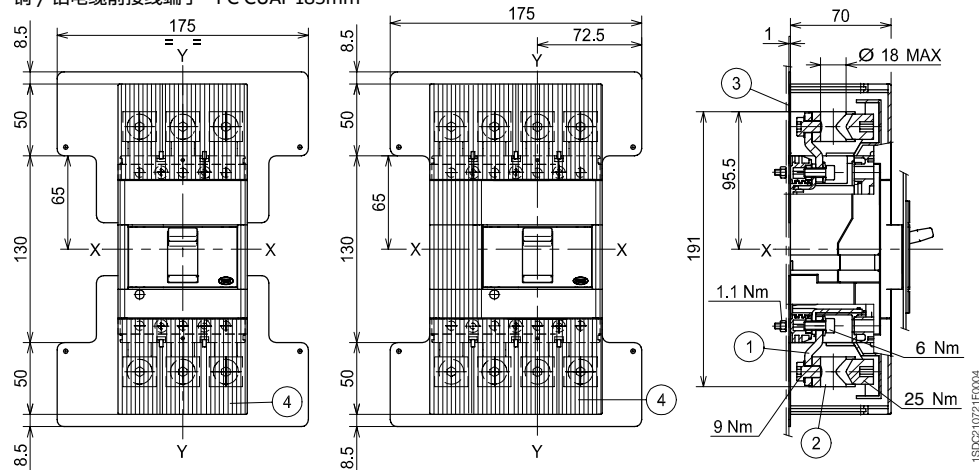
铜 / 铝电缆前接线端子 - FC CuAl 185mm 2
