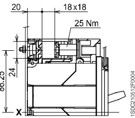
铜电缆前接线端子 - FC Cu
