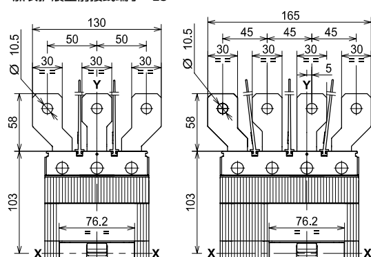
加长扩展型前接线端子 - ES
