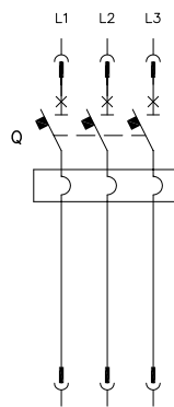
带磁脱扣器的3极断路器
