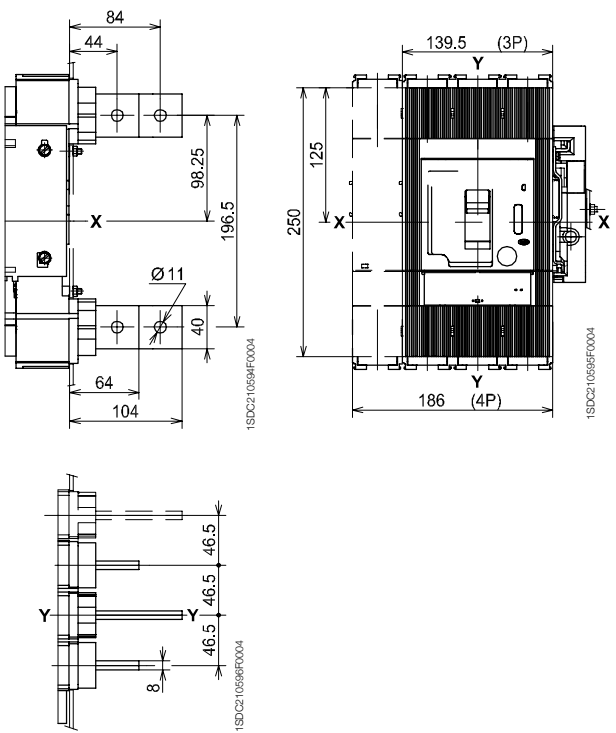
后垂直接线端子 - VR 630 A
