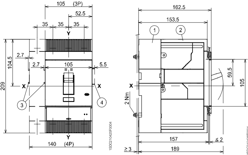
安装在钢板上
