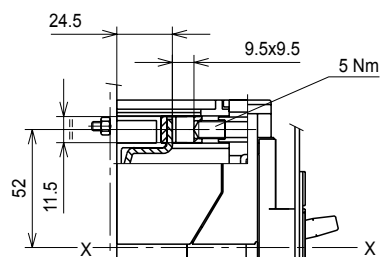
铜/铝电缆前接线端子 - FC CuAl 50mm 2
