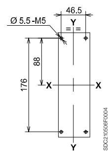
3极
