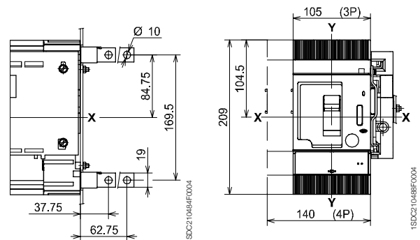
后垂直接线端子 - VR
