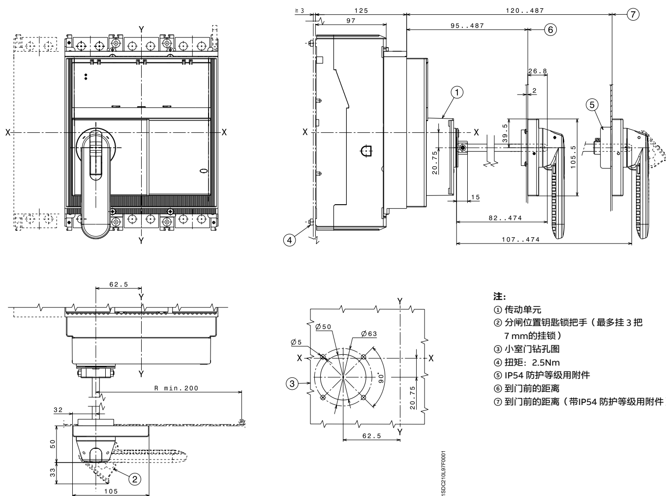
小室门上的旋转手柄操作机构
