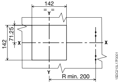
不带法兰
