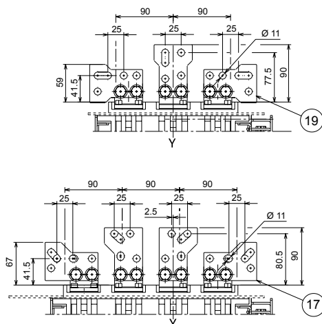
后扩展接线端子 - RS
