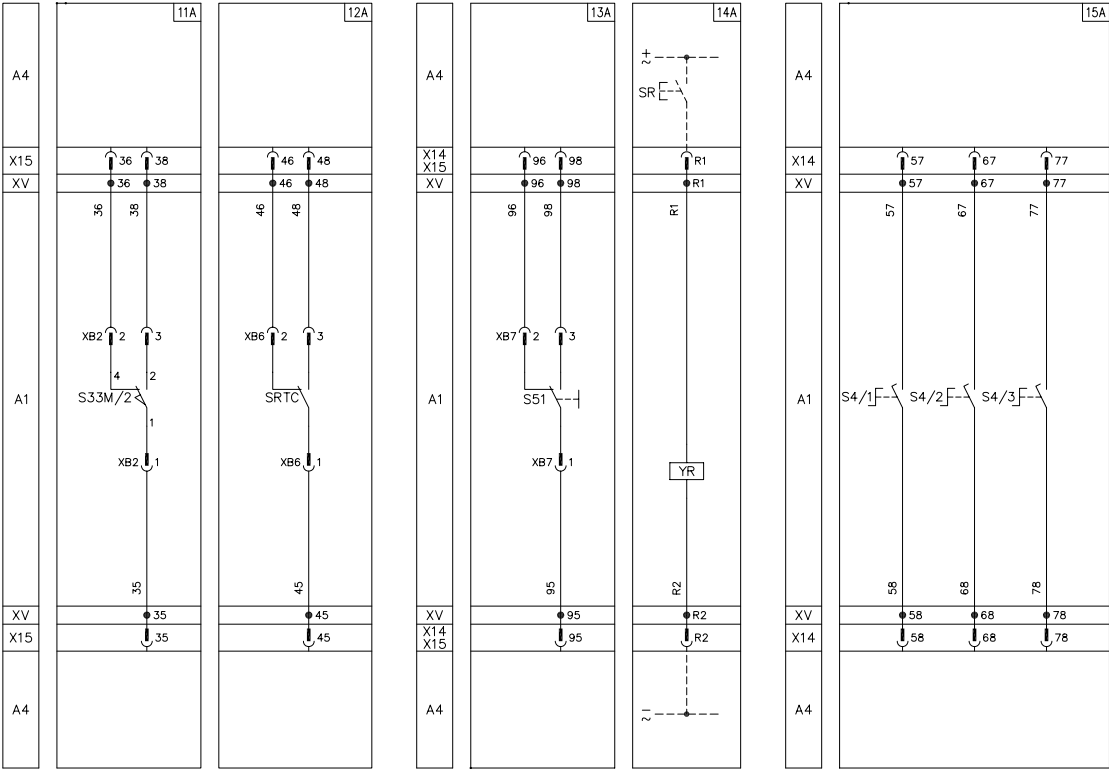
信号触头
