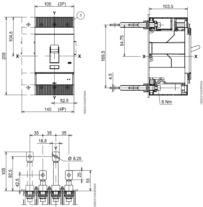
后接线端子 - R
