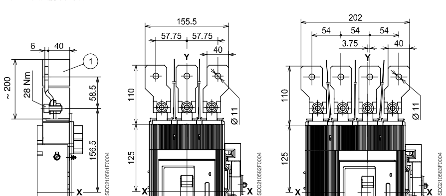
加长扩展前接线端子 - ES 630 A
