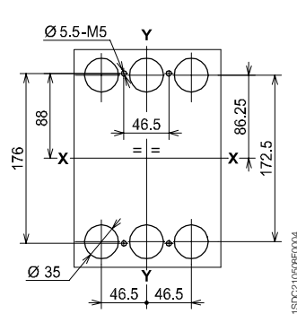
3极
