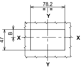
不带法兰 操作机构与 小室门平齐
