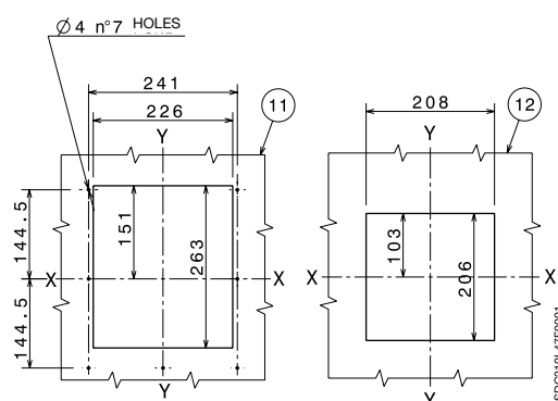
小室门钻孔图
