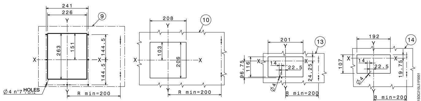
小室门钻孔图
