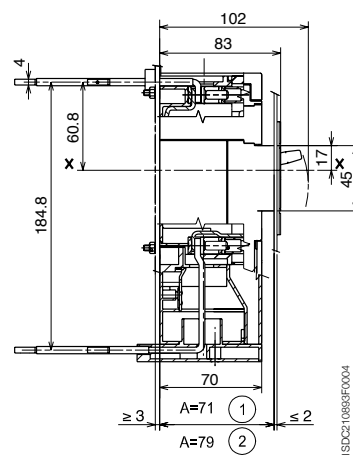
后水平接线端子 - HR
