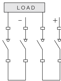
不接地电网的接线图
