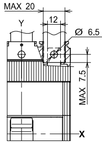
前接线端子 - F
