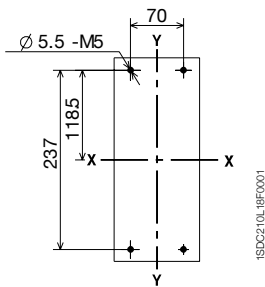
3 极
