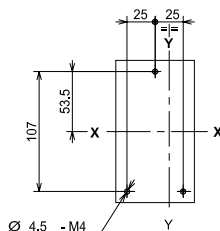
4极
