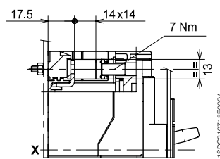
铜 / 铝电缆前接线端子 - FC CuAl 185mm 2
