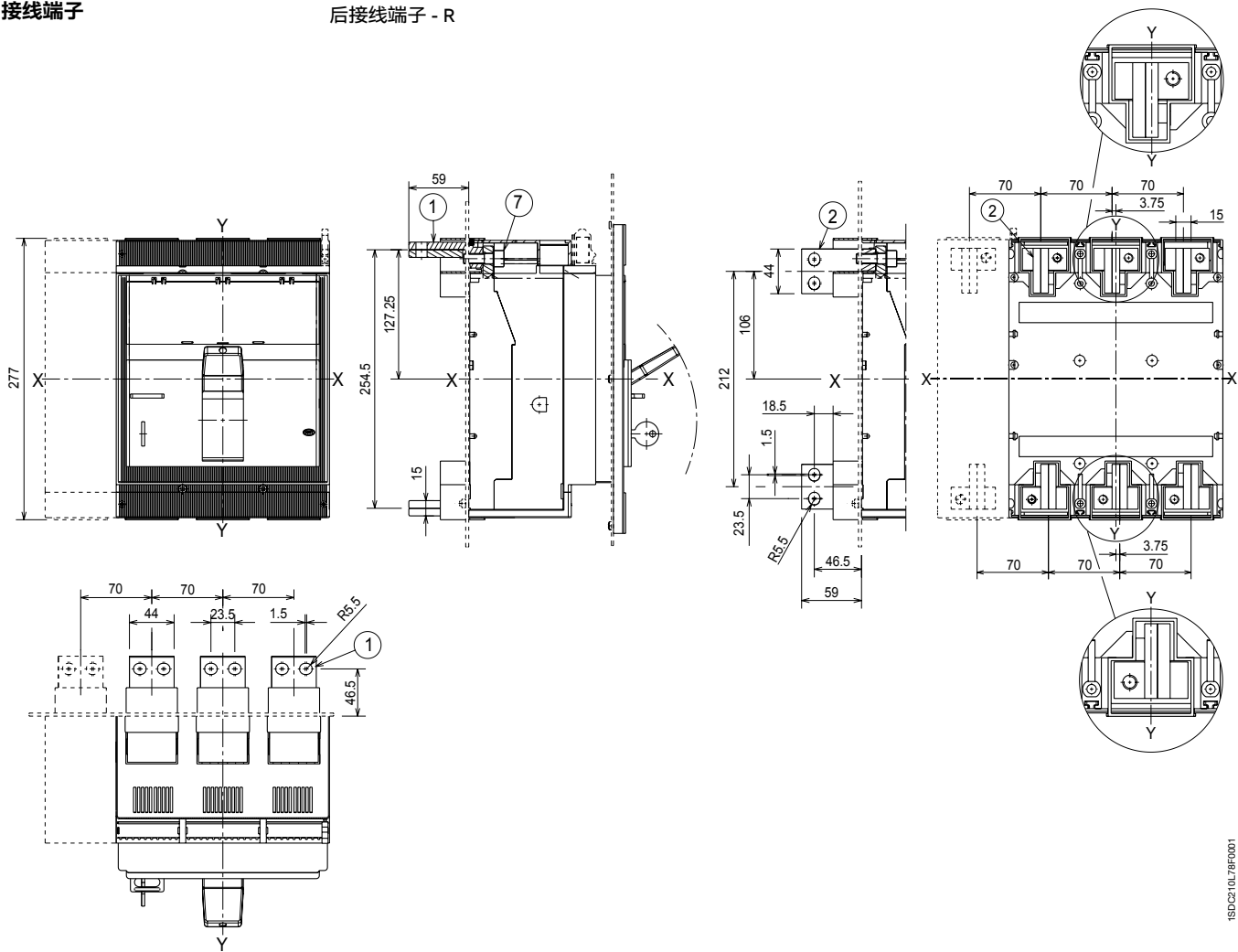
接线端子
