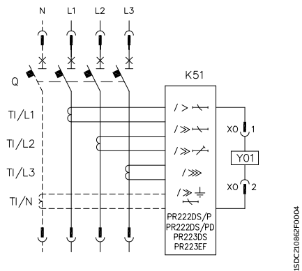
带PR222DS/P、PR222DS/PD、PR223DS或PR223EF电子脱扣器的3/4极断路器
