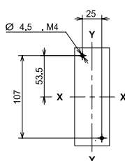
3极
