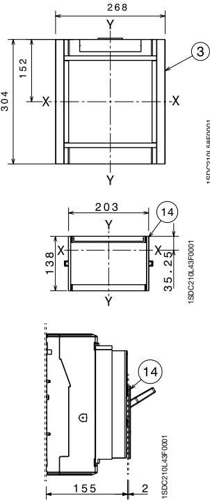
小室门法兰 (标配)
