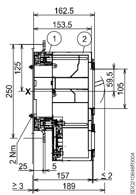
前接线端子 - F 安装在钢板上
