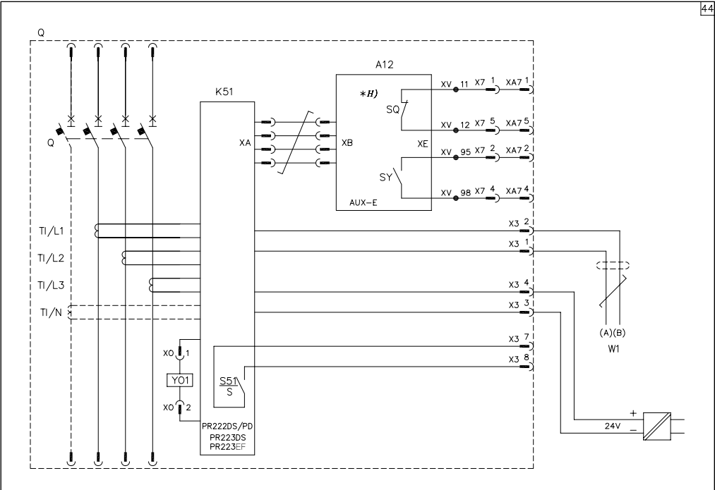
PR222DS/PD和PR223DS或PR223EF电子脱扣器与AUX-E辅助触头的连接
