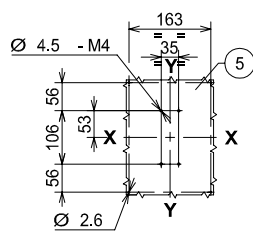
3 极
