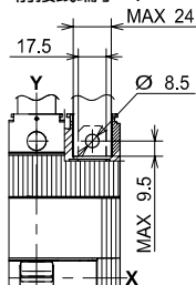
前接线端子 - F
