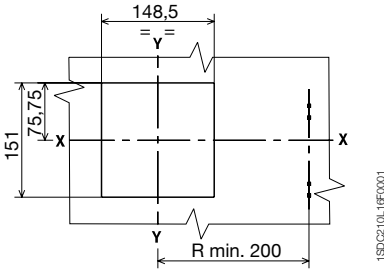
带法兰
