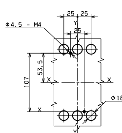
3极
