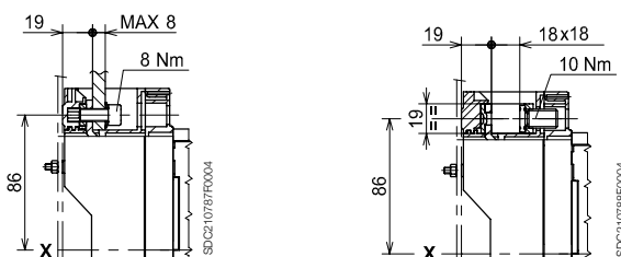
铜 / 铝电缆前接线端子 - FC CuAl 240mm 2
