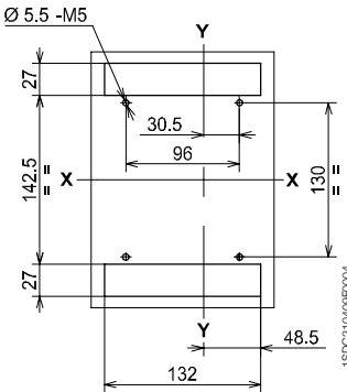
4 极
