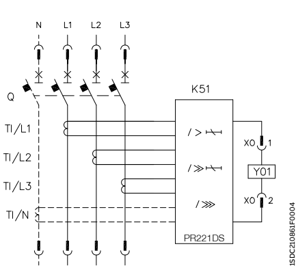
带PR221DS电子脱扣器的3/4极断路器
