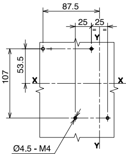
支撑钢板钻孔图
