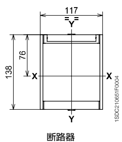
断路器
