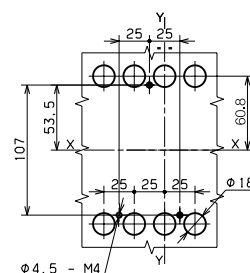
4极
