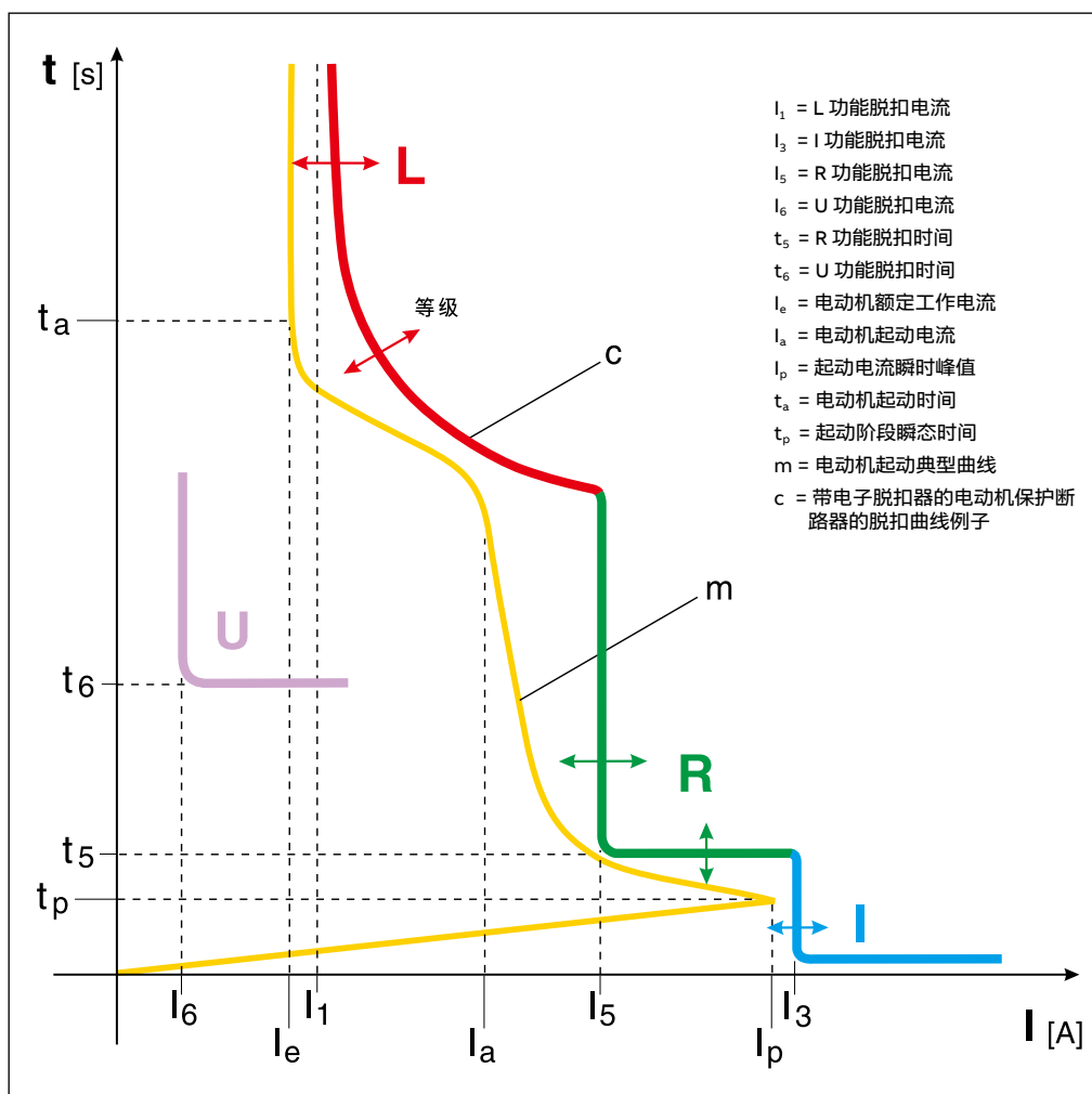
异步电动机运行特性曲线
