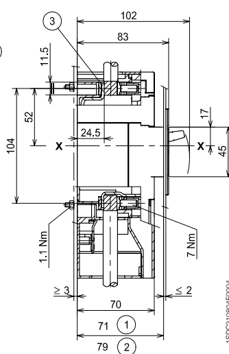
安装在钢板上
