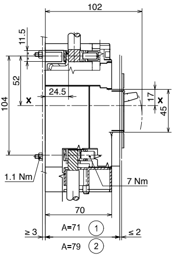
安装在钢板上
