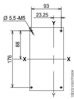
4极
