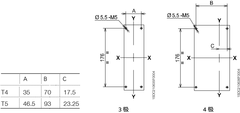
支撑钢板钻孔图
