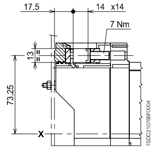
铜 / 铝电缆前接线端子 - FC CuAl 95mm 2
