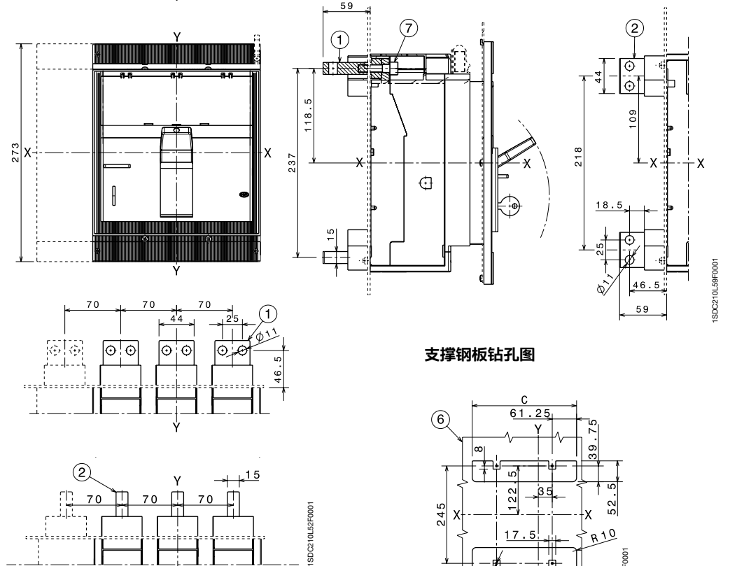
后水平或垂直接线端子 - HR/VR
