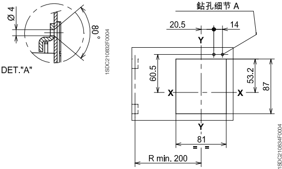
小室门钻孔图
