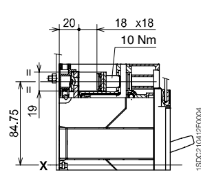
铜电缆前接线端子 - FC Cu
