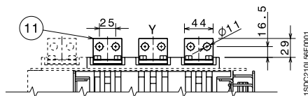
后水平接线端子 - HR
