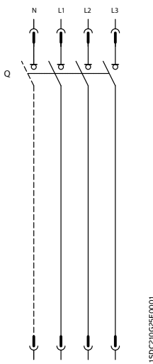
3/4隔离开关
