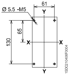
3 极
