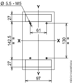
3 极
