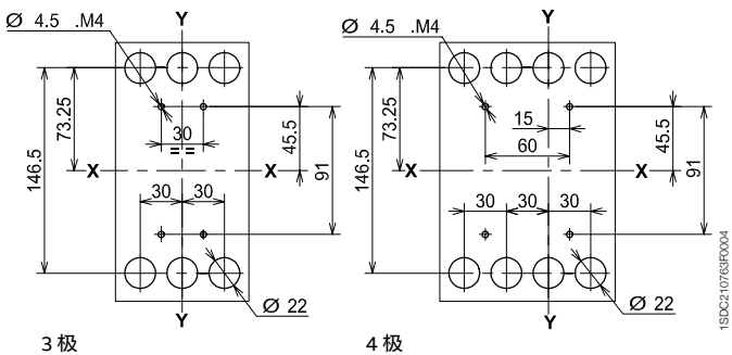
后接线端子 - R
