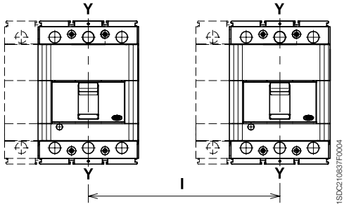
2 个并排断路器或叠装断路器之间的最小中心间距 对于并排安装断路器或叠装断路器, 检查连接母排或电缆, 确保空气绝缘距离不会减少
