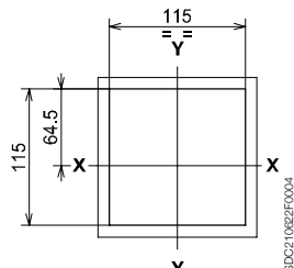
带法兰
