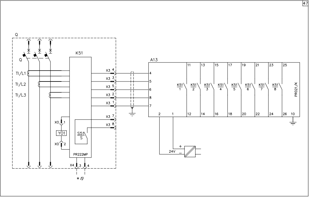
PR222MP电子脱扣器与PR021/K信号单元的连接
