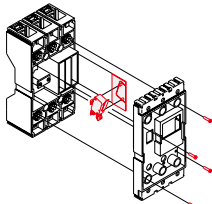
T2-T3
