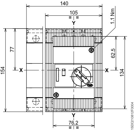
T3
