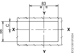
带法兰 操作机构与 小室门平齐
