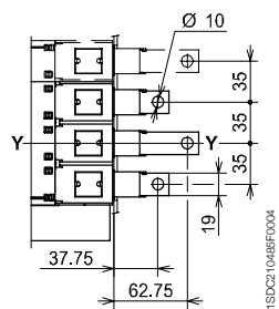
3-4 极
