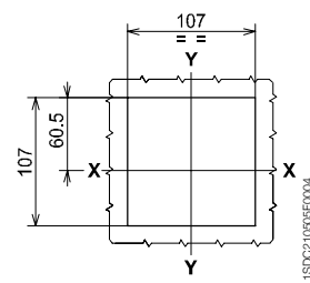
3-4 极 (不带法兰)
