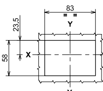
带法兰和断路器 与小室门平齐 (3-4极)
