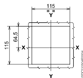
3-4 极 (带法兰)
