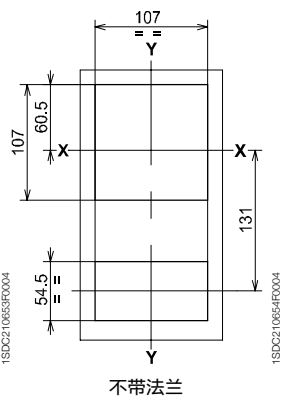
不带法兰
