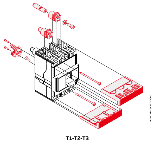
T1-T2-T3
