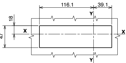
小室门钻孔图
