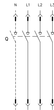
3/4极隔离开关
