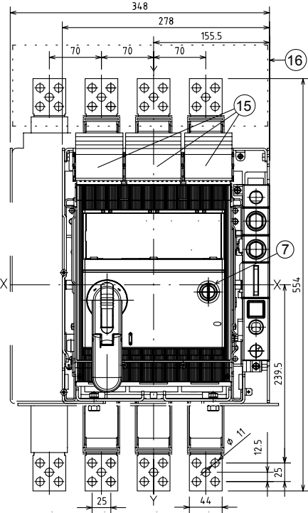
断路器上的旋转手柄操作机构
