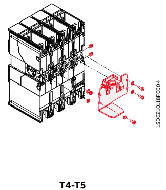
T4-T5
