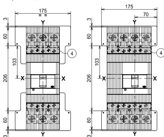
铜 / 铝电缆前接线端子 - FC CuAl 240mm 2
