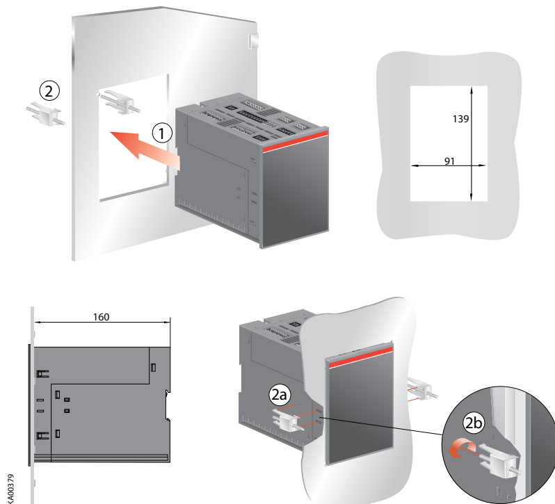
Рисунок 8.1: Установка на дверь ATS022
