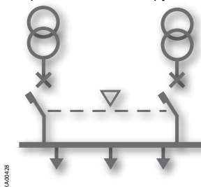
Рисунок 4.1: Схема применения 2CBs (2 Выключателя) – Генератор не используется
