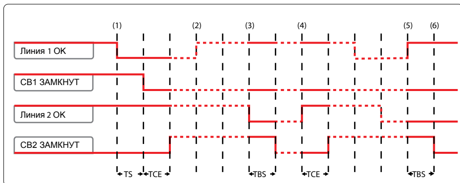
Рисунок 4.14: Временная диаграмма 2CBs (2 выключателя) - генератор не используется – без процедуры автовозврата
