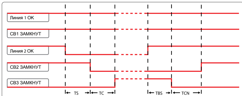
Рисунок 4.13: Временная диаграмма 3CBs BUS TIE (3 Выключателя. 2 ввода и секционный выключ.) – сбой линии LN2
