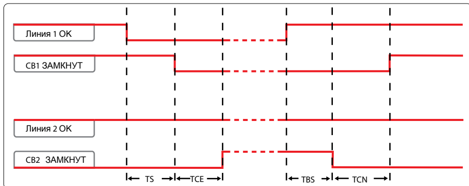
Рисунок 4.2: Временная диаграмма применения 2CBs (2 выключ.) - основная линия LN1
