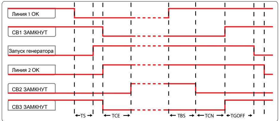
Рисунок 4.9: Временная диаграмма 3СВs NPL (СВ3 в линии неприор. нагр) - генератор используется
