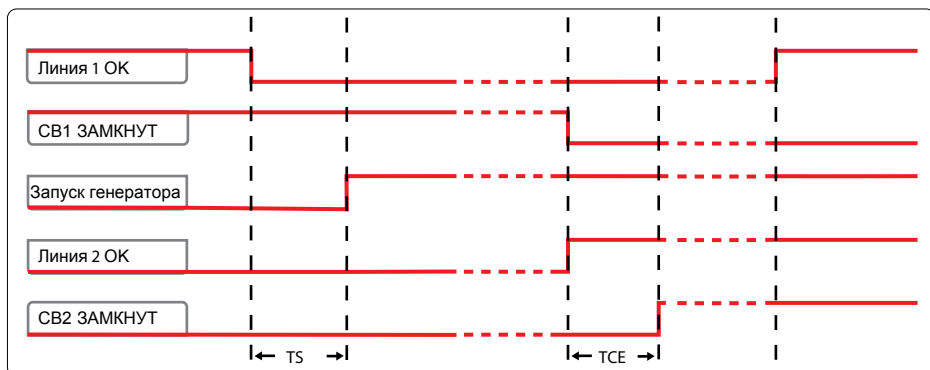
Рисунок 4.17: Временная диаграмма без приоритета линии питания – генератор используется
