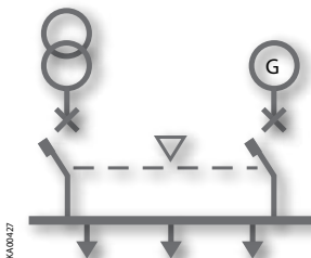
Рисунок 4.3: Схема применения 2CBs (2 Выключателя) – генератор используется
