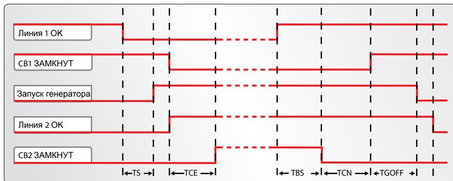
Рисунок 4.4: Временная диаграмма 2CBs (2 выключ.) - основная линия LN1
