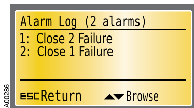
Рисунок 5.7: Диагностика – Страница журнала аварий ATS022
