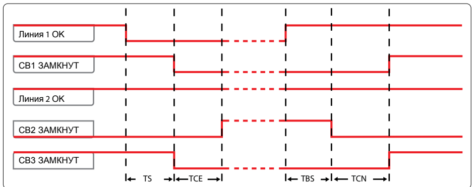
Рисунок 4.10: Временная диаграмма 3СВs NPL (СВ3 в линии неприор. нагр) - генератор не используется - основная линия LN1
