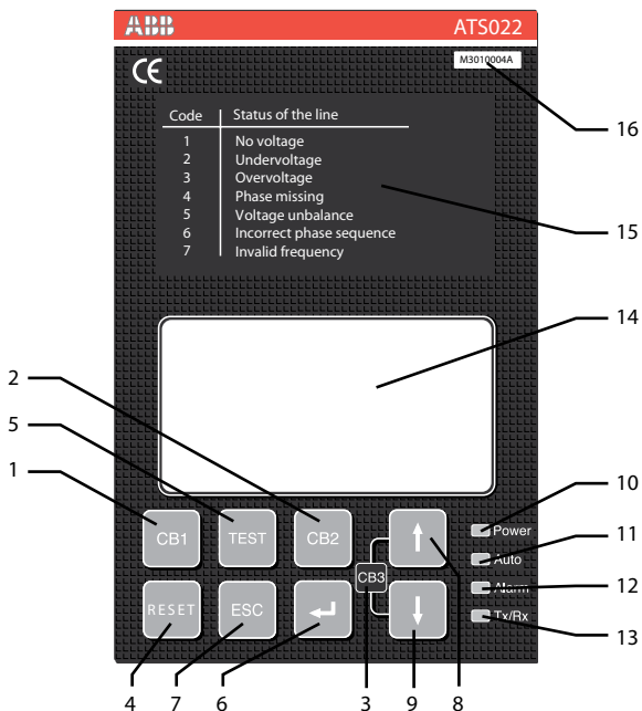
Рисунок 5.1: Описание интерфейса передней панели ATS022
