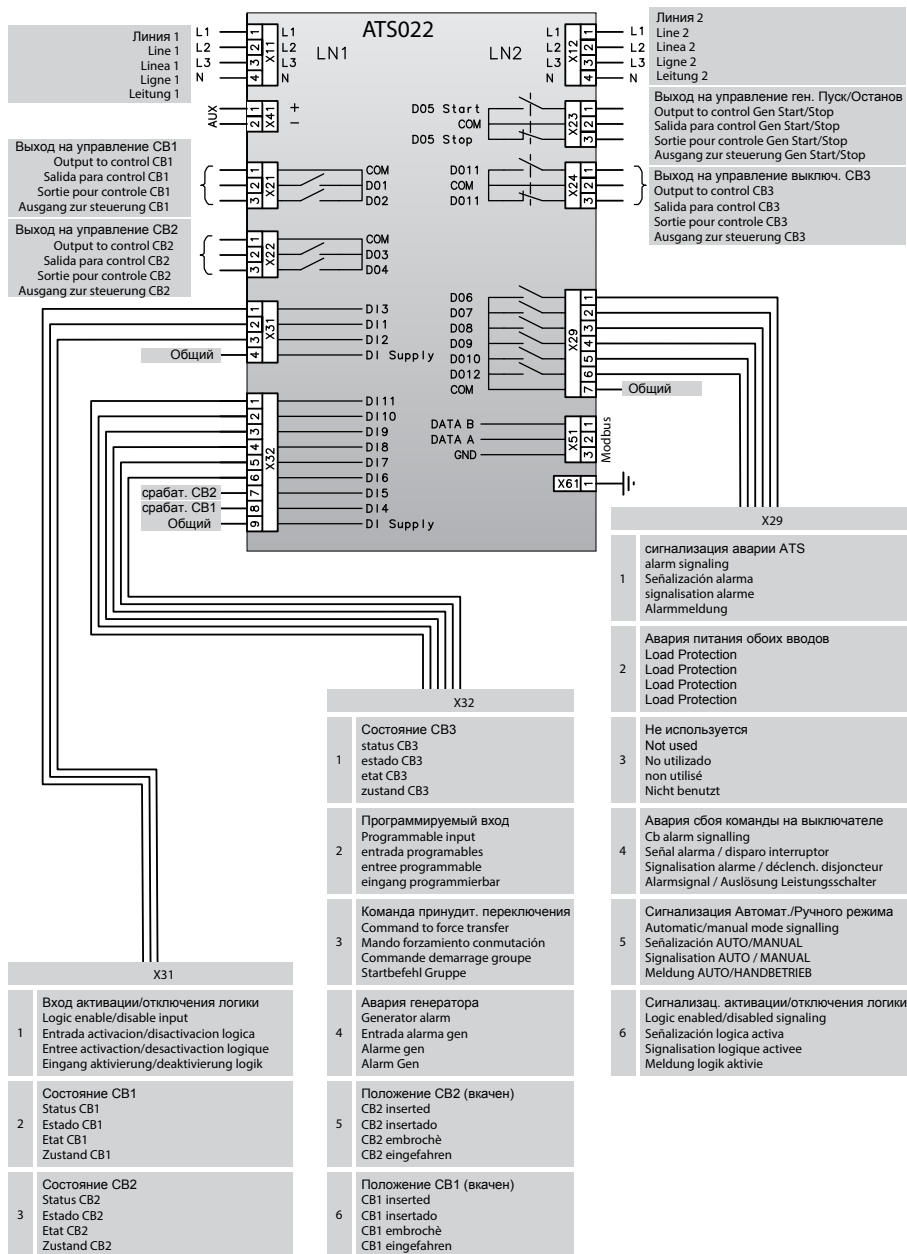
Рисунок 6.1: Схема цепей управления блока ATS022
