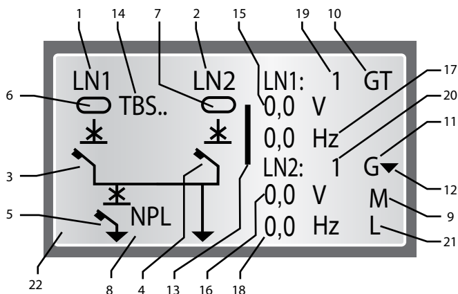
Рисунок 5.4: Описание дисплея ATS022
