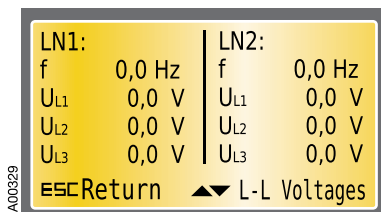
Рисунок 5.6: диагностика – страница измеренных значений ATS022
