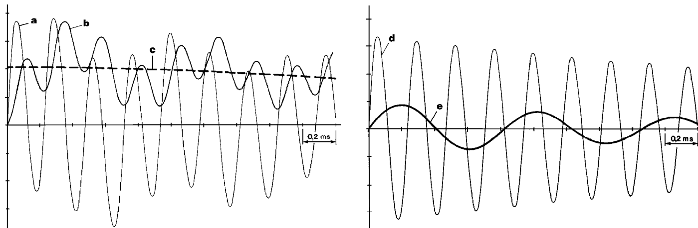
投切后初始 2ms 的电流、电压波形
