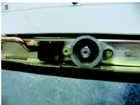
5 门闭锁装置 | 6 手车闭锁磁铁 | 7 不同额定电流的闭锁防护 | 8 电机驱动车手车
