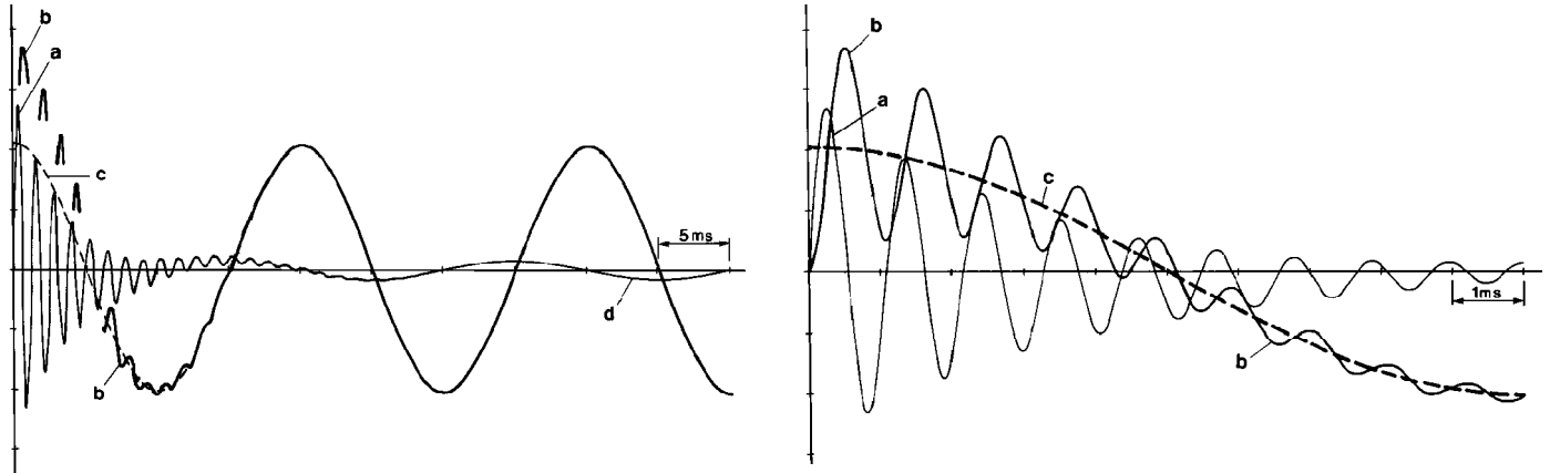
投切瞬时及投切后的电流、电压波形
