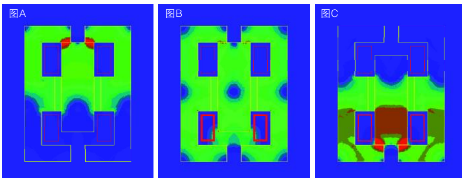
图A 合闸位置的磁场分布 | 图B 分闸线圈带电时的磁场分布 | 图C 分闸位置的磁场分布
