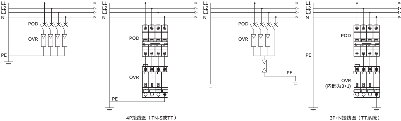
POD+电涌保护器接线图
