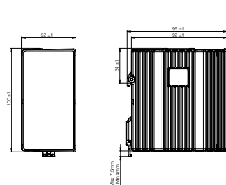
NE801
