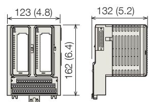
Redundant I/O
