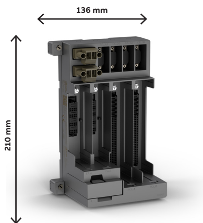
TU865 Ethernet FCI MTU
