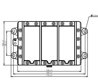
NE820
