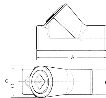
EYS1 – EYS5
