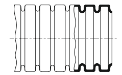
Grobprofil G Hohe Ausreisskräfte
