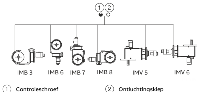
Afbeelding 3: Toegestane installatieposities
