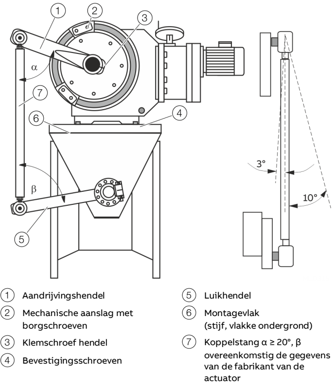
Afbeelding 4: Onderdelen voor hefboomaandrijving
