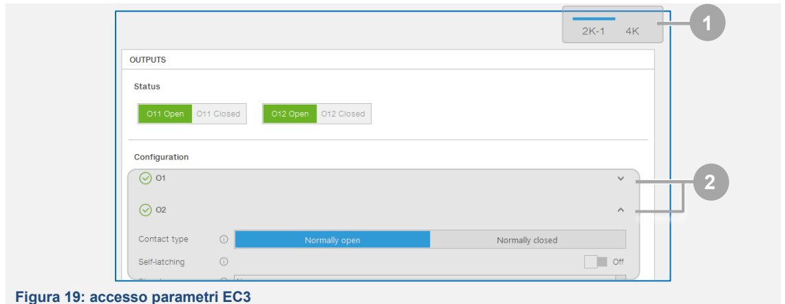
Figura 19: accesso parametri EC3
