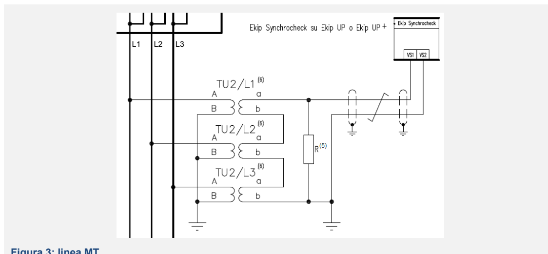
Figura 3: linea MT
