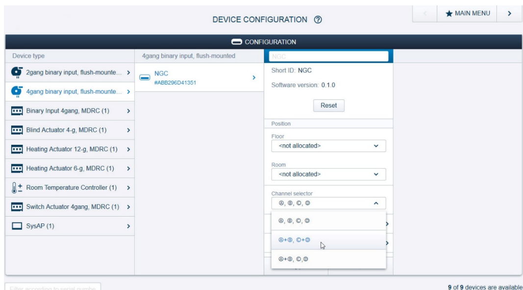
Fig. 1: Acoplamiento de dos canales para la conexión de un pulsador doble
