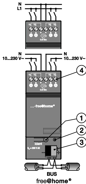
Fig. 5: Vista general de la entrada binaria de 4 canales para carril DIN
