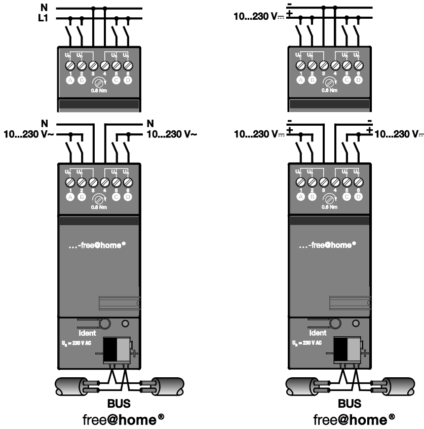
Fig 11: Conexión eléctrica BI-M-4.0.1
