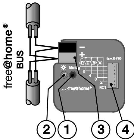
Fig. 4: Vista general de la entrada binaria de 4 canales empotrada
