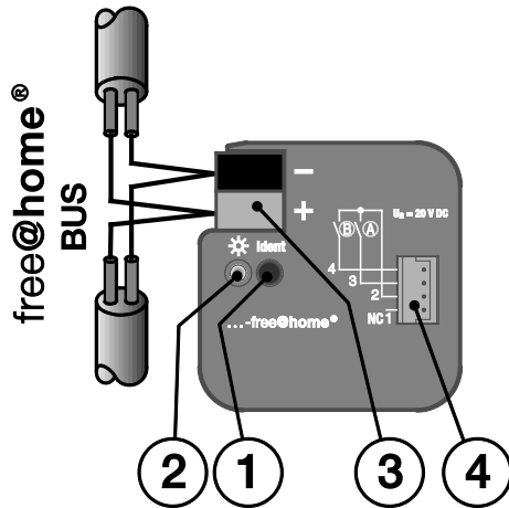
Fig. 3: Vista general de la entrada binaria de 2 canales empotrada
