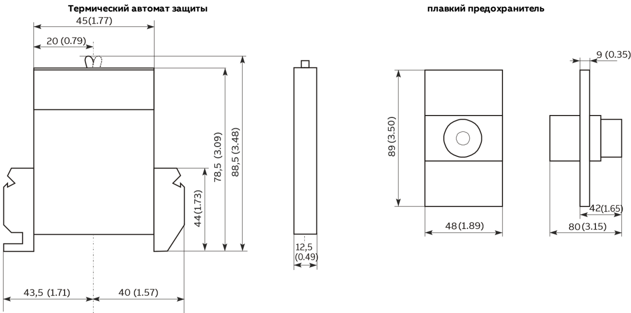
Рисунок 3. Габаритные размеры в мм (in)
