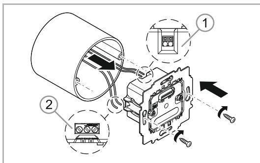
Abb. 7: Anschluss und Einbau
