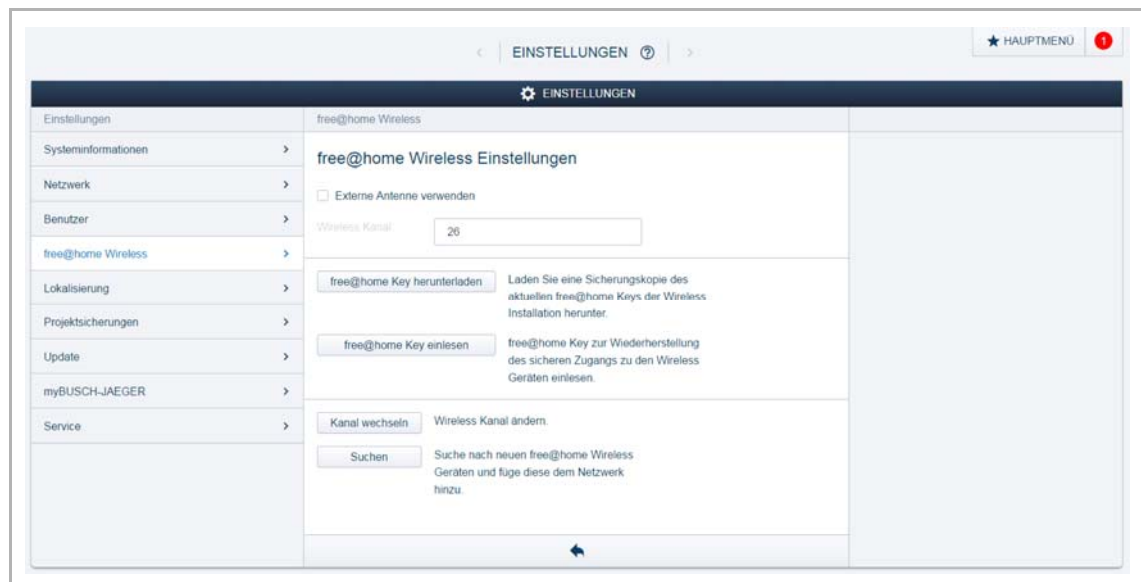
Abb. 11: Kopplung Wireless-Geräte mit System Access Point
