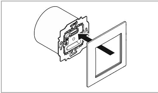
Abb. 9: Montage Rahmen
