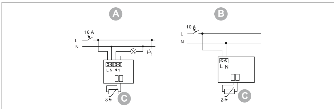
Abb. 5: Elektrischer Anschluss
