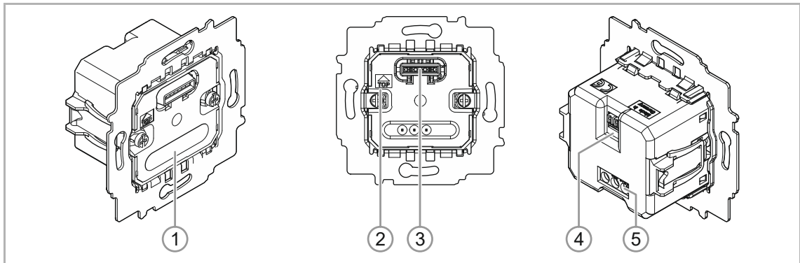
Abb. 2: Geräteübersicht Raumtemperaturregler
