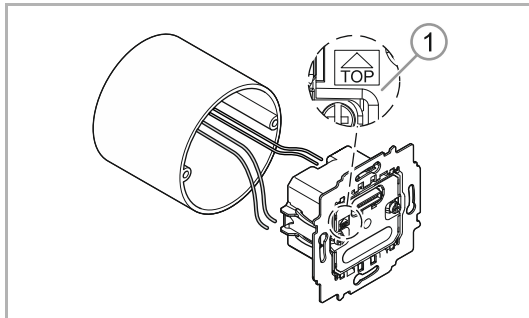
Abb. 6: Einbauposition
