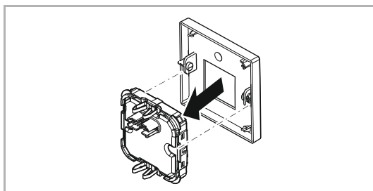
Abb. 8: Montage Abdeckung
