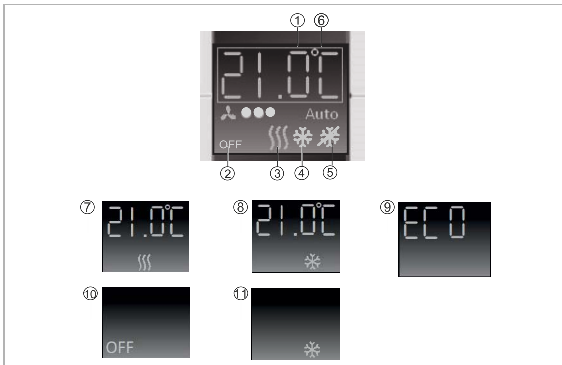
Abb. 21: Displayanzeigen
