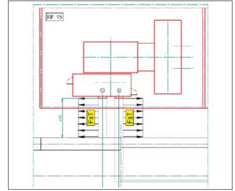
Fig 6 Rectifier bus bar force calculation
