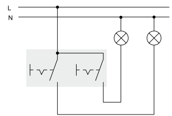
Διακόπτης κομιατέρ
