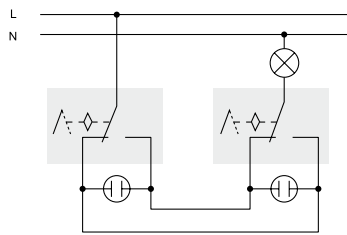
Διακόπτης αλέ-ρετούρ
